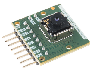
FIGURE 4.13 : Le module de capture FLIR
