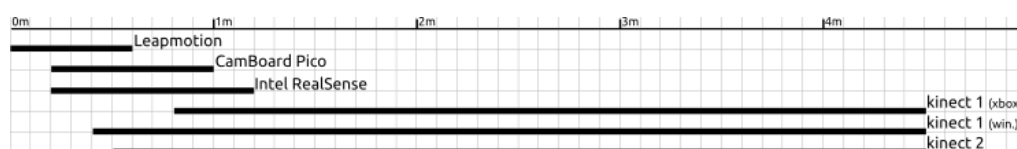
FIGURE 4.14 : Les zones de captures de chacun des périphériques offrant une sortie 3D
