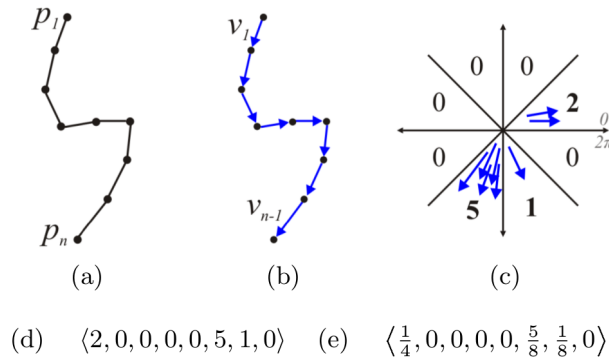
FIGURE 5.6 : Les étapes de traitement d'un tracé pour créer un tableau d'indices normalisés
