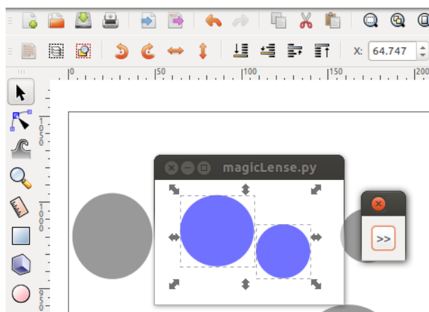
FIGURE A.3 : Implémentation du concept des "magic lenses". L'application complètement séparés a une fenêtre semi-transparente et peut modifier la couleur des éléments qui se situent derrière son cadre dans Inkscape
