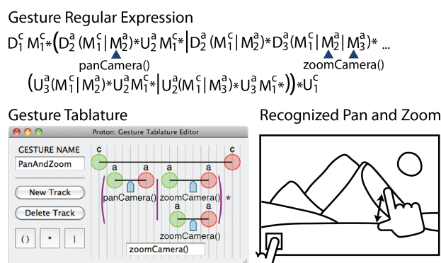
FIGURE 5.11 : Le moteur de création et de détection des gestes en les considérant comme des expression régulières Proton
