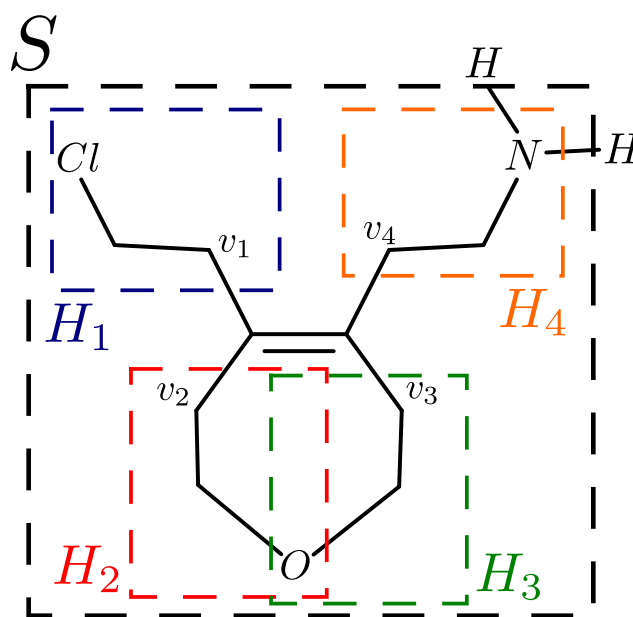
FIGURE 4.5 – Exemple d’un stéréo sous-graphe minimal S divisé en sous-graphes associés aux sommets de \text{StereoStar}^*(s) .
