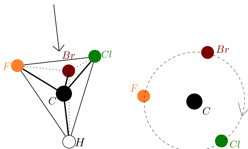
FIGURE 1.10 – Détermination de la nature R ou S du carbone asymétrique du (R)-bromochlorofluorométhane. On observe par la flèche, dans la direction du voisin de plus petite priorité, le H. Les sommets restants dans l'ordre de priorité décroissant, Br, Cl et F, sont rencontrés dans le sens horaire, on a donc une configuration R.
