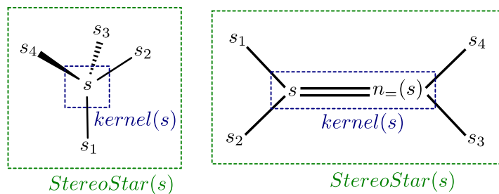
FIGURE 2.7 – Exemple d’ensembles et d’étoiles de stéréo sommets.
