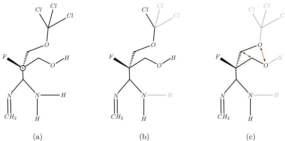
FIGURE 3.1 – Un graphe localement ordonné (a) avec un stéréo sommet \oplus . La suppression de quelques sommets peut ne pas modifier le fait que le sommet soit un stéréo sommet (b), mais la suppression de trop de sommets peut faire perdre à un sommet sa propriété stéréo (c).
