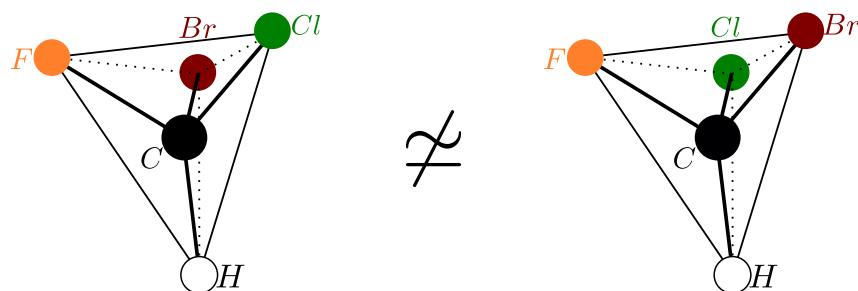
FIGURE 1.4 – Deux stéréoisomères de configuration, le (R)-bromochlorofluorométhane (à gauche) et le (S)-bromochlorofluorométhane (à droite).
