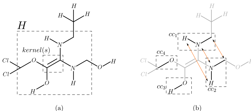
FIGURE 5.1 – On considère un sous-graphe H (a) d'un graphe localement ordonné. Les composantes connexes \{cc_1, cc_2, cc_3, cc_4\} (b) de H sont séparées en deux groupes. Dans ce cas on a \mathcal{I} = \{1, 2\} et \mathcal{J} = \{3, 4\} .
