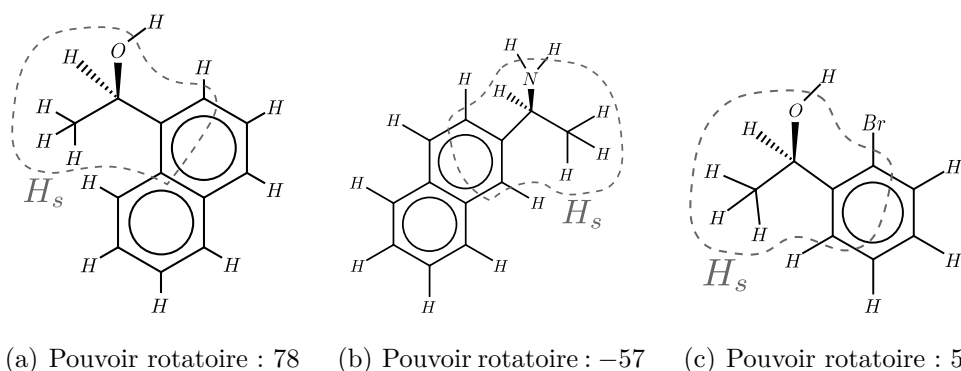
FIGURE 3.5 – Exemples de molécules avec leurs pouvoir rotatoire. Les stéréosous-graphes minimaux H_s sont entourés en gris.
