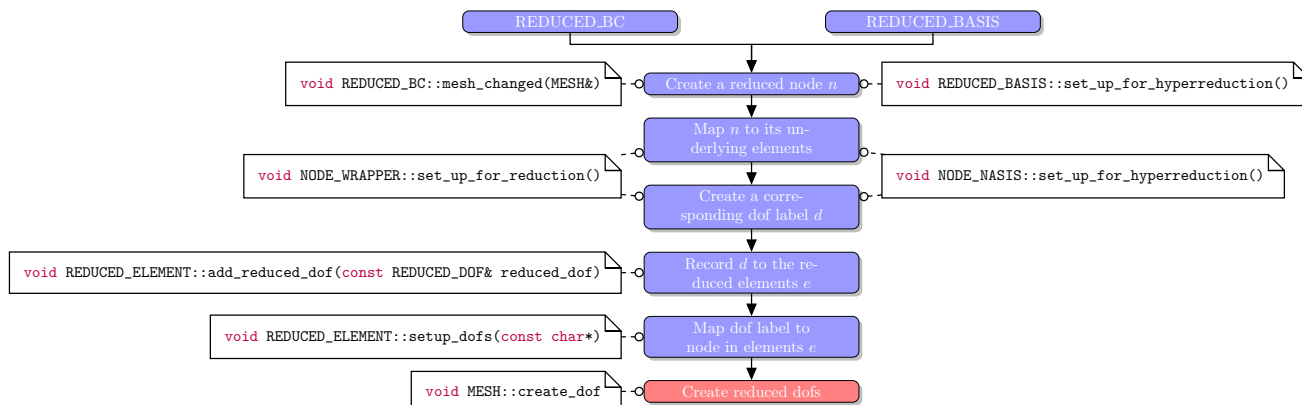
Figure 3.27 – Prise en compte des degrés de liberté réduits
