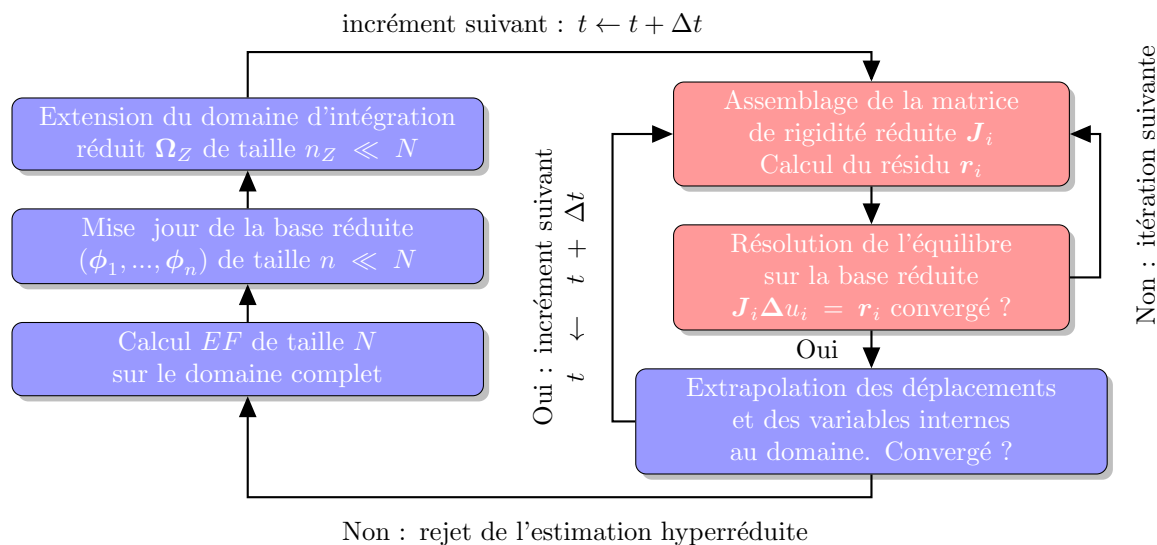
Figure 1.12 – Méthode d'hypperréduction
