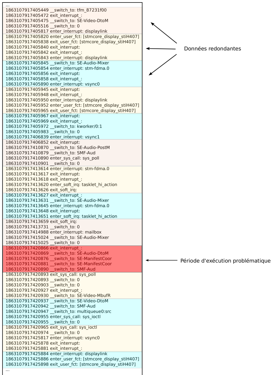
FIGURE 1.2 – Illustration des régimes de fonctionnement répétitifs et problématiques présents dans la trace d'exécution d'une application.
