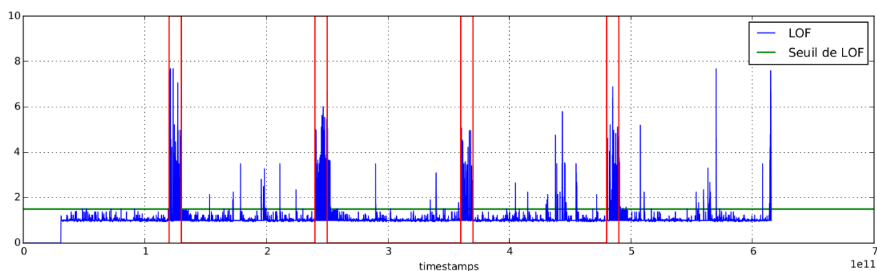
FIGURE 5.11 – Courbe des scores d'anomalies des fenêtres d'événements d'une trace d'exécution
