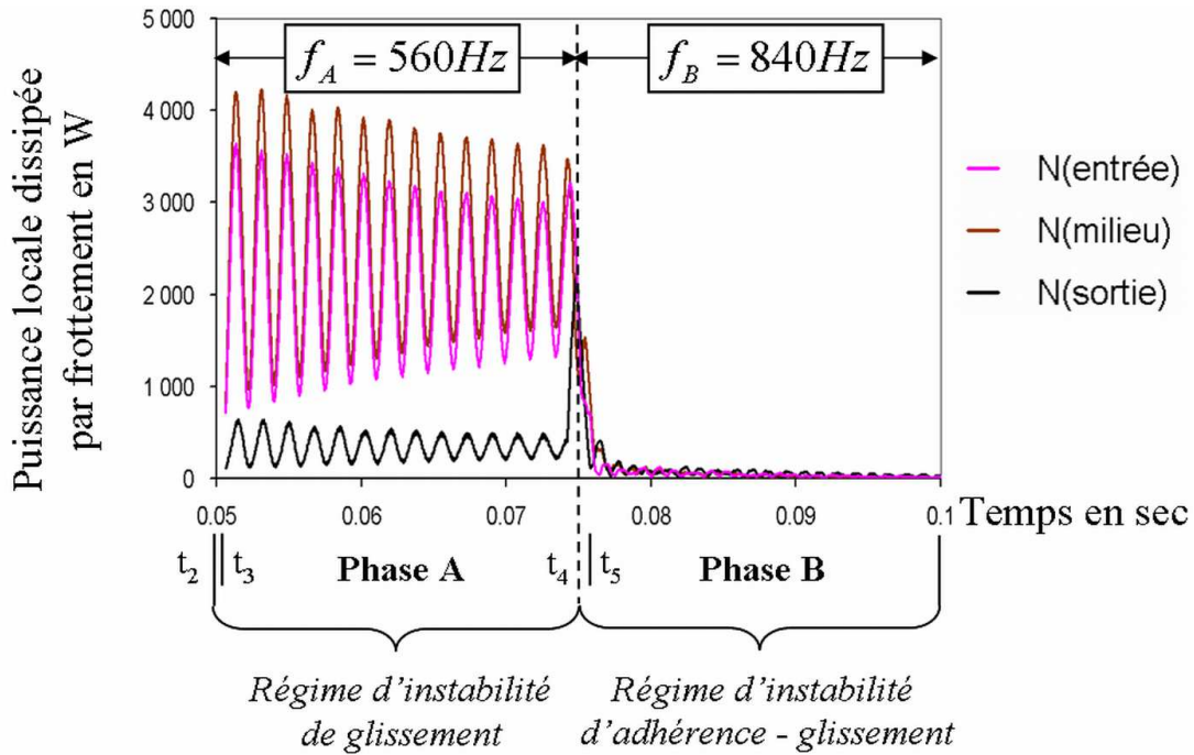
Figure 2–18. Evolution temporelle de la puissance locale dissipée par frottement en N(\text{entrée}) , N(\text{milieu}) et N(\text{sortie})
