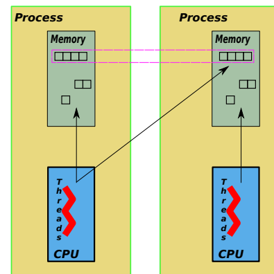
FIGURE 10 – PGAS représentation
