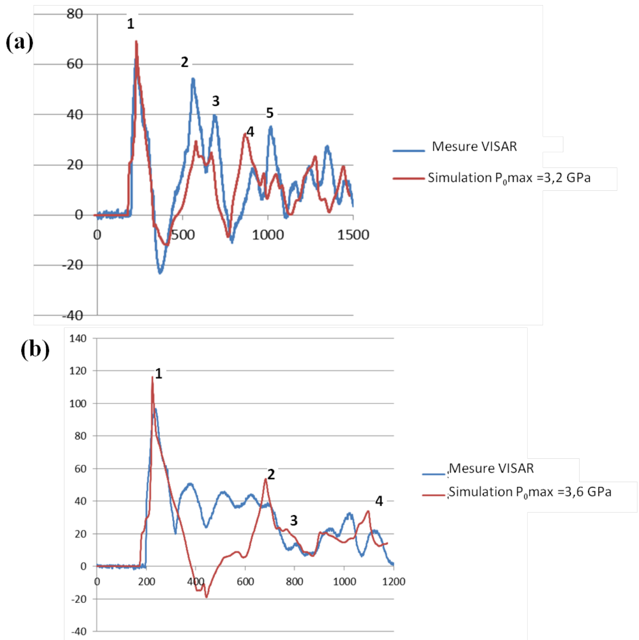
FIGURE IV.29: Profils de vitesse mesurés dans l'assemblage et simulés, (a) avec une densité de puissance laser de 1,8 GW/cm 2 correspondant à une pression maximale appliquée de 2,7 GPa, et (b) avec une densité de puissance laser de 3,9 GW/cm 2 correspondant à une pression maximale appliquée de 4 GPa.
