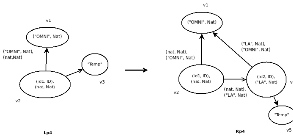
FIGURE 4.13 – Instantiation d’un nœud non terminal en un LA ( p_4 )
