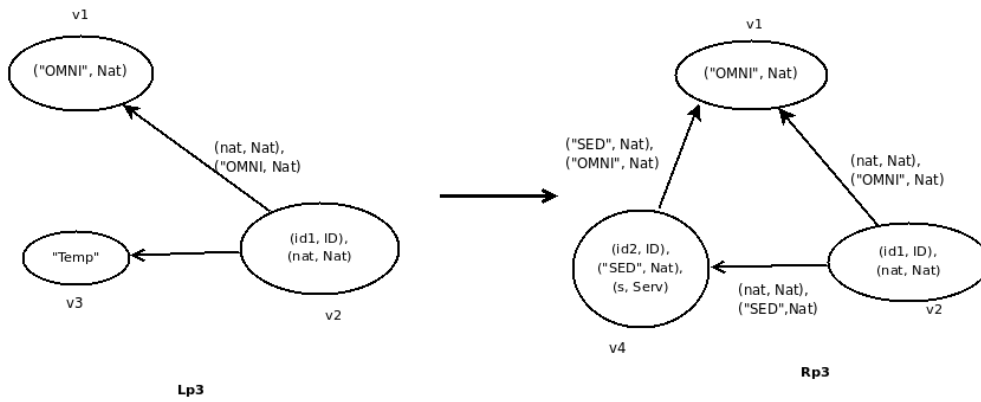
FIGURE 4.12 – Instantiation d’un nœud non terminal en un SED ( p_3 )
