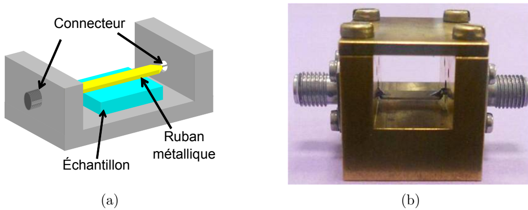
FIGURE 3.3 – a) Schéma 3D et b) photographie de la cellule triplaque. L'échantillon est inséré entre le ruban métallique suspendu et le plan de masse.
