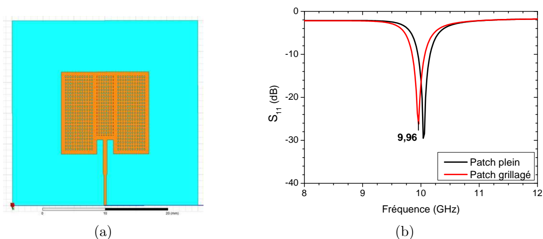
FIGURE 5.17 – a) Design HFSS® vu de dessus de l'antenne patch grillagée inspiré des travaux de S. Cheng [114]. b) Fréquence de résonance simulée sous HFSS® de l'antenne grillagée comparée à l'antenne avec un patch plein.
