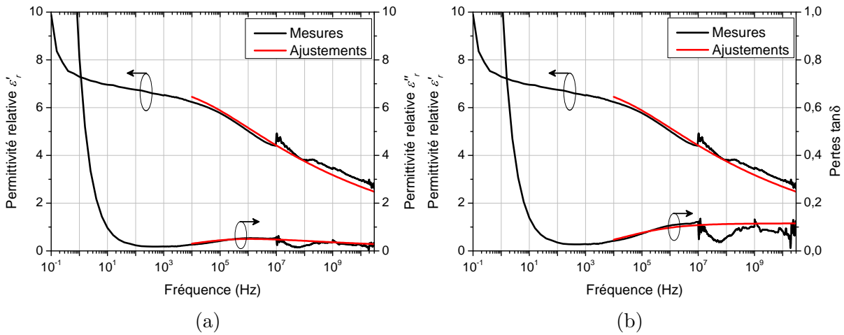
FIGURE 3.30 – Ajustements avec les formules de Havriliak et Negami de a) \varepsilon'_r et \varepsilon''_r et de b) \varepsilon'_r et \tan \delta issus des mesures sur PU87.
