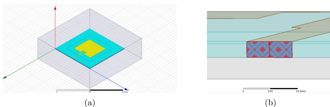
FIGURE 2.14 – a) Modèle 3D d’une antenne patch sur membrane de PU, entouré d’une boîte d’air pour les conditions aux limites du rayonnement et b) « LumpedPort » permettant de simuler l’excitation en mode quasi-TEM de l’antenne, sous HFSS®.
