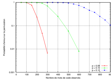
FIGURE 5.20 – Turbo-code parallèle poinçonné, probabilité d’erreur sur la permutation, pour le canal binaire symétrique, N = 64 .
