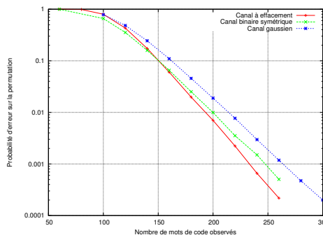
FIGURE 5.14 – Probabilité d’erreur sur la permutation pour une capacité de canal de 0.5, N = 64 et \mathcal{C}_2 = (1, \frac{1+D^2}{1+D+D^2}) .
