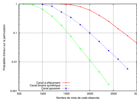
FIGURE 5.16 – Probabilité d’erreur sur la permutation pour une capacité de canal de 0.3, N = 64 et \mathcal{C}_2 = (1, \frac{1+D^2}{1+D+D^2}) .
