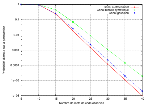
FIGURE 5.11 – Probabilité d’erreur sur la permutation pour une capacité de canal de 0.9, N = 64 et \mathcal{C}_2 = (1, \frac{1}{1+D}) .
