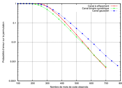
FIGURE 5.15 – Probabilité d’erreur sur la permutation pour une capacité de canal de 0.3, N = 64 et \mathcal{C}_2 = (1, \frac{1}{1+D}) .
