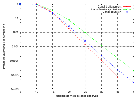
FIGURE 5.12 – Probabilité d’erreur sur la permutation pour une capacité de canal de 0.9, N = 64 et \mathcal{C}_2 = (1, \frac{1+D^2}{1+D+D^2}) .
