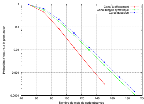
FIGURE 5.13 – Probabilité d’erreur sur la permutation pour une capacité de canal de 0.5, N = 64 et \mathcal{C}_2 = (1, \frac{1}{1+D}) .
