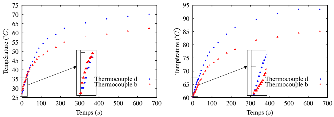
(b) Évolution de la température aux thermocouples b et d à une température extérieure de 27°C. (c) Évolution de la température aux thermocouples b et d à une température extérieure de 60°C.
