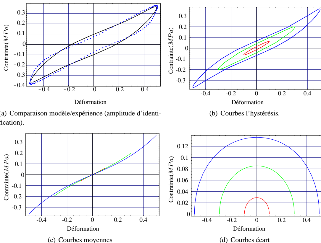
FIG. 3.5 – Résultats d'identification sur le modèle de Zener ; influence de l'amplitude sur les réponses du modèle (cisaillement 10%, 20%, 50%, f = 3.5Hz , T = 23^{\circ}C ).
