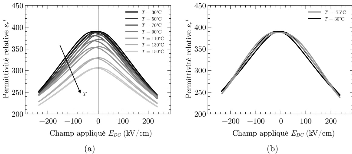
FIGURE 3.4 – Permittivité relative en fonction du champ appliqué pour différentes températures à une fréquence de 10 kHz.
