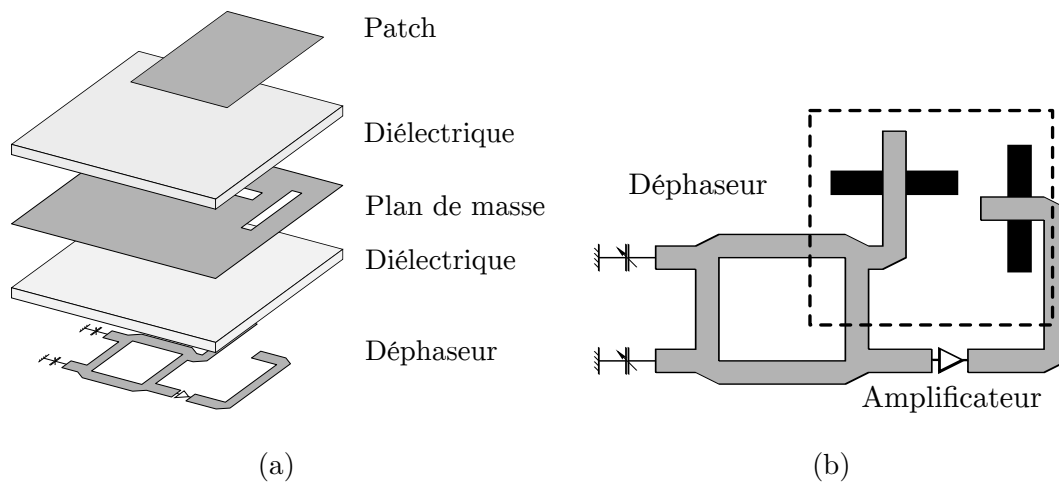
FIGURE 1.8 – Cellule utilisant un déphaseur à base d’hybride 90^\circ et amplificateur [32].
