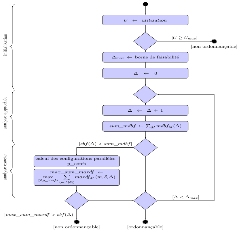
FIGURE 4.1 – Diagramme d'activité du test d'ordonnançabilité pour E-TDL
