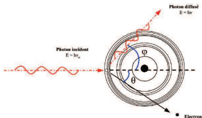
Figure II-1 : Effet Compton.
