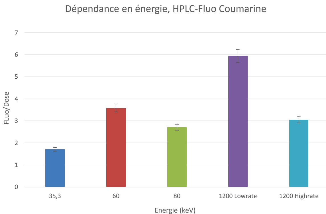
Figure III-9 : Pentas de formation de 7OHC en fonction de l'énergie d'irradiation, mesurée au HPLC-Fluo. Erreur fixée à 5%
