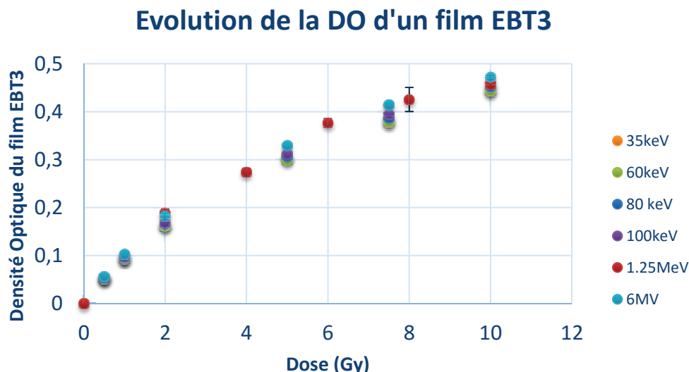
Figure III-20 : Irradiation à plusieurs énergies de films EBT3. La réponse générale du film est remarquablement similaire pour une gamme d'énergie très étendue.
