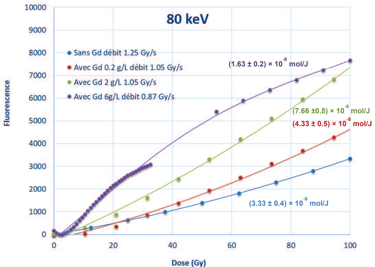
Figure III-16 : Maximum de fluorescence de RN formé sous irradiation monochromatique à 80 keV en fonction de la dose. Solution initiale de RNO de concentration 5 \times 10^{-4} M. (Baldacchino et al. , non publié)
