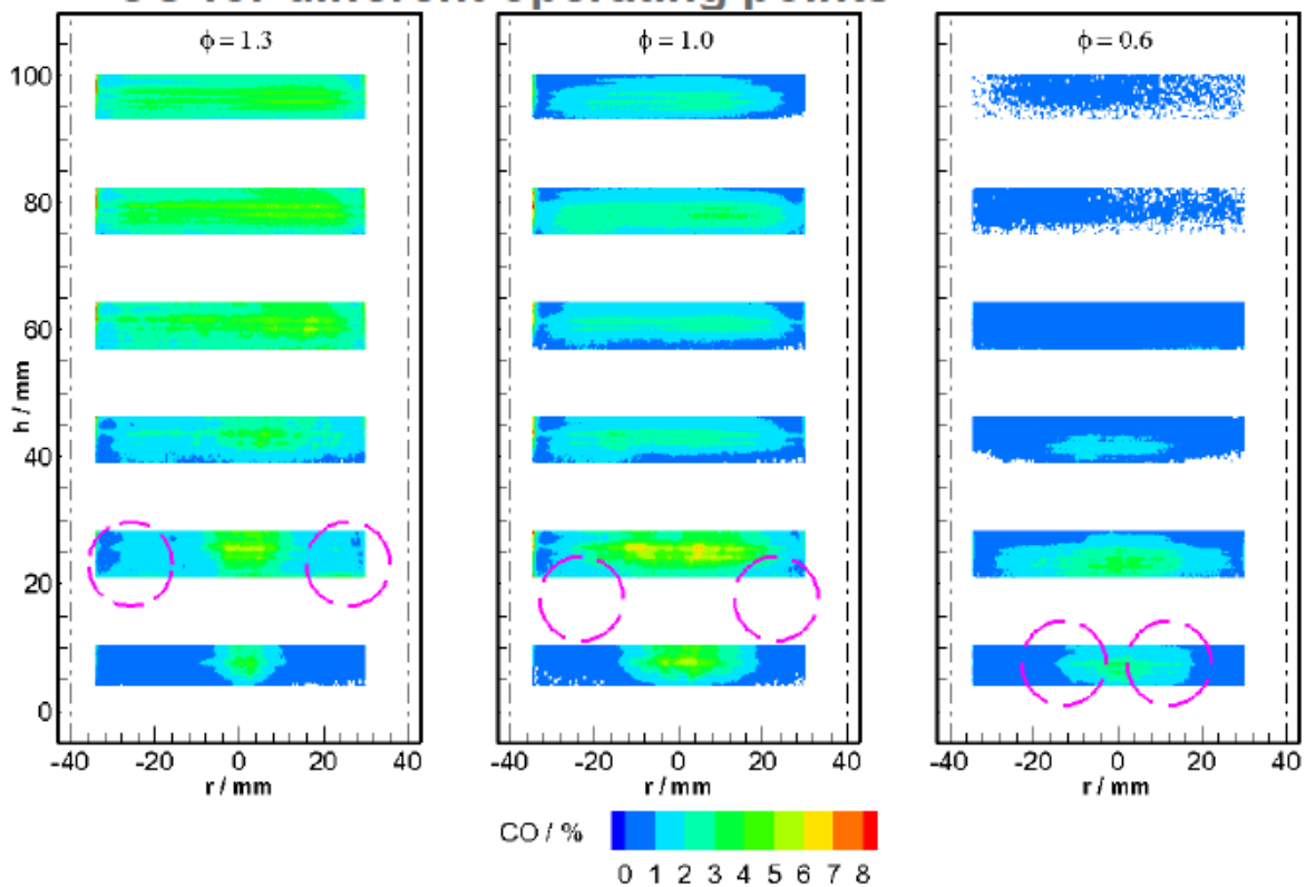
FIGURE 5.16 – Distribution spatiale de la concentration de CO mesurée dans une flamme de diffusion \text{CH}_4/\text{air} à 5 bar pour trois richesses, 1,3, 1 et 0,6 [134]. I_L=70 \text{ MW}\cdot\text{cm}^{-2} , \Delta\sigma_L=0,05 \text{ cm}^{-1} .
