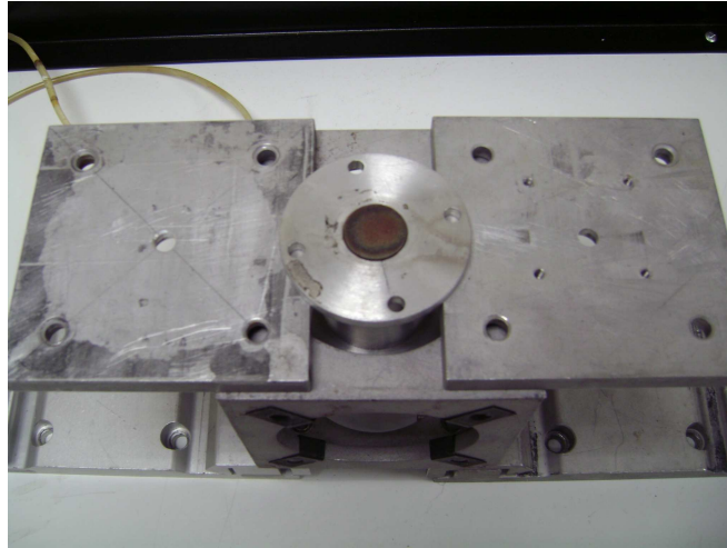
FIGURE 3.3 – Brûleur à flamme plate utilisé pour les mesures LIF à deux photons de CO.
