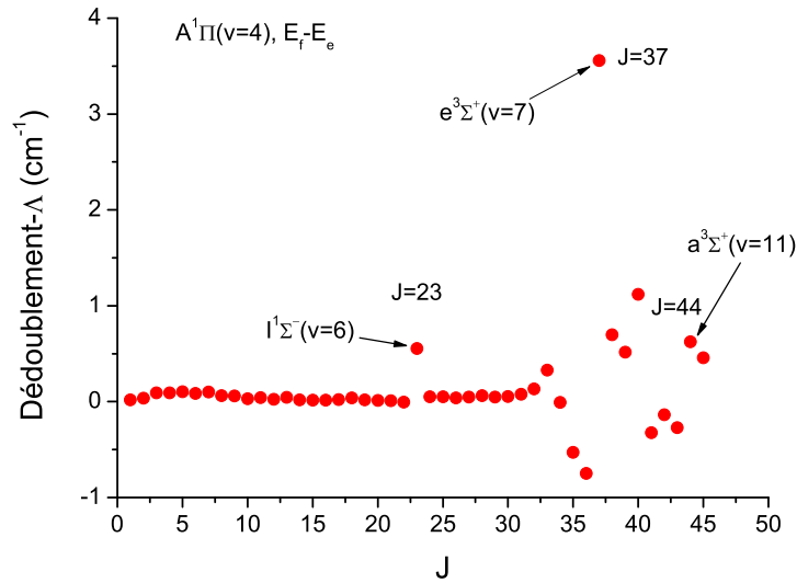
FIGURE 2.10 – Dédoublé-A de CO en fonction du nombre quantique J dans l'état A^1\Pi ( v = 4 ) [140].
