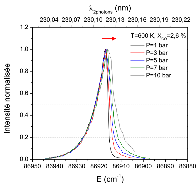
FIGURE 4.14 – Evolution de la forme du spectre d'excitation de CO expérimental avec la pression à 600 K dans les mêmes conditions que la figure 4.13.
