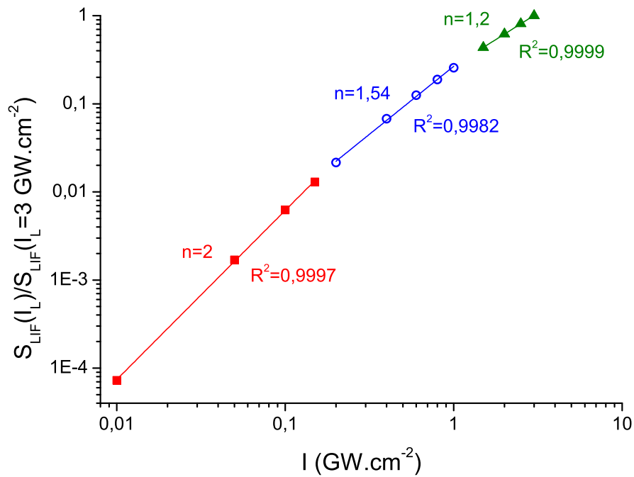
FIGURE 2.28 – Calcul du signal de fluorescence de CO normalisé par le signal obtenu à 3 \text{ GW.cm}^{-2} en fonction de l'intensité laser ( I_L ). T=300 \text{ K} , P=1 \text{ bar} , N_2=78,4 \% , O_2=19 \% et CO=2,6 \% . Variation de S_{LIF} en I_L^n , n déterminé par la pente de la droite.
