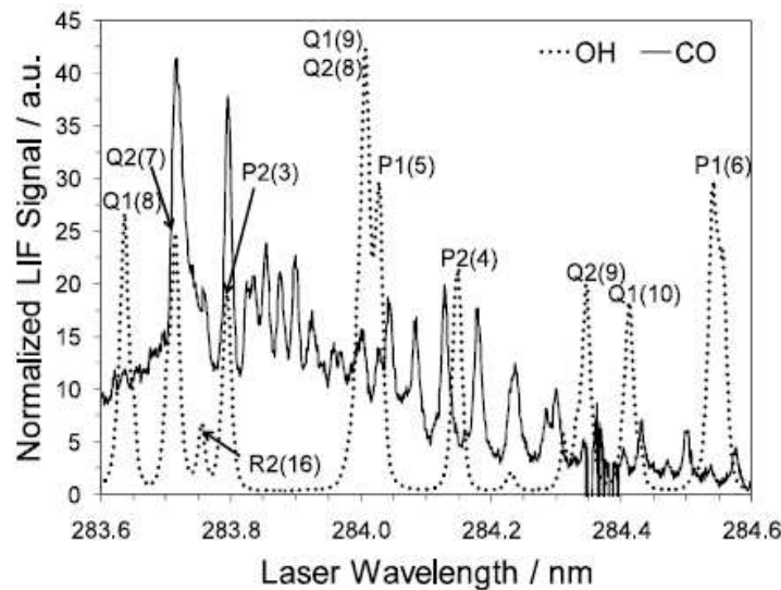
FIGURE 2.9 – Superposition du spectre de rotation de la bande A(4)-X(0) de CO avec le spectre de rotation de la bande A(1)-X(0) de OH. Le spectre d'excitation de CO est mesuré pour une fraction molaire de 7,5 % de CO dans une atmosphère de \text{N}_2 à 300 K, 1 bar. Le spectre d'excitation de OH est mesuré dans une flamme de méthane/air à 1 bar [113].
