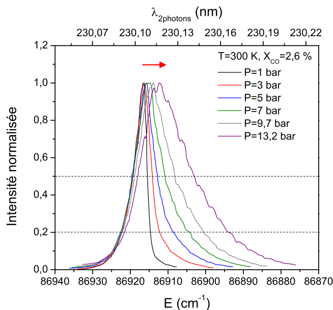
FIGURE 4.13 – Evolution de la forme du spectre d'excitation de CO expérimental avec la pression à 300 K. La fraction molaire de CO est de 2,6 % dilué dans de l'air sec. \Delta\sigma_L=0,8 \text{ cm}^{-1} (FWHM), I_L=0,1 \text{ GW.cm}^{-2} et détection avec le filtre Semrock.
