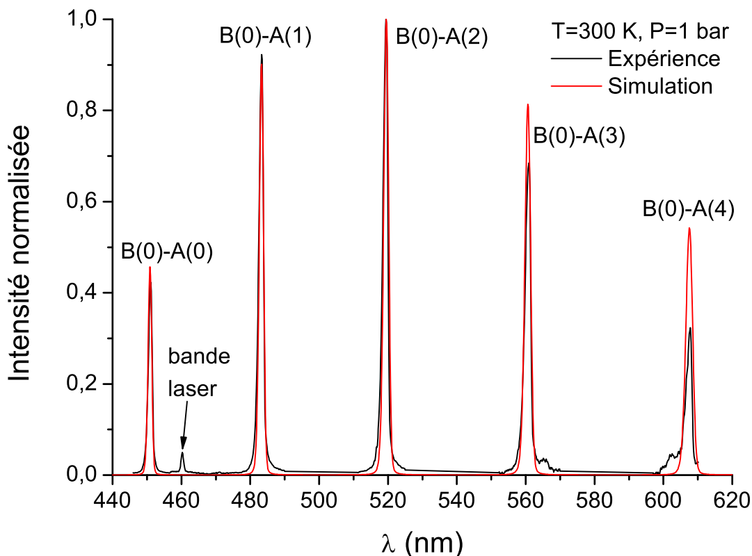
FIGURE 4.1 – Spectres de fluorescence de CO dispersée mesuré et simulé pour une fraction molaire de CO de 2,6 % dilué dans de l'air sec à 300 K, 1 bar. \lambda_L=230,105 nm, \Delta\sigma_L=0,7 cm -1 (FWHM) et I_L=0,15 GW.cm -2 . La résolution du spectrographe est de 1 nm. La dispersion est de 0,138 nm/pixel. Accumulation sur 1000 tirs laser.
