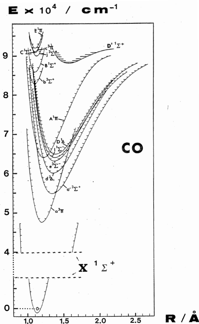
FIGURE 2.1 – Courbes d'énergie potentielle des différents états électroniques de la molécule CO issues de Le Floch [140].
