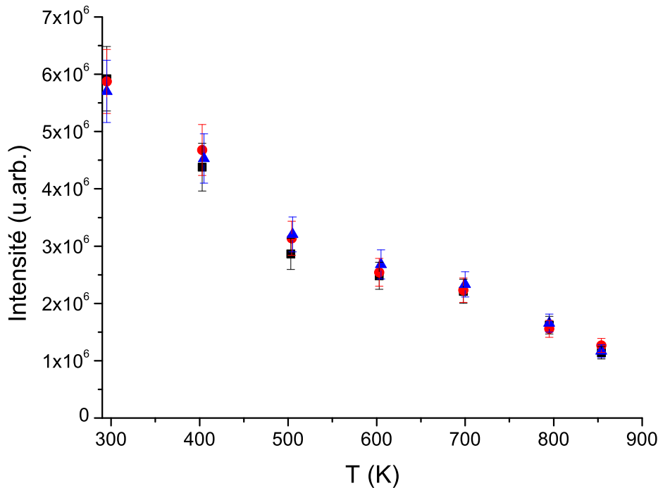
FIGURE 3.28 – Variation du signal de fluorescence intégrée de la transition B(0)-A(1) de CO avec la température, pour une fraction molaire de CO égale à 2,6 % dans de l’air sec à P=1 bar. I_L=0,146 GW.cm -2 , \lambda_L=230,105 nm.
