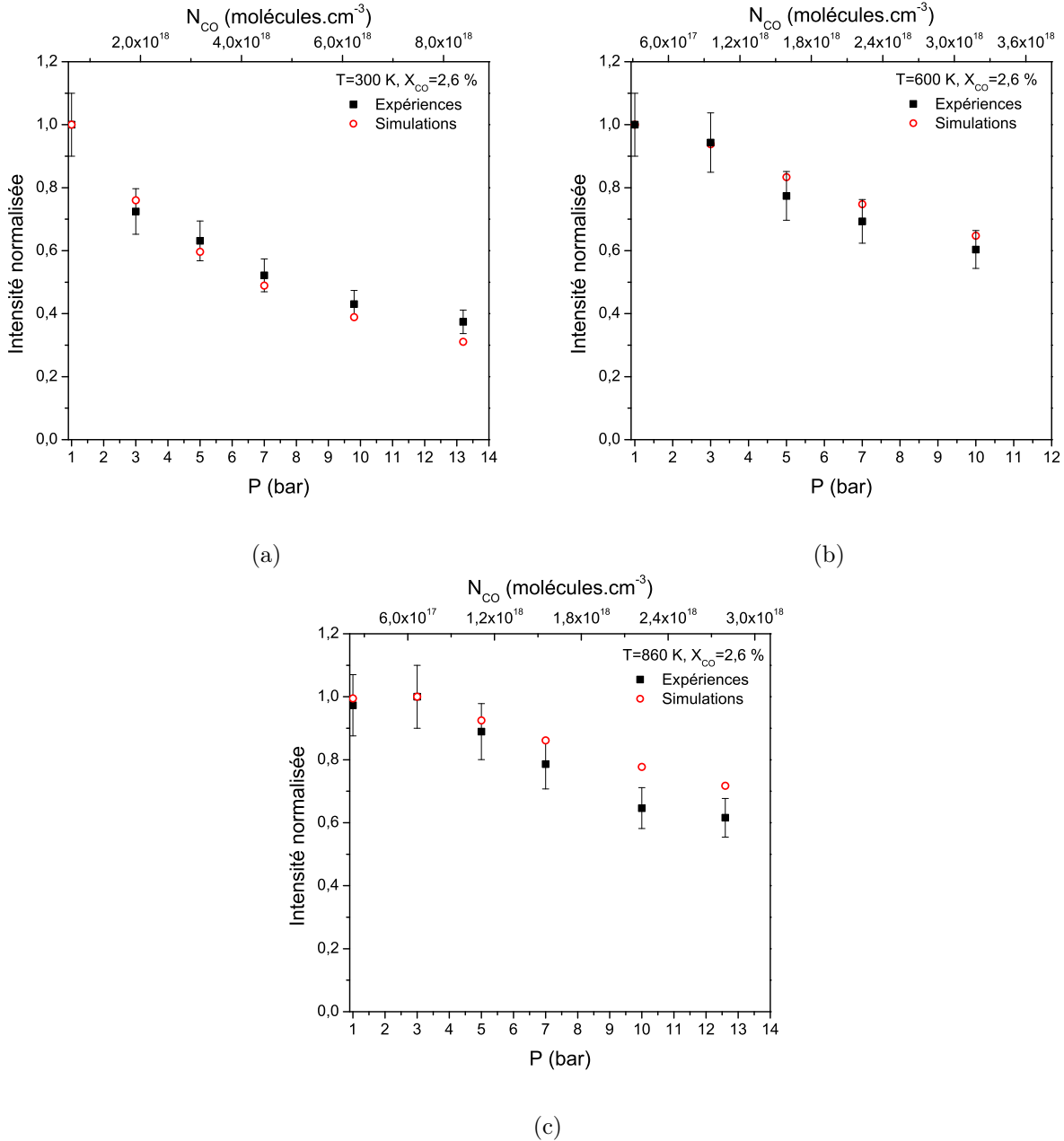
FIGURE 4.12 – Variation de l’intensité du pic de la branche Q de CO avec la pression mesurée et calculée à 300 K (a), 600 K (b) et 860 K (c). X_{CO}=2,6 %. I_L=0,076 GW.cm -2 , \Delta\sigma_L=0,8 cm -1 (FWHM) et détection avec le filtre Semrock.
