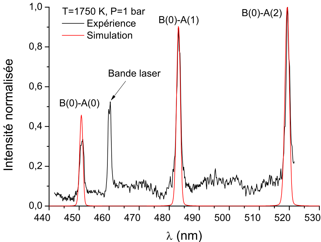
FIGURE 4.3 – Spectres de fluorescence dispersée de CO mesuré et simulé en flamme méthane/air pour une richesse 1,16 à 1 bar et à h=0,7 mm. \lambda_L=230,104 nm, \Delta\sigma_L=0,7 \text{cm}^{-1} (FWHM) et I_L=0,10 \text{GW}\cdot\text{cm}^{-2} . La résolution du spectrographe est de 1 nm. La dispersion est de 0,138 nm/pixel. Accumulation sur 1000 tirs laser.
