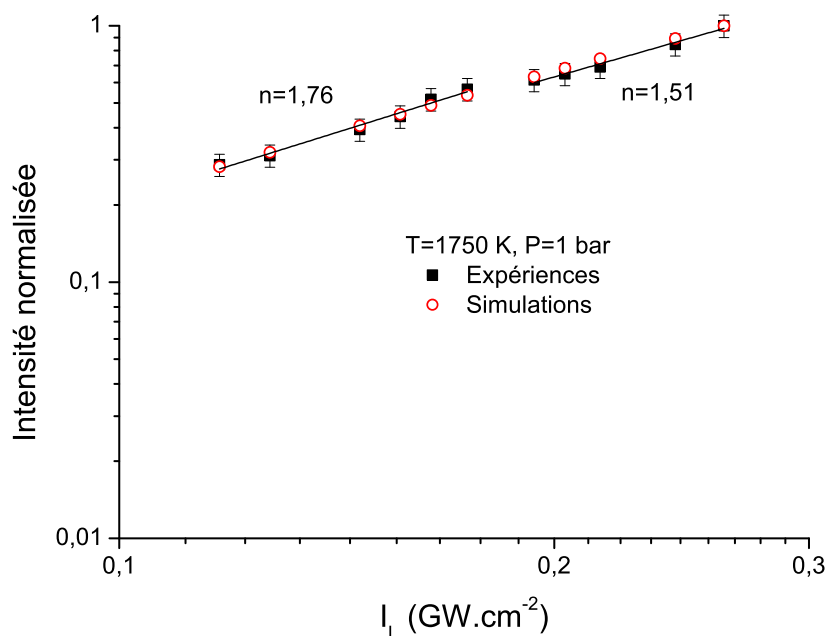
FIGURE 3.14 – Evolution du signal de fluorescence de CO en fonction de l'intensité laser dans la flamme de prémélange méthane/air. T=1750 K, D_{air}=1,8 \text{ ln.min}^{-1} , D_{CH_4}=0,22 \text{ ln.min}^{-1} , \phi=1,16 . Intensité relative par rapport à l'intensité laser maximale. Excitation laser à 230,104 nm, détection avec le filtre Semrock.
