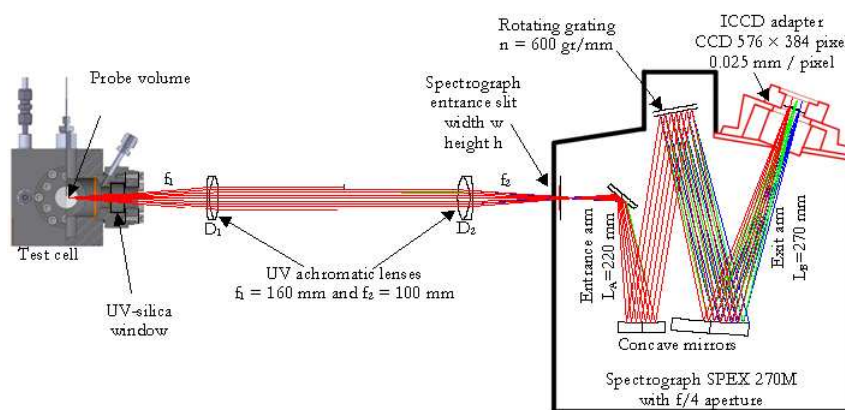
FIGURE 3.6 – Système optique permettant l'enregistrement des spectres de fluorescence dispersée de CO [228].
