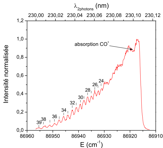
FIGURE 3.23 – Spectre d'excitation corrigé mesuré en flamme \text{CH}_4/\text{air} . T=1750 K, P=1 bar. I_L=0,27 \text{GW}\cdot\text{cm}^{-2} , détection avec le filtre Semrock. N.B. : avec 0,27 \text{GW}\cdot\text{cm}^{-2} , S_{LIF} varie comme I_L^{1,51} qui est pris en compte dans la correction de l'intensité.
