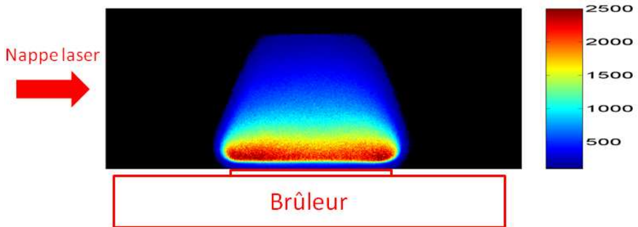
FIGURE 5.9 – Distribution spatiale du signal LIF de OH dans la flamme méthane/air pour une richesse de 1,16. I_L = 22 \text{ MW.cm}^{-2} . Taille de l'image : 48,7 \times 18,7 \text{ mm}^2 (largeur \times hauteur).
