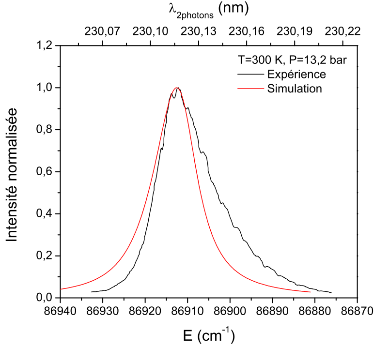
FIGURE 4.20 – Comparaison de la forme du spectre d'excitation de CO calculé et mesuré à 13,2 bar et 300 K avec -\Delta\sigma_s=0,218P+0,00158P^2 .
