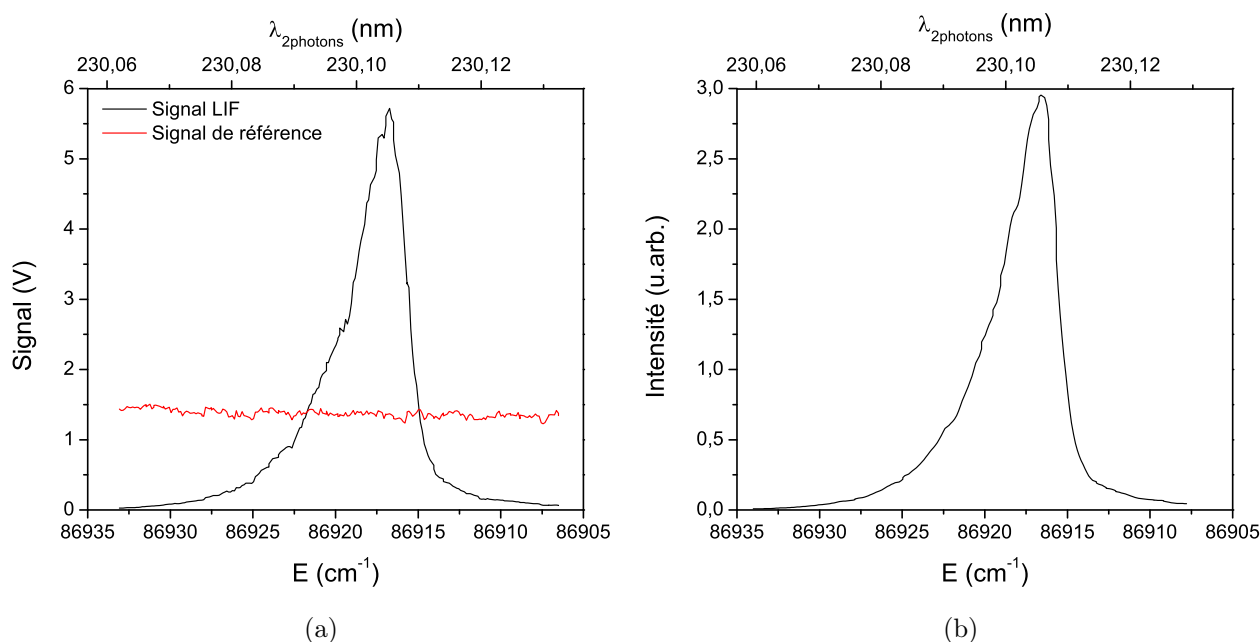
FIGURE 3.20 – Spectres d'excitation de la transition B(0)-X(0) de CO non corrigé (a) et corrigé par les fluctuations d'énergie laser au carré (b). T=300 \text{ K} , P=1 \text{ bar} , X_{CO}=2,6 \% dans de l'air sec. I_L=0,1 \text{ GW.cm}^{-2} , détection avec le filtre Semrock. Les longueurs d'onde d'excitation à deux photons sont données dans le vide.
