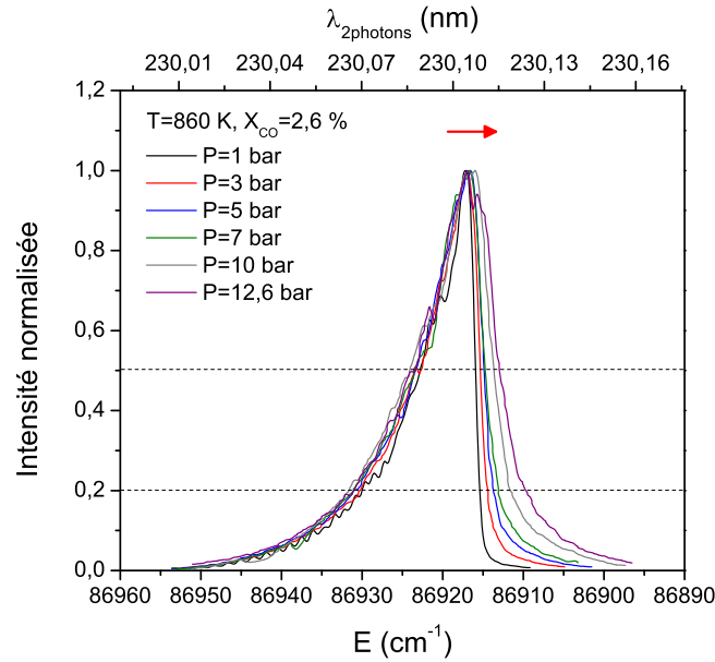
FIGURE 4.15 – Evolution de la forme du spectre d’excitation de CO expérimental avec la pression à 860 K dans les mêmes conditions que la figure 4.13.
