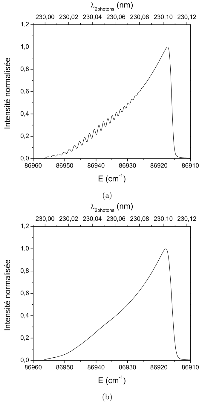
FIGURE 5.2 – Spectre d’excitation LIF-CO simulé pour \Delta\sigma_L=0,8 \text{ cm}^{-1} (a) et \Delta\sigma_L=1,4 \text{ cm}^{-1} (b). T=1750 \text{ K} , P=1 \text{ bar} , N_2=78 \% , CO_2=8 \% , H_2O=10 \% et CO=4 \% . Détection avec une bande passante centrée à 485 \text{ nm} ( FWHM=25 \text{ nm} ).
