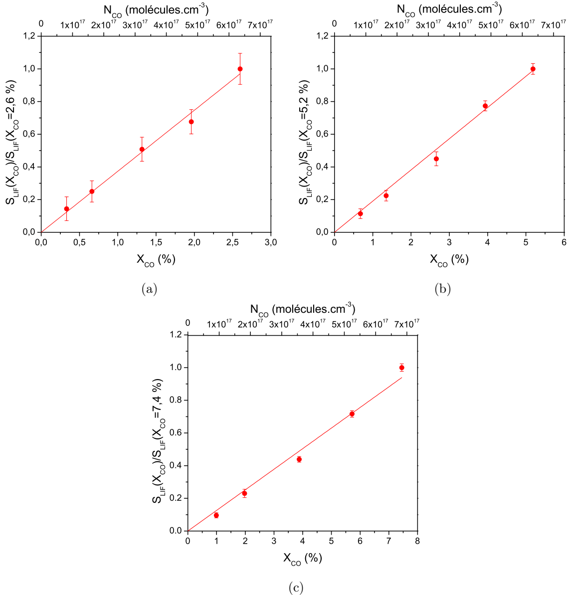
FIGURE 3.29 – Linéarité du signal de fluorescence intégrée de la transition B(0)-A(1) de CO avec la fraction molaire de CO dans de l'air sec à 300 K (a), 600 K (b) et 860 K (c), P=1 bar. I_{laser}=0,146 GW.cm -2 , \lambda_{laser}=230,105 nm.
