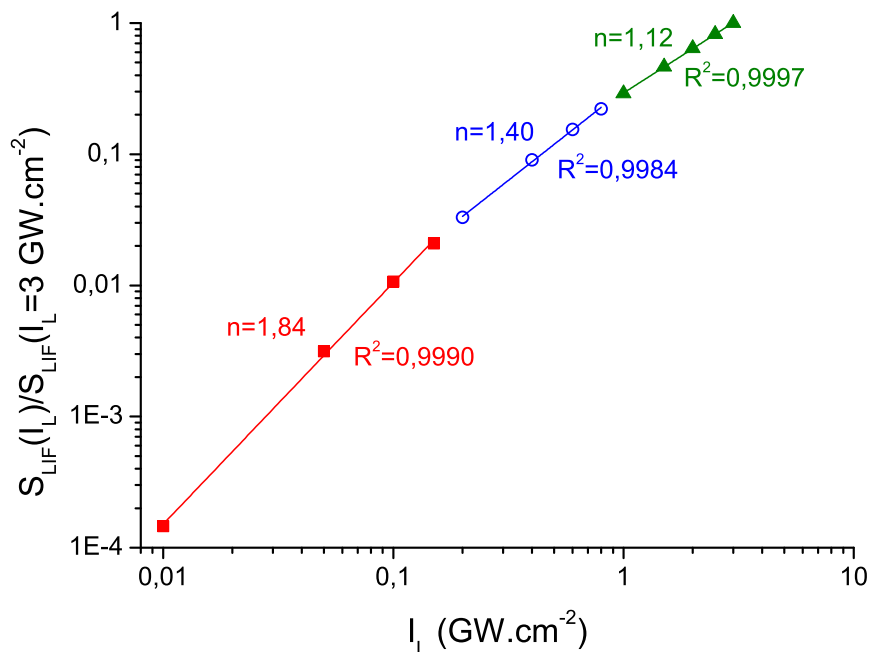
FIGURE 2.29 – Calcul du signal de fluorescence de CO normalisé par le signal obtenu à 3 \text{ GW.cm}^{-2} en fonction de l'intensité laser ( I_L ). T=1750 \text{ K} , P=1 \text{ bar} , N_2=78 \% , CO_2=8 \% , H_2O=10 \% et CO=4 \% . Variation de S_{LIF} en I_L^n , n déterminé par la pente de la droite.
