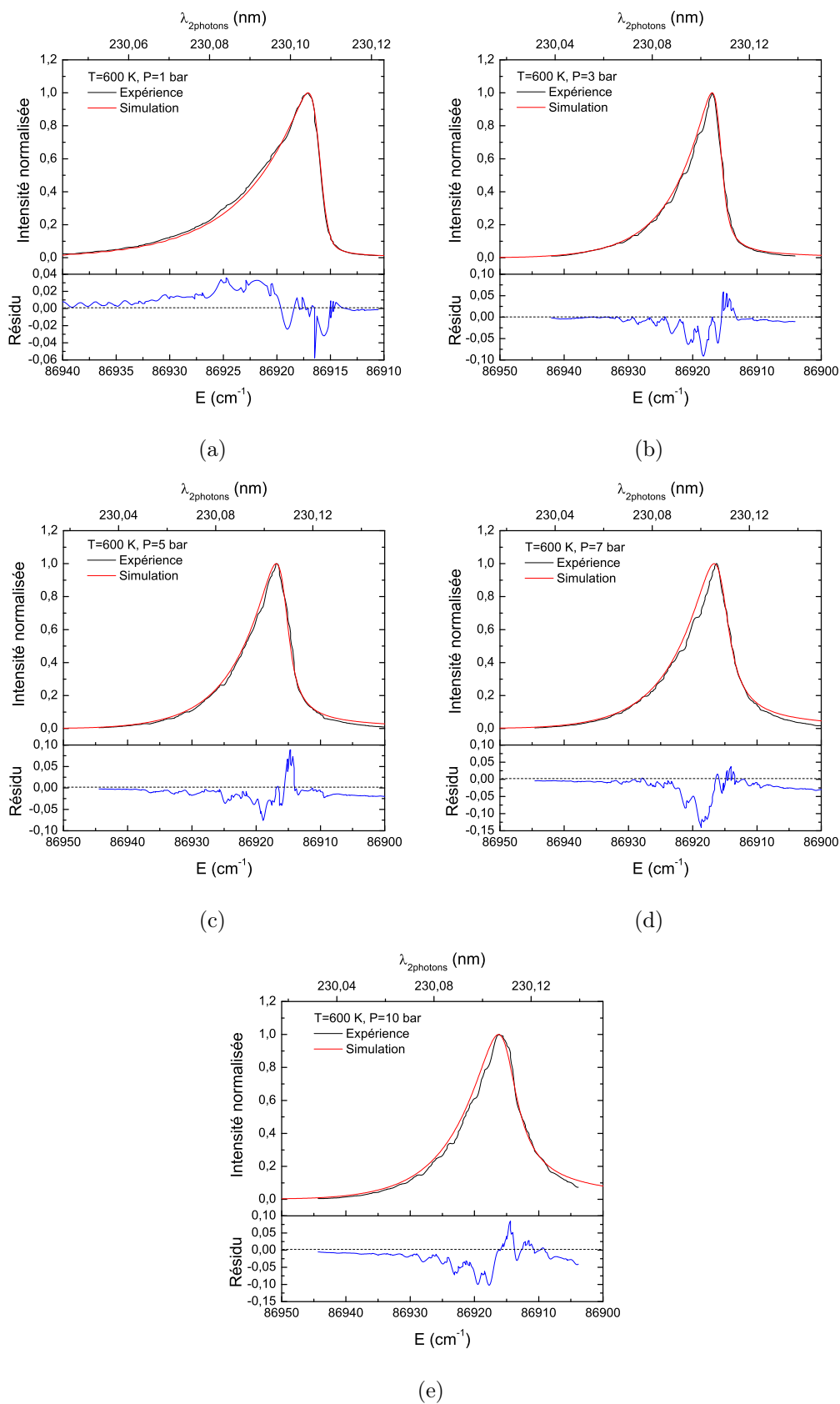
FIGURE 4.34 – Calculs des spectres d'excitation de CO à 1 bar (a), 3 bar (b), 5 bar (c), 7 bar (d), 10 bar (e). T=600 \text{ K} . Mêmes conditions que la figure 4.33. Comparaison avec les spectres mesurés.
