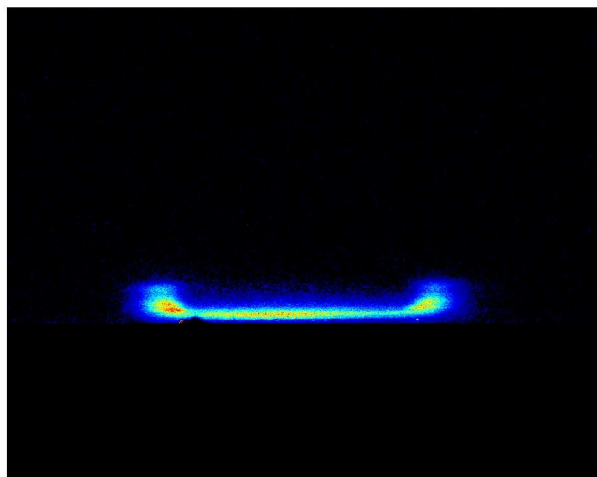
FIGURE 5.7 – Image PLIF-CO corrigée du bruit laser. Le champ d'observation est de 50×50 mm 2 . I_L=0,28 GW.cm -2 .
