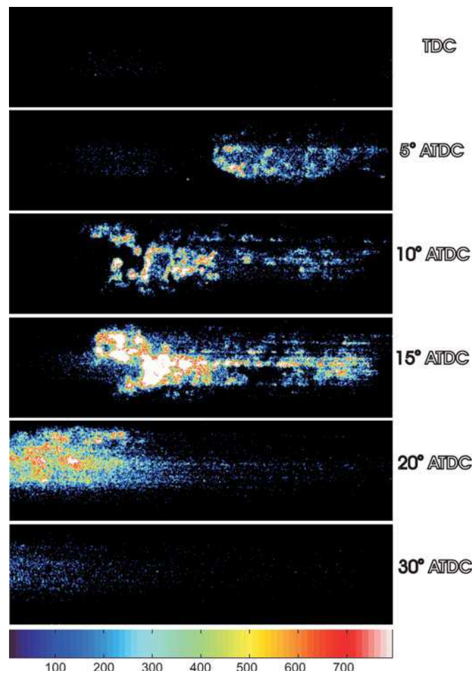
FIGURE 5.15 – Distribution spatiale de CO pour différents angles de vilebrequin dans un moteur automobile à allumage commandé alimenté en isoctane à 1 bar [133]. I_L=50 MW.cm -2 , \Delta\sigma_L=0,3 cm -1 . 47 \times 12 mm 2 (largeur \times hauteur).
