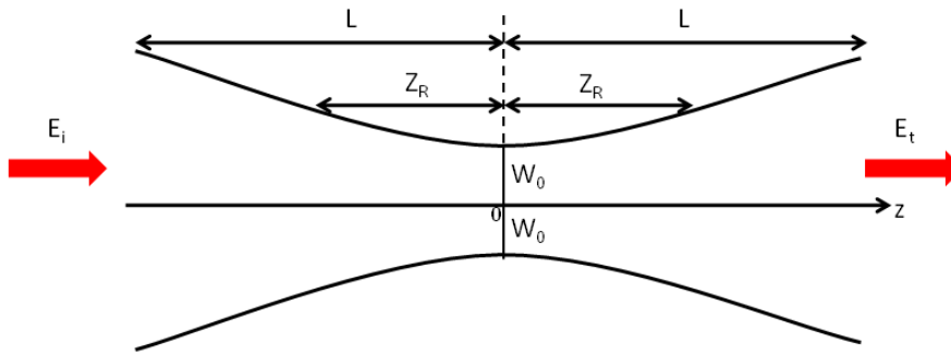
FIGURE 3.15 – Faisceau Gaussien.
