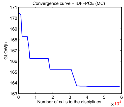
Figure 18.15: Courbe de convergence d'IDF-PCE
