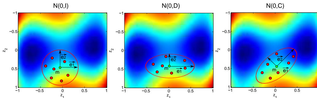
Figure 18.8: Espace de recherche pour différentes matrices de covariance
