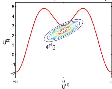
Figure 18.5: Analyse de fiabilité avec \phi^{\mathbf{e}1}(\cdot) Figure 18.6: analyse de fiabilité avec \phi^{\mathbf{e}2}(\cdot) Des approches basées sur CMC [Zhang et al., 2010] ou FORM [Qiu et al., 2008] ont été proposées pour résoudre ce type de problèmes au travers d'une double boucle. À chaque itération de l'optimiseur, une analyse de fiabilité par CMC ou FORM est réalisée. Cependant, le coût de calcul engendré par ce type d'approche est prohibitif. Afin d'éviter ces deux niveaux de calcul, CMC ainsi que IS ont été étendus à la prise en compte directe d'intervalles. Néanmoins, ces méthodes permettent
