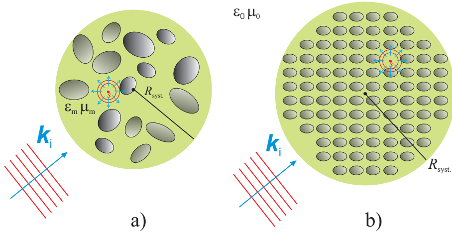
FIG. 2 – Système inhomogène immergé dans un milieu sphérique de géométrie sphérique de rayon R_{\text{sys}} et ayant des paramètres constitutifs \varepsilon_m \neq \varepsilon_0 et \mu_m \neq \mu_0 .
