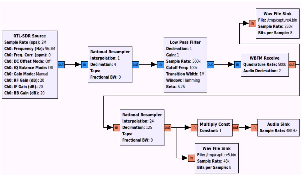
Figure V.11: Schéma bloc utilisé pour la capture
