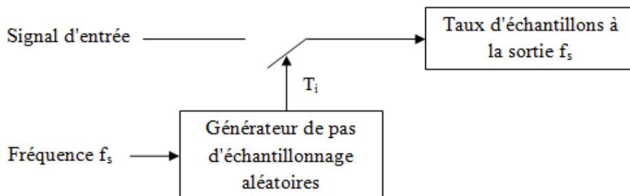
Figure III.3: Schéma de principe de l'échantillonnage aléatoire
