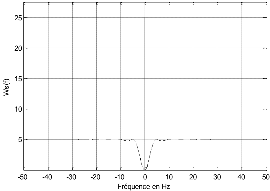
b: Jitter stationnaire [-0.5T, 0.5T] , \beta=5\text{Hz}
