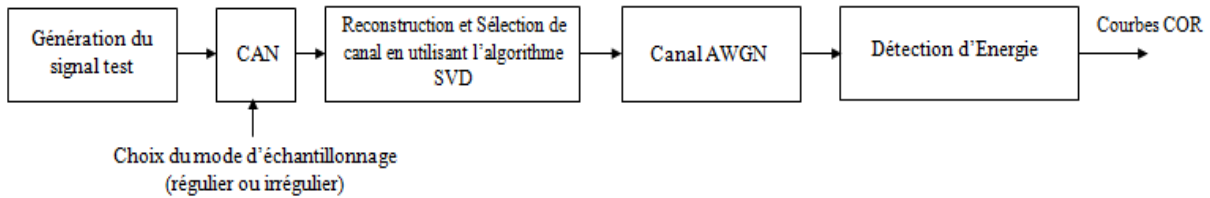
Figure IV.7: Diagramme en blocs de l'approche
