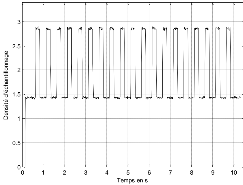
d: Loi uniforme de \tau_n sur [-1.4T, 1.4T] , ( LR=\sigma/T=0.808 )
