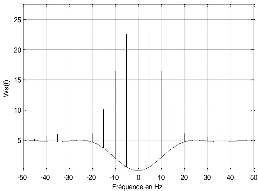
b: Jitter sur [-0.1T, 0.1T] , \beta=5\text{Hz}
