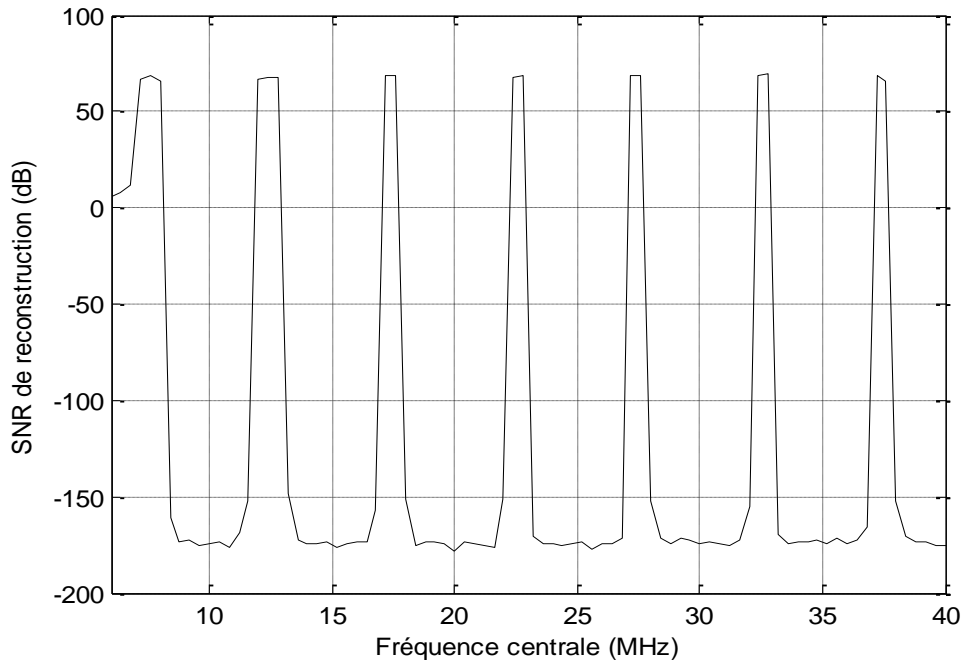
Figure II.13: Variation du SNR de reconstruction en fonction de la fréquence centrale en mode d'échantillonnage uniforme (cas de l'algorithme SVD)
