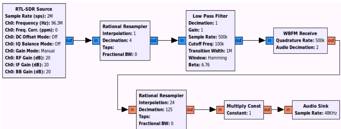
Figure V.7: Schéma final sous GNU Radio
