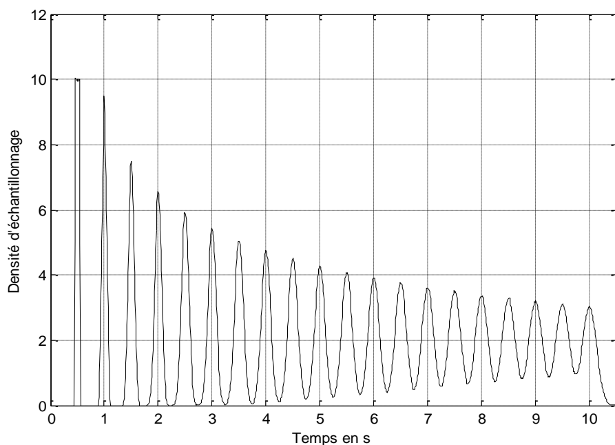
a: Loi uniforme de \tau_n sur [-0.1T, 0.1T] , ( LR=\sigma/T=0.058 )
