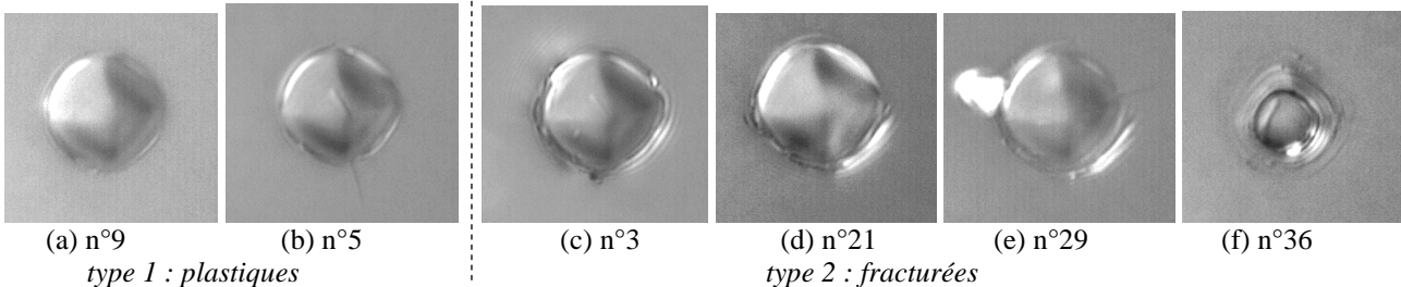
Figure 60 : différents types d'indentations sphériques (avant tir laser) :
