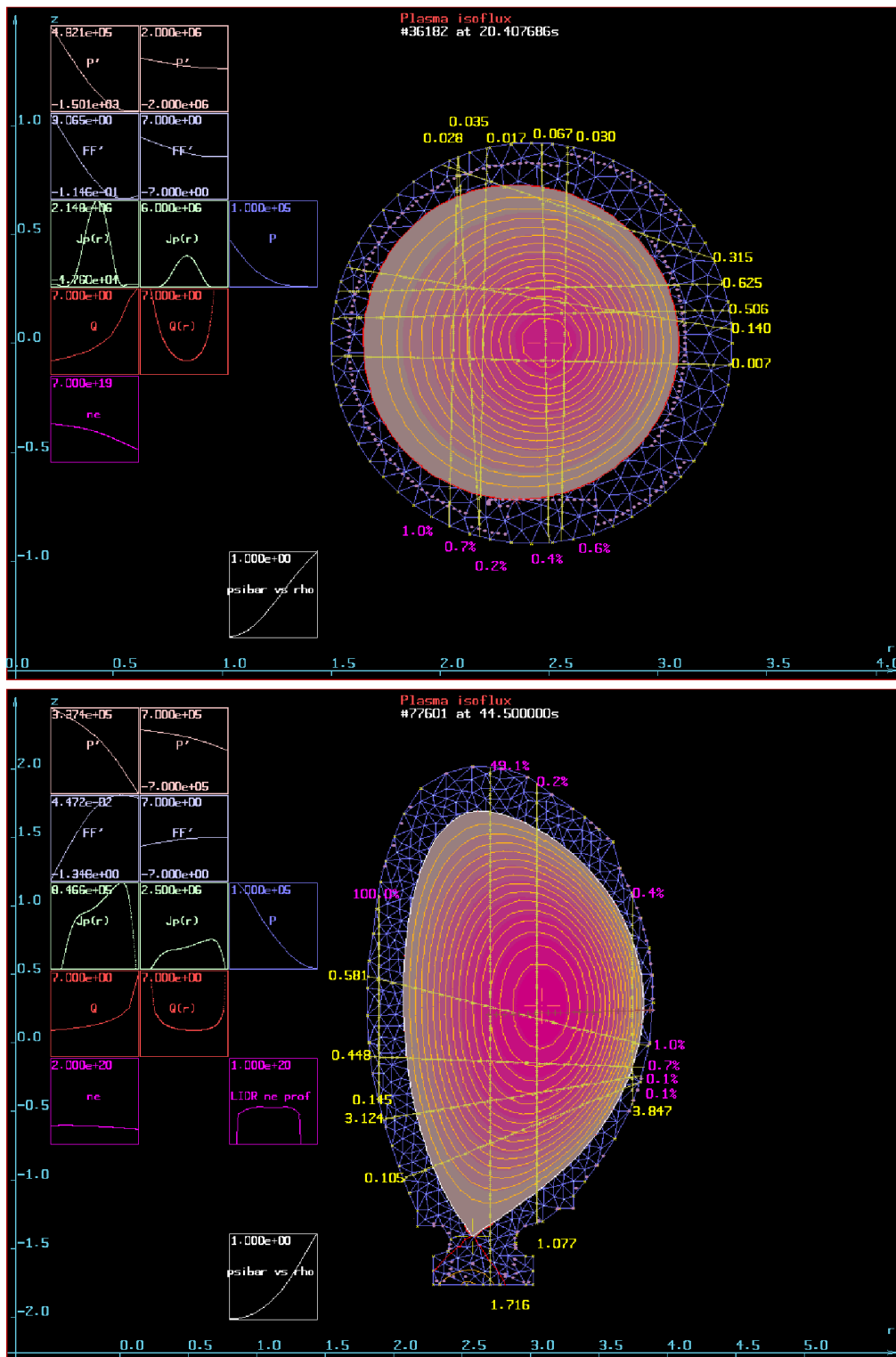
FIGURE 1.2 – Equilibres reconstruits. ToreSupra en haut et JET en bas. Le maillage du domaine apparaît là où le plasma en couleur n'est pas présent. Dans le plasma les isoFlux sont représentées depuis l'axe magnétique jusqu'à la frontière. Les cordes des mesures d'interférométrie et polarimétrie sont représentées en jaune. Les graphes sur la gauche permettent de visualiser différents profils comme les fonctions p' et ff' identifiées, la densité de courant toroidal fonction de r sur l'axe magnétique z = z_a , la pression, le facteur de sécurité q et la densité électronique identifiée.
