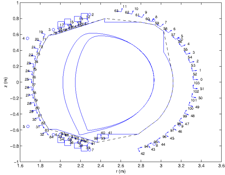
FIGURE 1.6 – Section poloidale du tokamak WEST. Deux frontières plasma différentes calculées à partir du code CEDRES++ sont représentées. Les bobines de mesures du champ poloidal sont représentées par des flèches et numérotées de 0 à 103. Les boucles de flux sont représentées par des cercles et numérotées de 0 à 9. Les quatre bobines basses du divertor et les quatre bobines hautes sont représentées. Le contour du limiteur est également représenté ainsi que son enveloppe convexe (en tirets) qui est utilisé comme contour \Gamma_V i.e la frontière du domaine de calcul pour le code EQUINOX.
