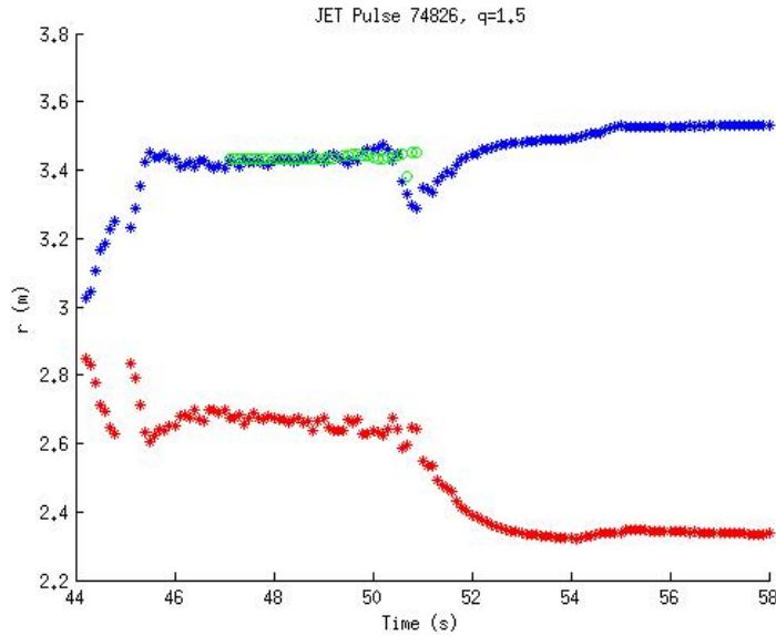
FIGURE 1.3 – Comparaison de la position des surfaces magnétiques q = 3/2 au cours d'une décharge JET. En rouge et bleu sorties d'EQUINOX côté fort et faible champ. En vert position trouvée par analyse MHD indépendante basée sur des mesures ECE (electron cyclotron emission).
