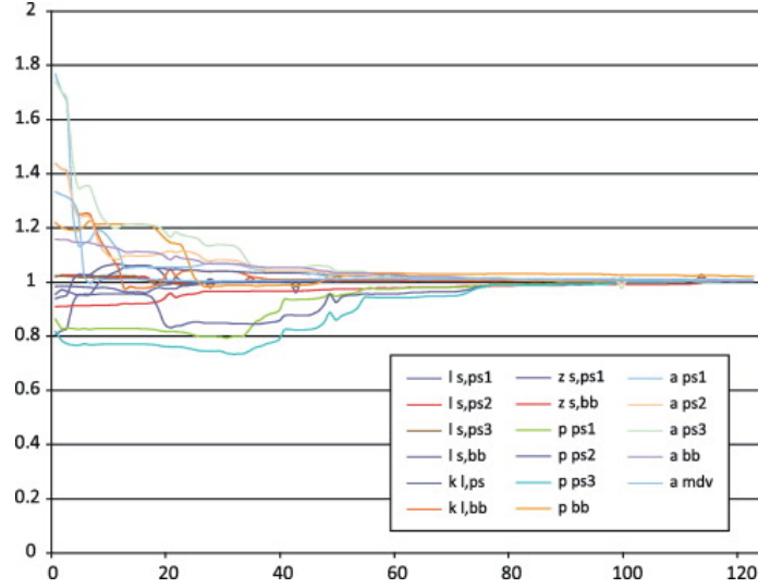
FIGURE 2.3 – Variations des paramètres en fonction des itérations de minimisation. Les valeurs sont normalisées par les valeurs optimales.
