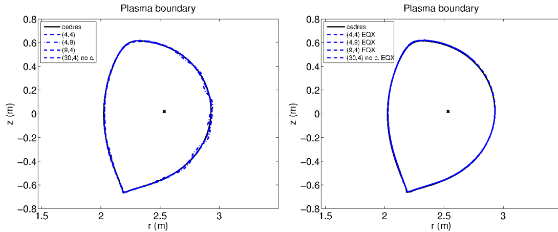
FIGURE 1.7 – Frontières plasma reconstruites. Gauche : à partir des harmoniques toroidales seules. Les frontières calculées avec (n^e = 4, n^i = 4) ou (n^e = 9, n^i = 4) et (n^e = 30, n^i = 4) sans prendre en compte les bobines de champ poloidal (no c.) sont presque superposées avec la frontière de référence calculée avec le code CEDRES++. La frontière calculée avec (n^e = 4, n^i = 9) présente des irrégularités. Droite : mêmes frontières calculées avec EQUINOX et interpolation des données sur le contour \Gamma_V de la Fig. 1.6
