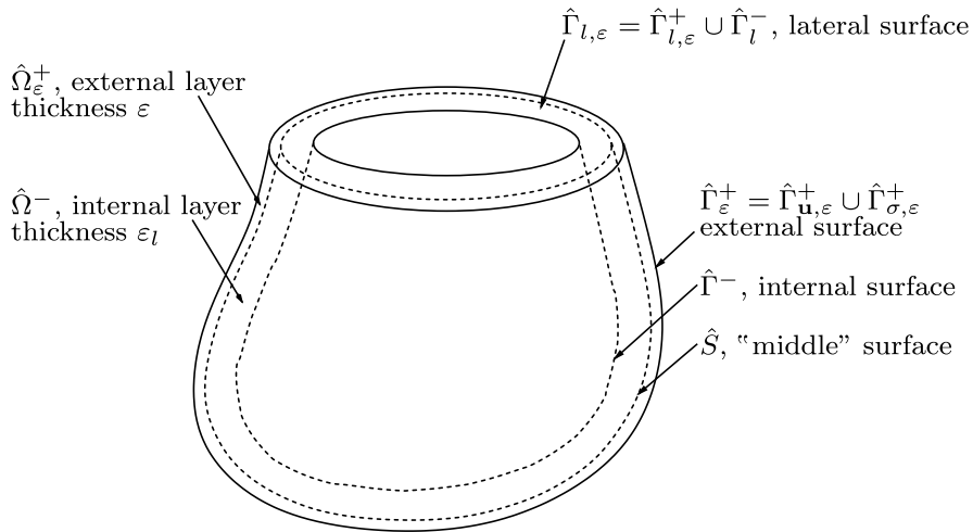
Fig. 2. The domain \hat{\Omega}_\varepsilon = \hat{\Omega}_\varepsilon^+ \cup \hat{\Omega}^- .
