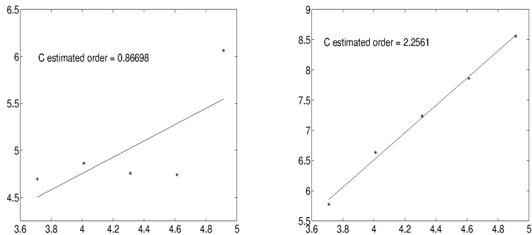
FIGURE 2.6 – -\log(\text{Erreur}) versus -\log(\Delta t) . Courbes de convergence pour le schéma de splitting classique à gauche, et pour le schéma d'ordre 2 proposé à droite.
