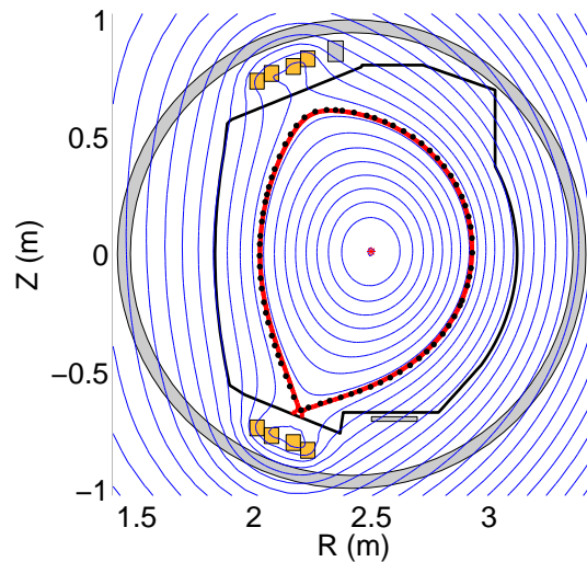
FIGURE 1.9 – Iso- \psi calculées par CEDRES++ en mode inverse statique. Les points noirs représentent la frontière désirée et la courbe rouge la frontière calculée.
