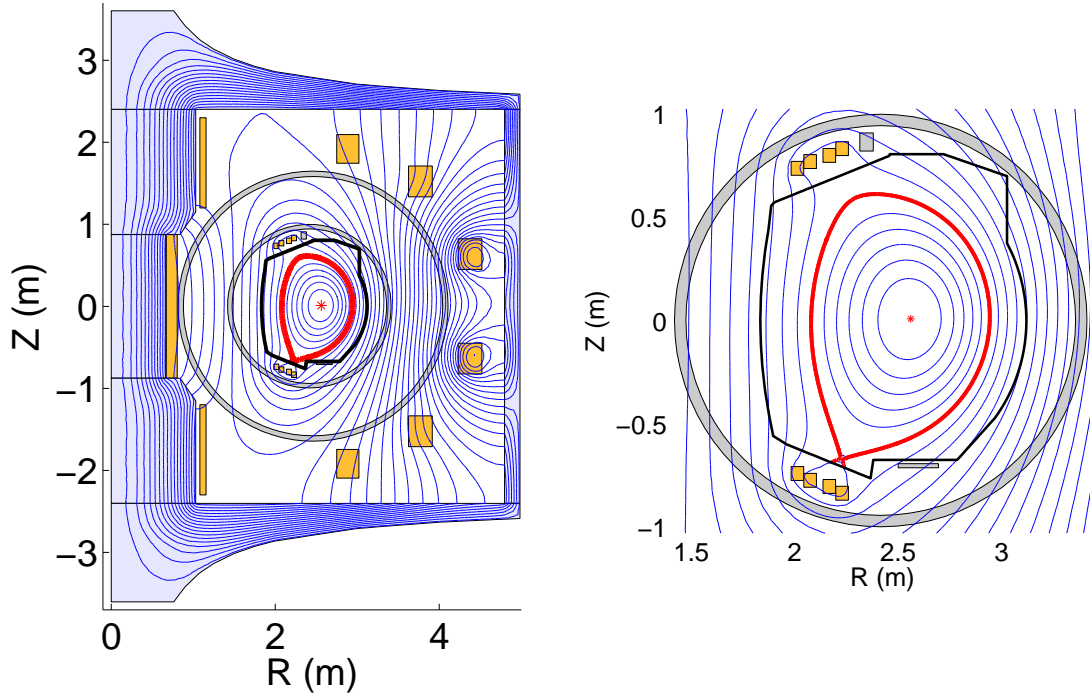
FIGURE 1.8 – Exemple de calcul d'équilibre pour le tokamak WEST représentant les isoflux dans le plan poloidal. Gauche : vue d'ensemble. Droite : zoom sur la chambre à vide. Le fer est représenté en bleu clair, les bobines de champ poloidal en orange et les structures passives en gris clair (chambre à vide et éléments de stabilisation verticale). La courbe noire est le limiteur. La courbe rouge est la frontière du plasma calculée. L'axe magnétique est également représenté en rouge.
