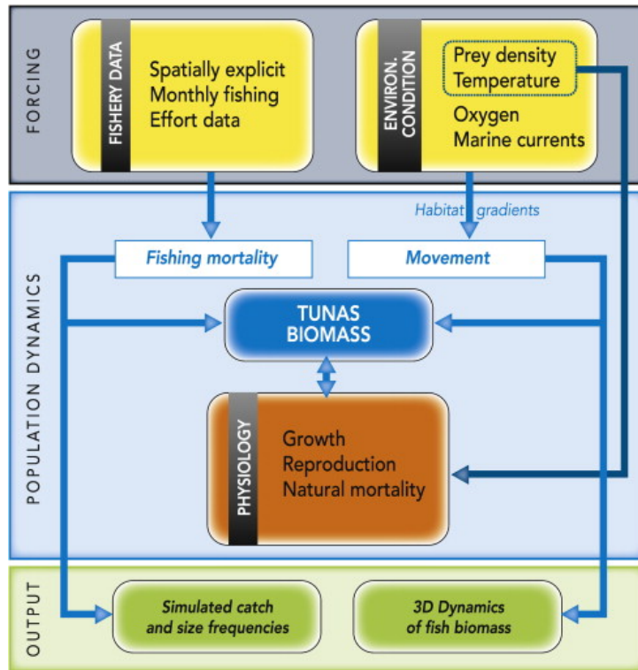
FIGURE 2.1 – Schéma de synthèse présentant les forçages, les processus affectant la dynamique de population et les sorties du modèle APECOSM-E
