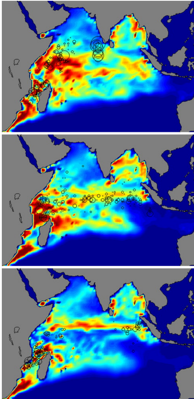
FIGURE 2.2 – Population exploitable de thons Listao calculée versus captures observées (cercles) dans l’océan Indien. Avril 1993, février 1998 et avril 1998
