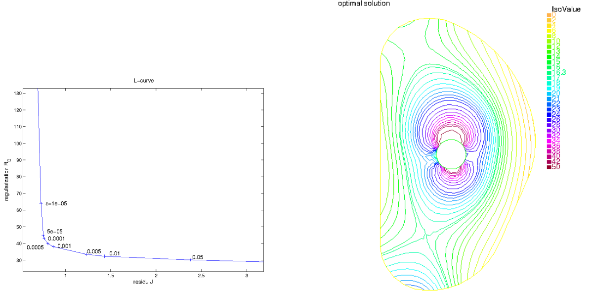
FIGURE 1.5 – Reconstruction du flux poloidal dans le vide pour la géométrie ITER. Gauche : L-curve donnant \varepsilon = 5 \times 10^{-4} . Droite : Reconstruction de \psi dans le domaine \Omega
