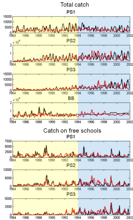
FIGURE 2.4 – Comparaison entre les captures agrégées par mois simulées (rouge) et observées (noir) pour les différentes flotilles : PS1, PS2 et PS3 les senneurs (purse seiners), et BB les canneurs (bait boats). En haut pour les captures totales et en bas capture sur les bancs libres uniquement. L'optimisation est réalisée à partir des données de captures totales de 1984 à 1993.
