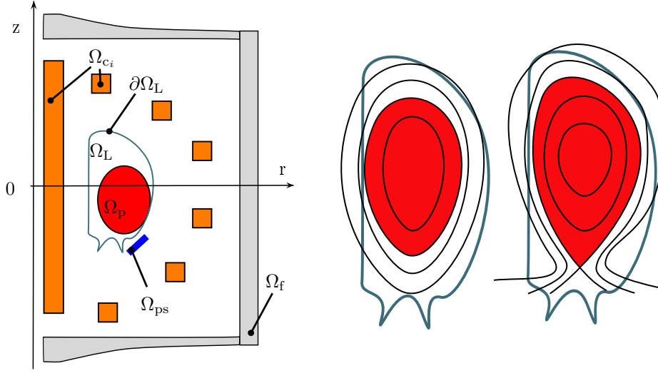
FIGURE 1.1 – Gauche : représentation schématique du plan poloidal d'un tokamak. \Omega_p est le domaine du plasma, \Omega_L est le domaine du limiteur accessible au plasma, \Omega_{c_i} représentent les bobines de champ poloidal, \Omega_{ps} les structures passives et \Omega_f les structures ferromagnétiques. Droite : exemple de plasma dont la frontière est définie par le contact avec le limiteur ou par la présence d'un point X.
