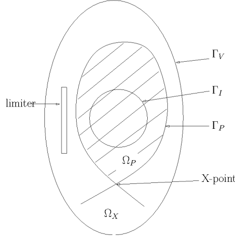
FIGURE 1.4 – Le domaine \Omega_V de frontière \Gamma_V est la réunion du domaine \Omega_X et du domaine plasma \Omega_P dont la frontière \Gamma_P est ici définie par un point-X. \Gamma_I est le contour fictif.
