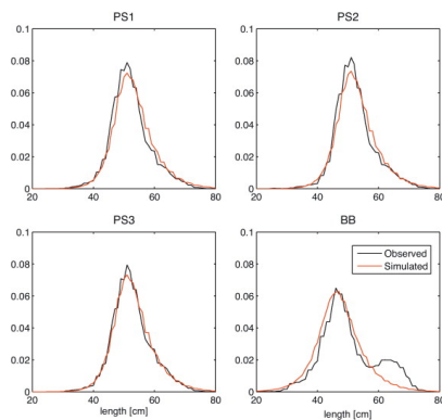
FIGURE 2.5 – Comparaison entre fréquences de tailles simulées et observées pour les 4 flotilles sur la période 1984-1993
