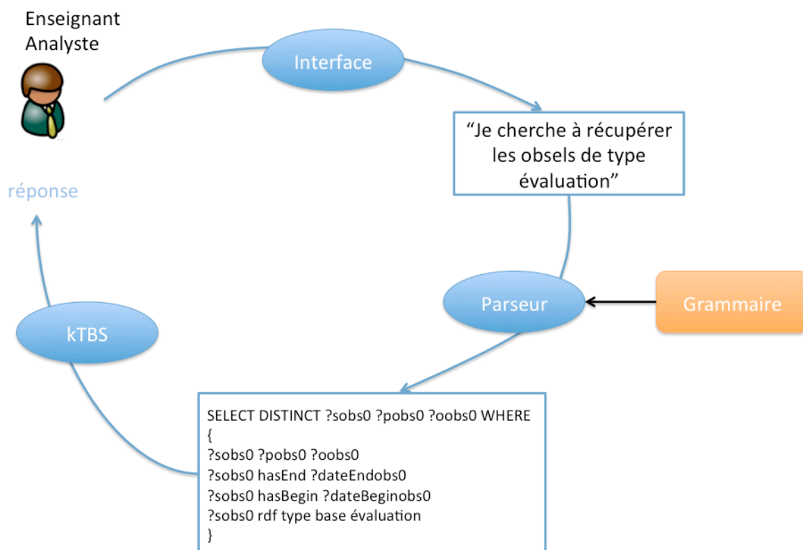
Figure 40. Processus d’interrogation des traces via SPARE-LNC
