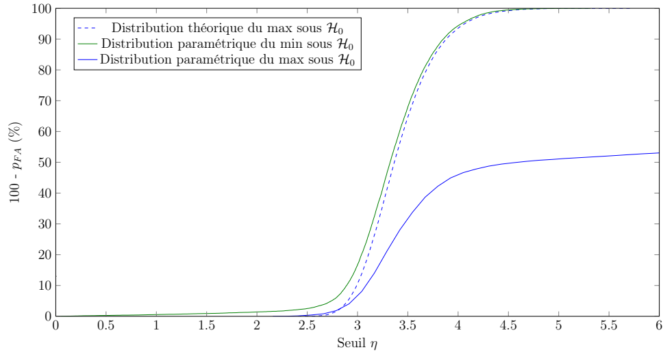
FIGURE 3.14 – Répartition empirique des valeurs maximales et des valeurs minimales calculées sur les spectres d'un cube de données synthétiques contenant des sources. La répartition théorique du max-test sous l'hypothèse nulle est également reportée (courbe en pointillés).
