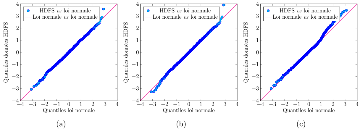
FIGURE 4.5 – Diagrammes quantiles-quantiles des données HDFS avant réduction par le cube de variance (a), après réduction par le cube de variance (b) et après filtrage adapté (c). A noter que dans les trois cas, les données sont centrées-réduites à l'aide des estimateurs de moyenne et de variance de la loi sous l'hypothèse \mathcal{H}_0 obtenus par \sigma -clipping par point fixe afin de comparer à la loi normale.
