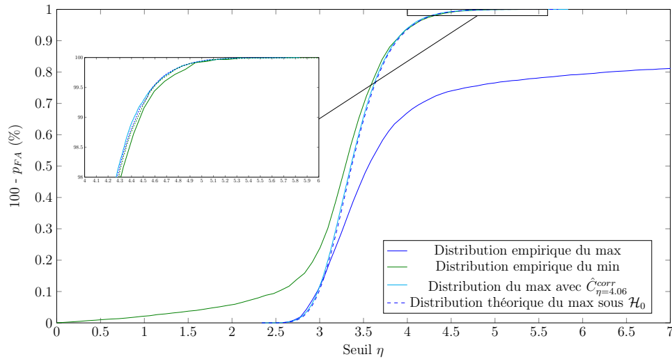
FIGURE 3.21 – Répartition empirique des valeurs maximales et des valeurs minimales calculées sur les spectres du DryRun après filtrage adapté. La répartition théorique du max-test sous l’hypothèse nulle est également reportée (courbe pointillée).
