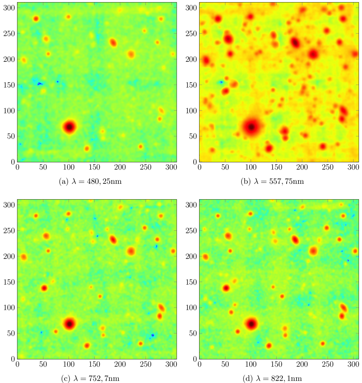
FIGURE 4.3 – Images extraites du cube de données HDF5 à différentes longueurs d’onde après filtrage adapté. L’échelle de couleur varie car la dynamique des images est différente d’une longueur d’onde à l’autre du fait de la corrélation (spatiale et spectrale) du bruit, les données en sortie du filtrage ne sont pas centrées réduites.
