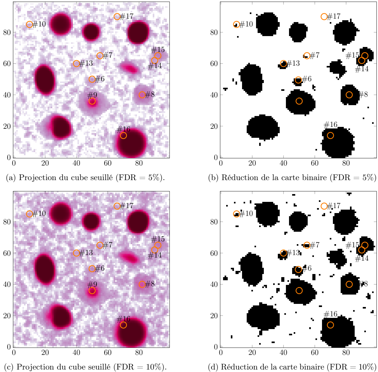
FIGURE 3.24 – Résultats du seuillage du cube DryRun par la procédure de contrôle du FDR par la procédure de Benjamini and Hochberg [1995] dans le cas de test dépendant. Les figures (a) et (c) sont les cartes obtenues en sommant les pixels (binaires) de chaque spectre. Les pixels blancs signifient que tous les pixels du spectre ont été classés dans \mathcal{C}_0 , plus la couleur est foncée, plus le spectre contient de pixels classés sous \mathcal{H}_1 . Les figures (b) et (d) tiennent compte des a priori physique que nous avons sur les galaxies de type Ly \alpha : une raie d'émission a une largeur significative qui est étendue par la LSF lors du filtrage adapté. Tous les spectres qui ne présentent pas plus de 5 éléments consécutifs classés sous \mathcal{H}_1 sont rejetés de la carte de proposition. Les cercles oranges modélisent les galaxies de type Ly \alpha dans les données DryRun.
