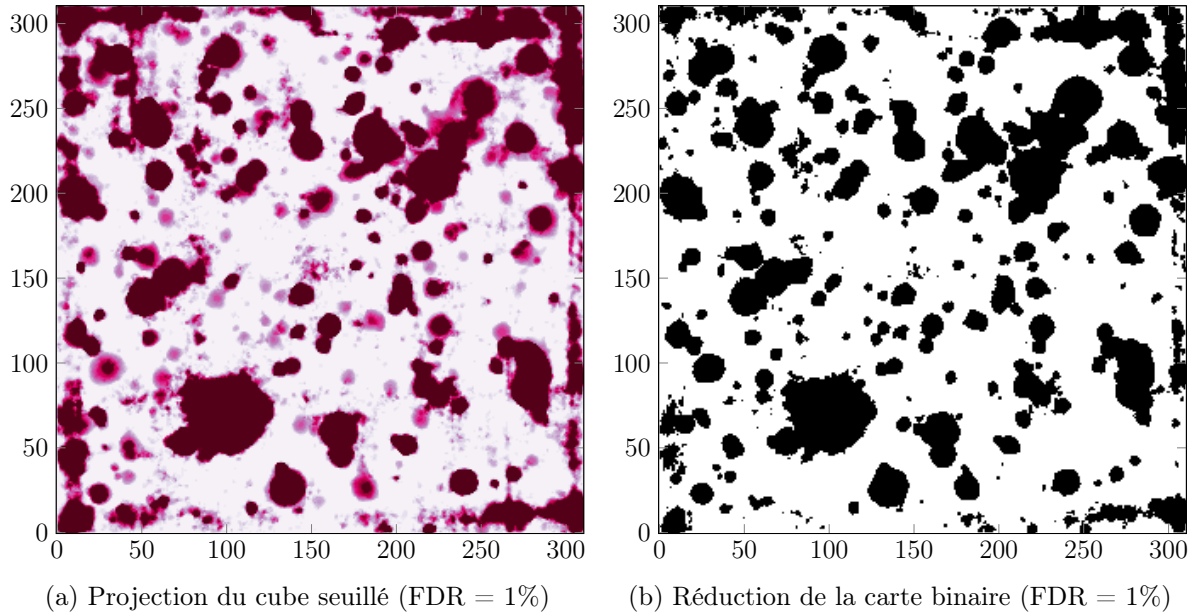
FIGURE 4.11 – Résultats du seuillage du cube HDF5 par la procédure de contrôle du FDR par la procédure de Benjamini and Hochberg [1995] dans le cas de tests dépendants. La figure (a) est la carte obtenue en sommant les pixels (binaires) de chaque spectre. Les pixels blancs signifient que tous les pixels du spectre ont été classés dans \mathcal{C}_0 , plus la couleur est foncée, plus le spectre contient de pixels classés sous \mathcal{H}_1 . La figure (b) tient compte de l'hypothèse que les raies Ly \alpha présentent une certaine largeur spectrale (quelques bandes consécutives avec la résolution de l'instrument MUSE). Tous les spectres qui ne présentent pas plus de 5 éléments consécutifs classés sous \mathcal{H}_1 sont rejetés de la carte de proposition.
