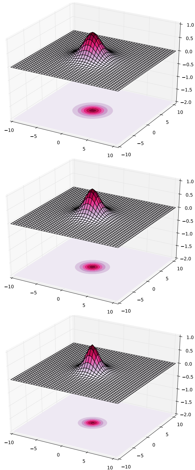
FIGURE 1.15 – Modélisation de la FSF (non normalisée) de MUSE pour le cube HDFS à différentes longueurs d’onde. Haut : \lambda = 480nm ( FWHM_{480} = 0.76 arcsec), centre : \lambda = 700nm ( FWHM_{700} = 0.66 arcsec) et bas : \lambda = 930nm ( FWHM_{930} = 0.55 arcsec).
