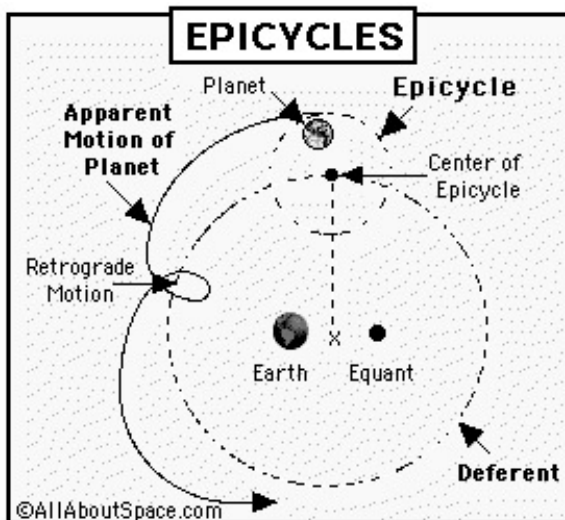
Figure 15 : Modèle ptoléméen de l'Univers
