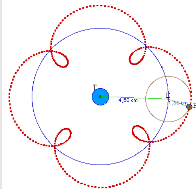
Figure a: Modèle de l'univers géocentrique de Ptolémée: les planètes ne décrivent pas d'orbites simples, mais font des pirouettes (épicycles) censées expliquer leur mouvement rétrograde à certains moments.
