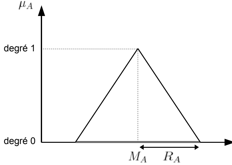
FIG. 1.11: Représentation d'un intervalle flou triangulaire symétrique
