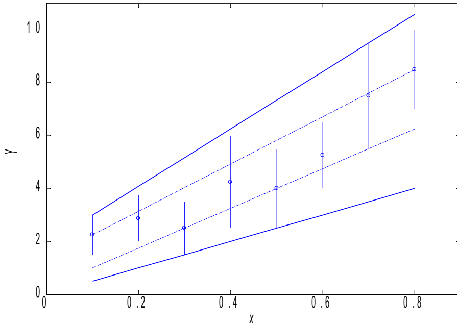
FIG. 2.2: Modèle flou trapézoïdal identifié
