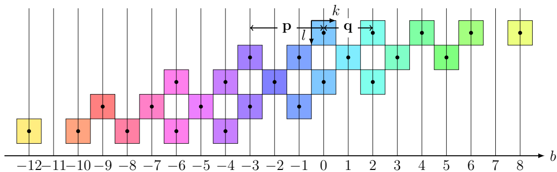
(b) Calcul de la même projection en sur-échantillonnant et en décalant les lignes de l'image
