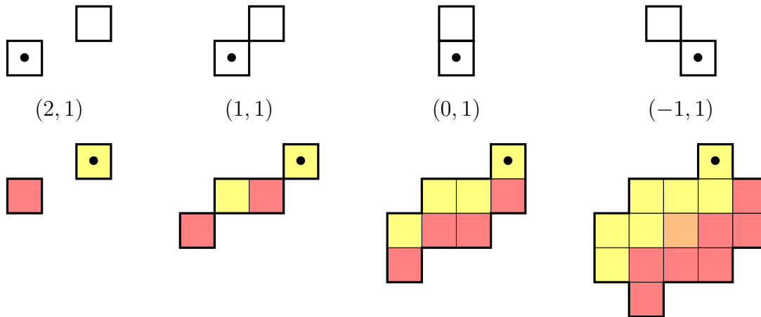
FIGURE 3.27 – Dilatations successives d’un pixel central par les éléments structurants à deux pixels correspondant aux vecteurs (2, 1) , (1, 1) , (0, 1) et (-1, 1) . L’origine du plan discret est représentée par le symbole \bullet . Pour chaque étape, les pixels jaunes correspondent aux pixels pré-existants et les pixels rouges sont créés par la dilatation des pixels jaunes. Les pixels appartenant à la fois à ces deux catégories sont colorés en orange.
