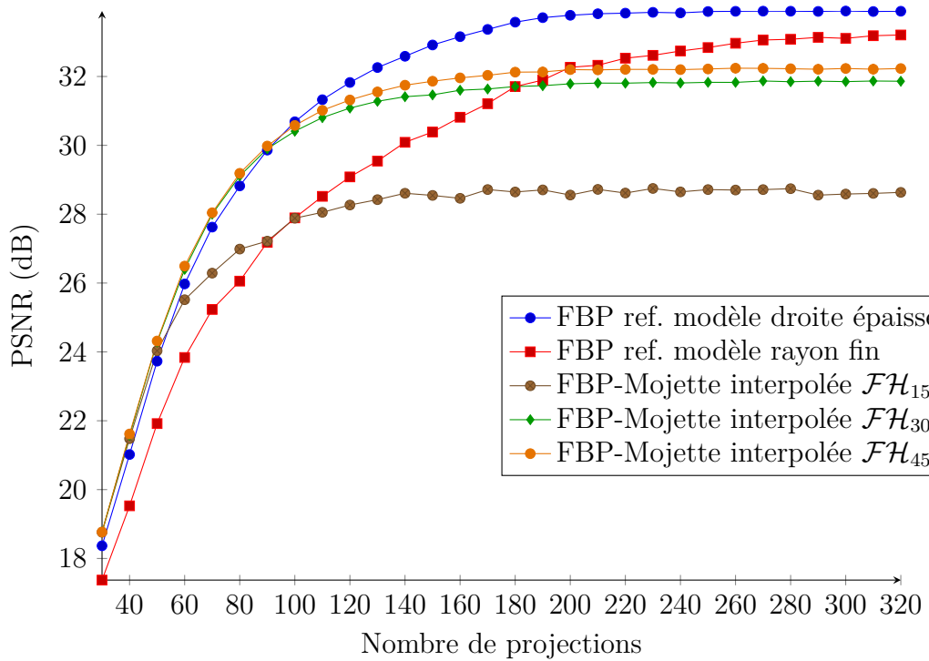
(a) FBP-Mojette
