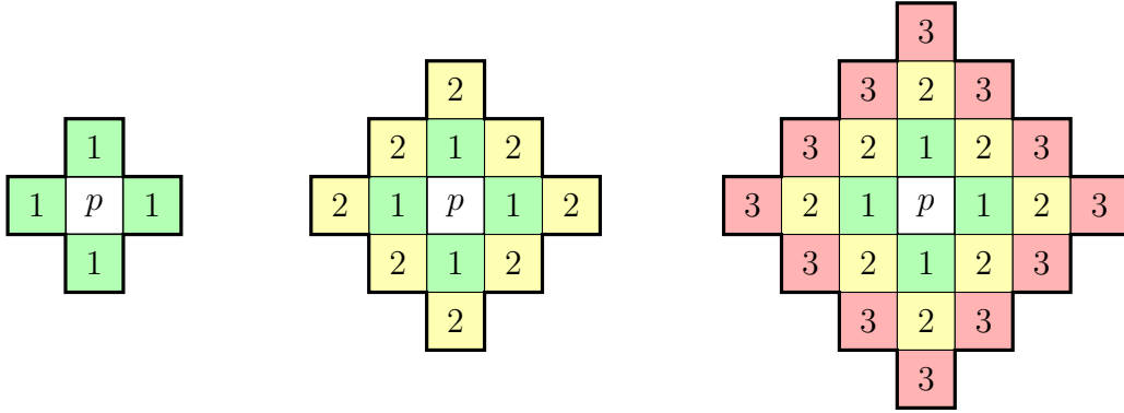
(a) Boules de distances B_{<}(p, r) pour d_1 avec r \in \{1, 2, 3\}
