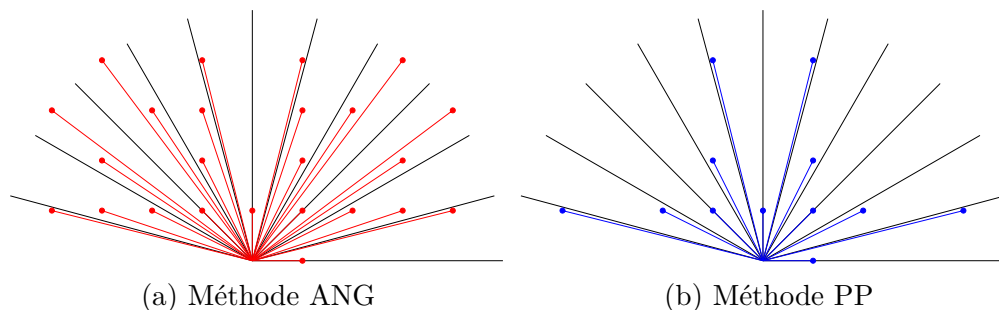
FIGURE 5.2 – Illustration des deux méthodes de ré-échantillonnage proposées. Ici, N_\theta = 12 et on utilise \mathcal{FH}_4 .
