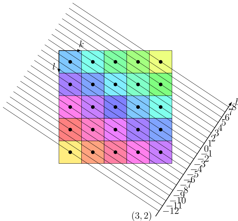
(a) Projection Mojette d'angle (3, 2) d'une image de taille 5 \times 5
