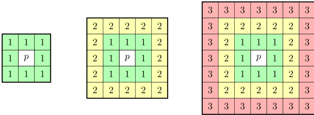
(b) Boules de distances B_{<}(p, r) pour d_2 avec r \in \{1, 2, 3\}
