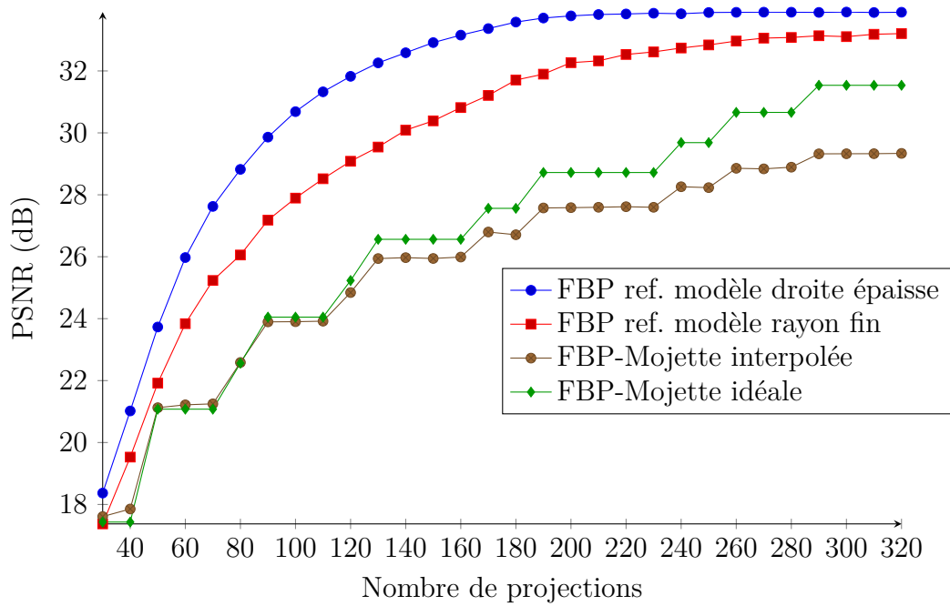
(a) FBP-Mojette
