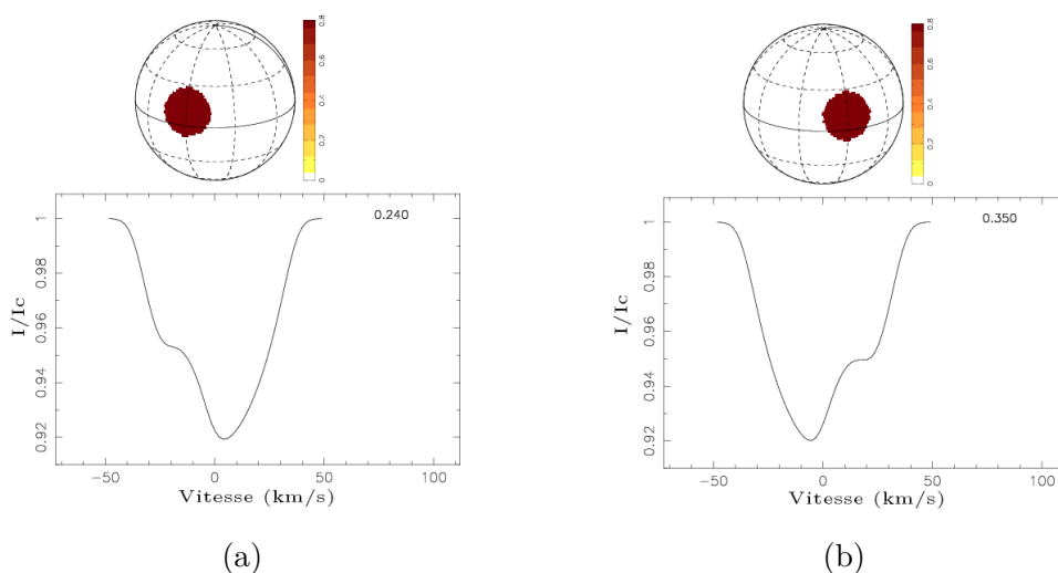
FIGURE 1.5 – Projections par imagerie DOPPLER d'une perturbation sur un astre à différentes étapes de sa rotation, traduite depuis [129]
