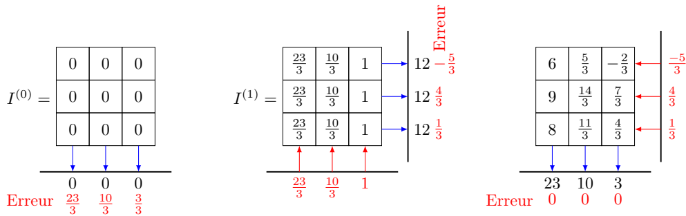
(b) Estimée initiale I^{(0)}
