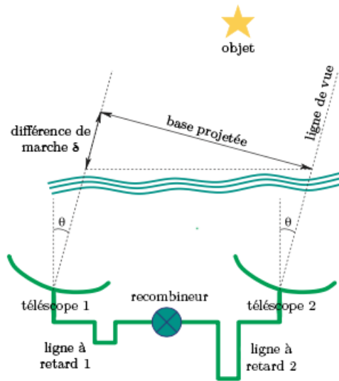
FIGURE 1.7 – Schéma d’un interféromètre stellaire à deux télescopes, traduite depuis [175]
