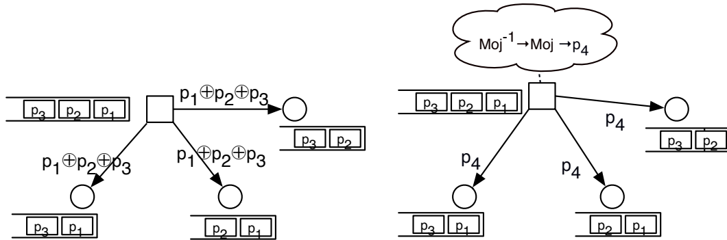
FIGURE 1.13 – Codage basé sur la transformée Mojette pour la transmission sécurisée de paquets sur un réseau, reproduit de [139]
