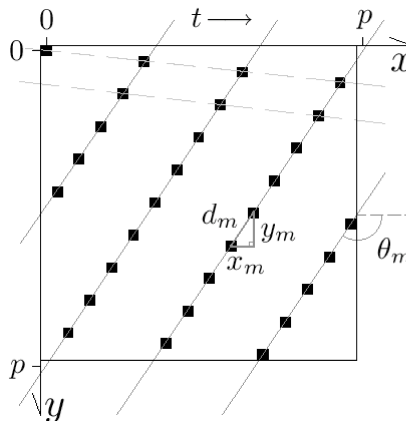
FIGURE 2.20 – Exemple de projection de direction m et l'angle discret (x_m, y_m) correspondant pour la transformée Mojette, tiré de [170]
