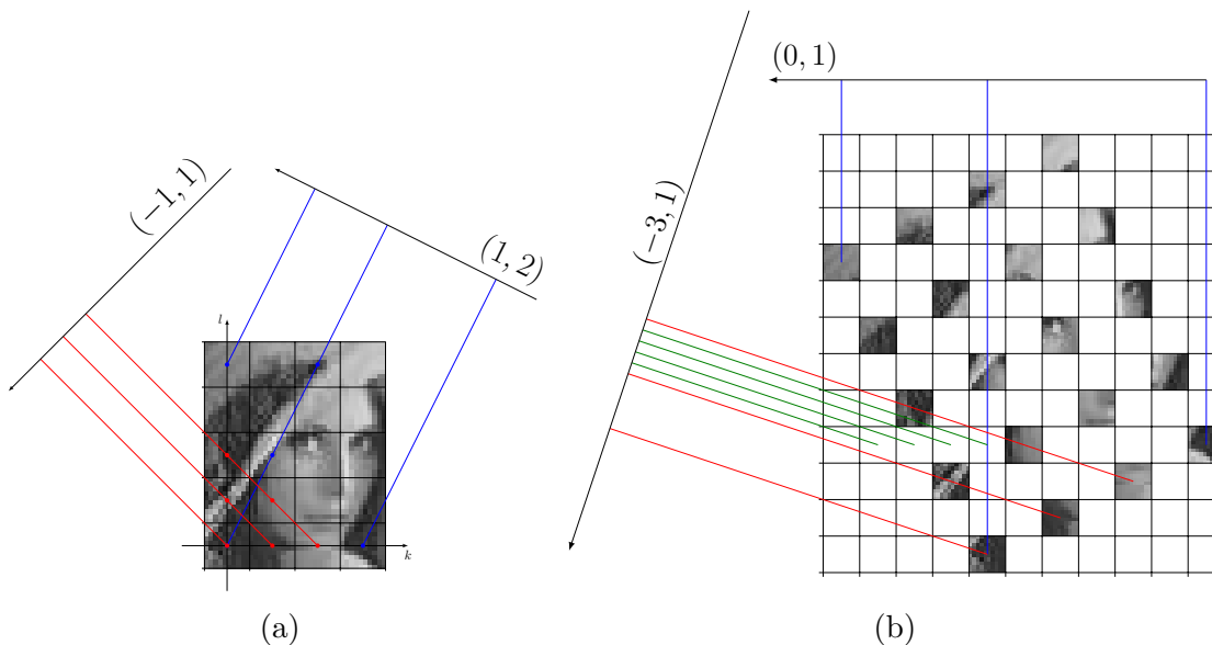
FIGURE 4.4 – (a) Image de 4 \times 5 pixels avec deux projections Mojette de directions (-1, 1) et (1, 2) . (b) Image résultante d'une rotation discrète d'angle (2, 1) de taille 11 \times 12 pixels. Les deux projections Mojette de directions (-1, 1) et (1, 2) deviennent respectivement (-3, 1) et (0, 1) . Dans l'espace Mojette, la rotation entraîne un sur-échantillonnage de certaines projections, représenté par les lignes vertes.
