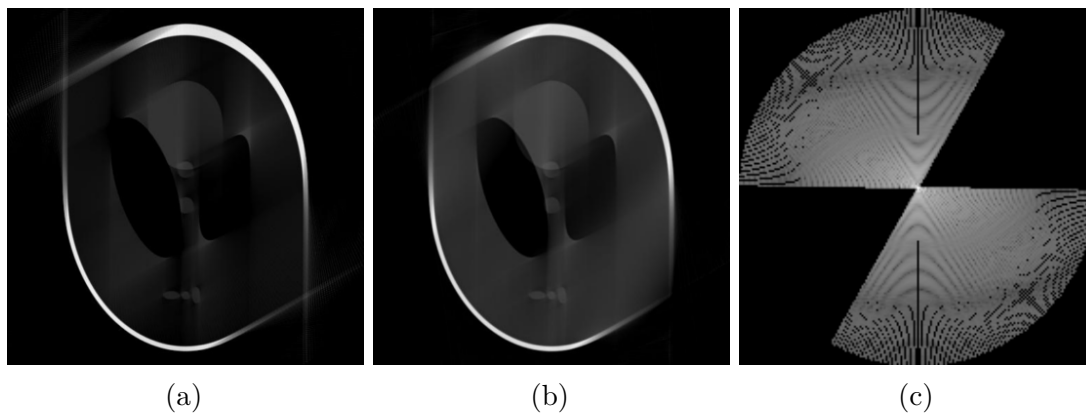
FIGURE 2.14 – Reconstruction à partir du sinogramme incomplet de la figure 2.13b avec (a) Méthode analytique FBP (b) Méthode itérative SART. (c) Espace de FOURIER correspondant à l'image reconstruite par rétroprojection filtrée. Images issues de [146]
