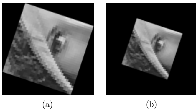
FIGURE 4.9 – (a) Rotation directe dans l'espace Moiré d'angle (1, 3) donnant une 129 \times 129 image. (b) Même résultat obtenu par rotations successives d'angles (2, 1) et (1, 1) , avec une taille d'image finale de 193 \times 193 .
