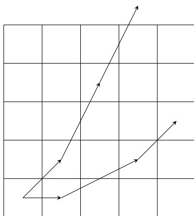
FIGURE 2.23 – Interprétation géométrique du critère de KATZ, tiré de [86]
