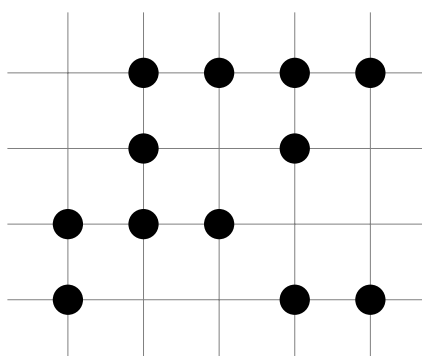
FIGURE 2.18 – Matrice binaire (a) et ensemble fini du plan discret correspondant (b)
