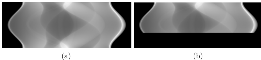
FIGURE 2.13 – Sinogrammes du fantôme de L. A. SHEPP et B. F. LOGAN (a) Sur [0, 180^\circ[ (b) Sur [0, 120^\circ[ .
