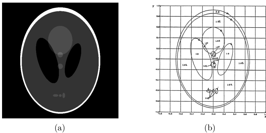
FIGURE 2.12 – Fantôme de L. A. SHEPP et B. F. LOGAN : (a) Image numérique du fantôme (b) Définition analytique [163]
