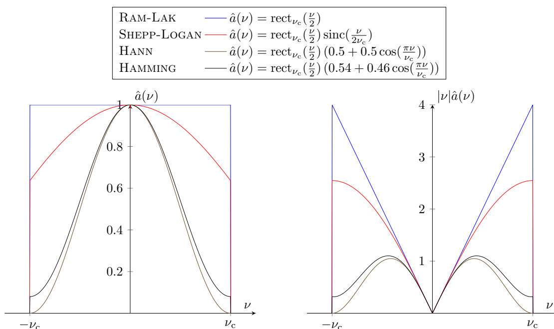
FIGURE 2.11 – Fenêtres d’apodisation (à gauche) et filtres de reconstruction correspondants (à droite)
