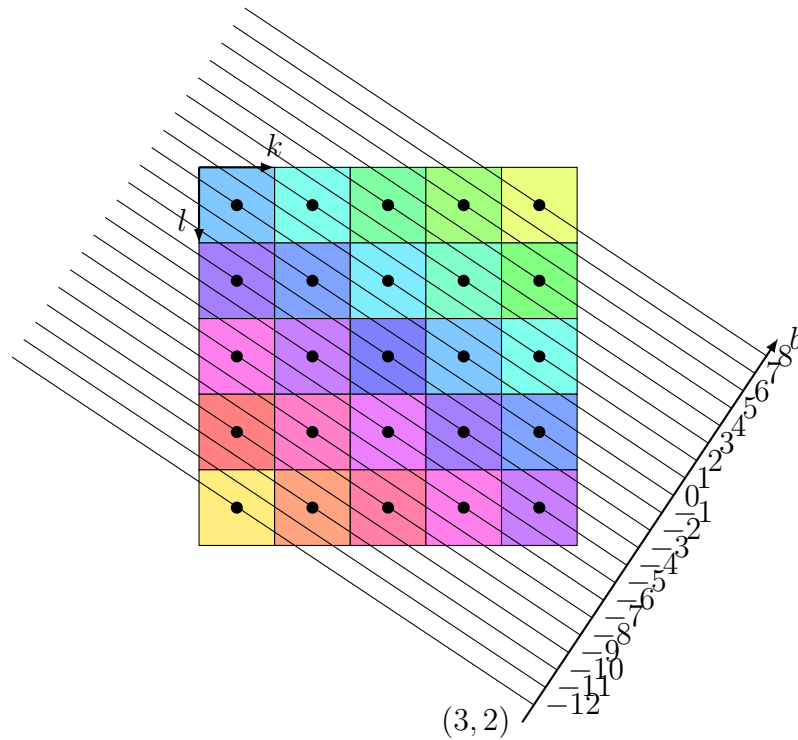
(a) Projection Mojette d'angle (3, 2) d'une image de taille 5 \times 5
