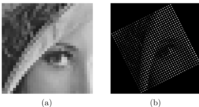
FIGURE 4.5 – (a) Image originale de taille 32 \times 32 . (b) Rotation dans l'espace Mojette d'angle (2, 1)
