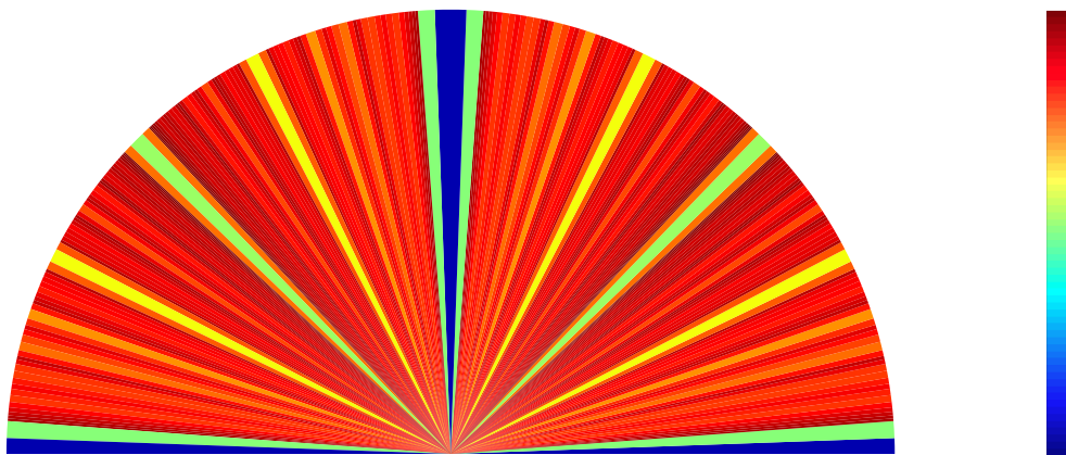
FIGURE 5.13 – Écart angulaire entre chaque direction discrète de projection dans \mathcal{FH}_{14}
