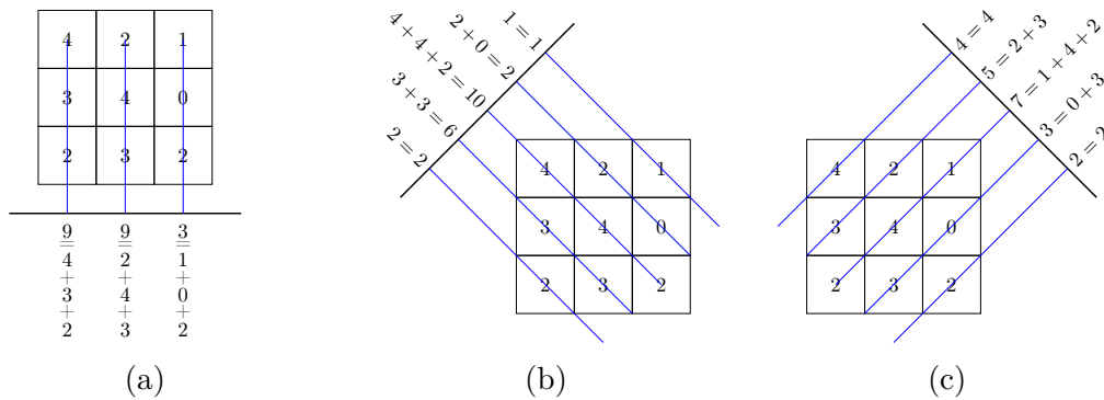
FIGURE 1.15 – Obtention des projections discrètes d'une image de taille 3 × 3
