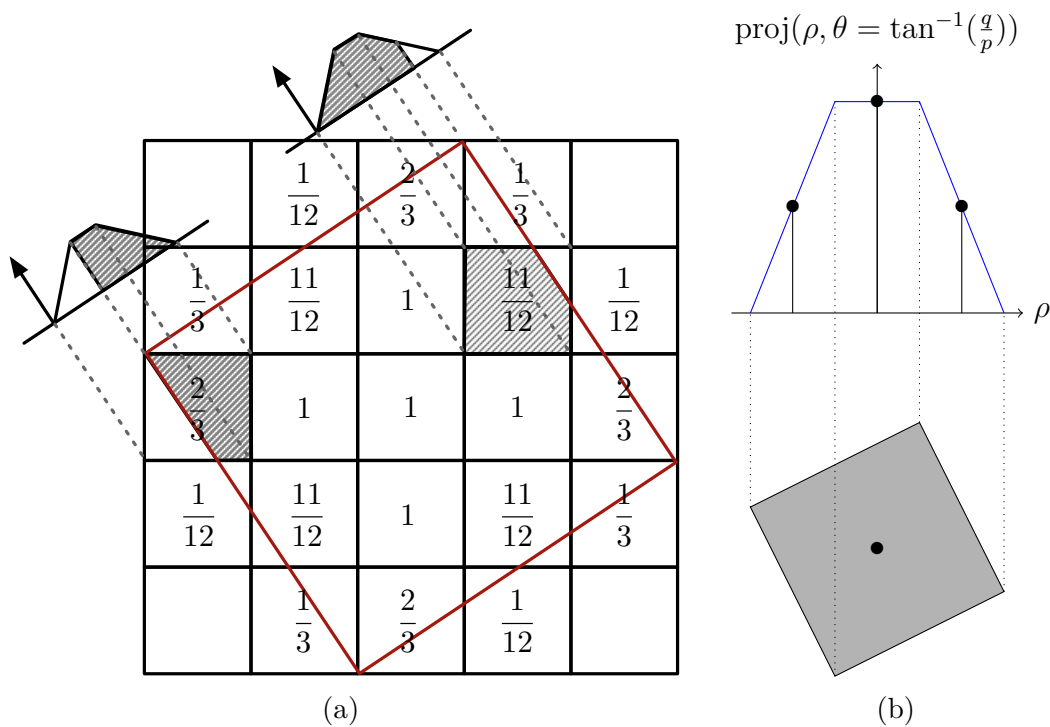
FIGURE 4.7 – (a) L'aire commune entre le pixel transformé et les pixels du pavage initial est égale à l'aire sous la courbe du trapèze délimitée par les droites de directions (p_\vartheta, q_\vartheta) et (-q_\vartheta, p_\vartheta) . (b) Trapèze issu de la projection continue d'un pixel dans la direction (2, 1)
