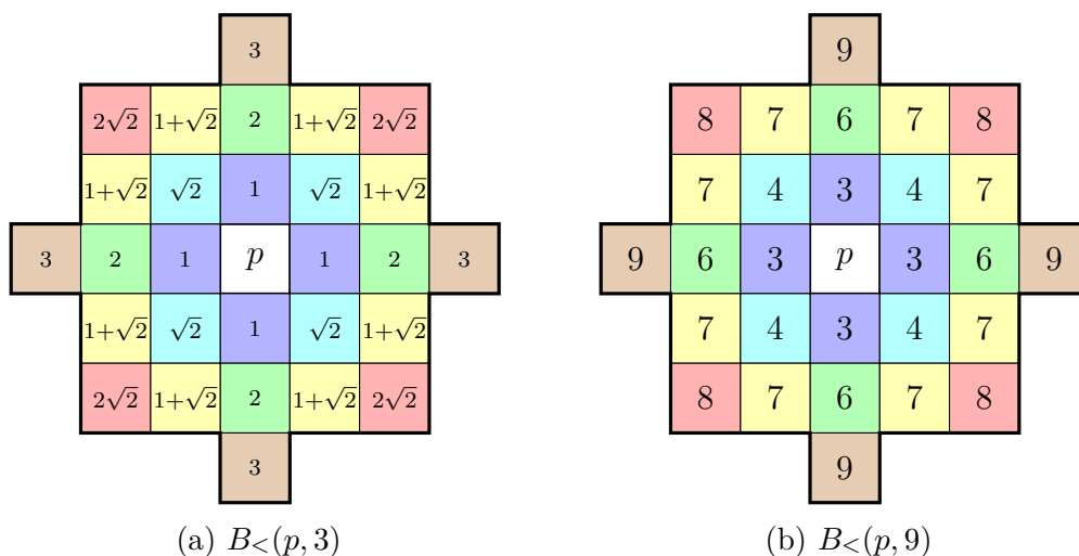
FIGURE 3.11 – Boules de distances pour (a) d_{1,\sqrt{2}} et (b) d_{3,4}
