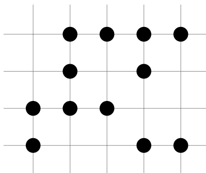
FIGURE 2.18 – Matrice binaire (a) et ensemble fini du plan discret correspondant (b)
