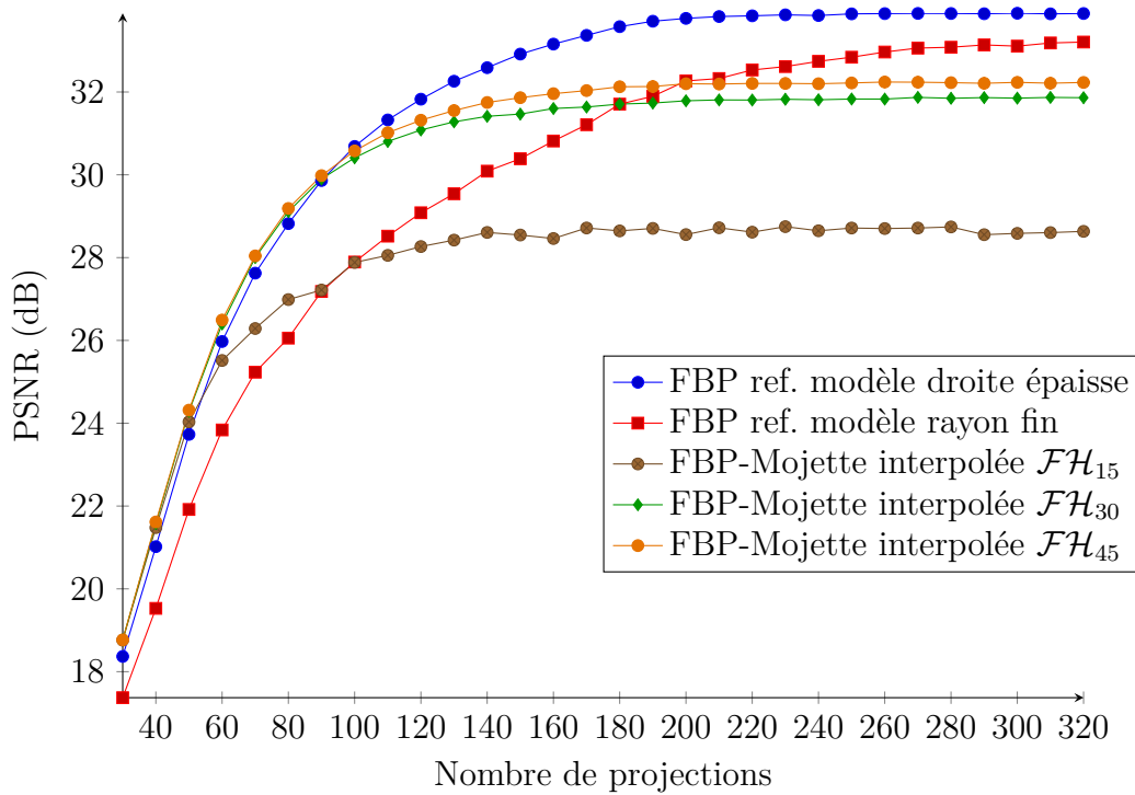
(a) FBP-Mojette
