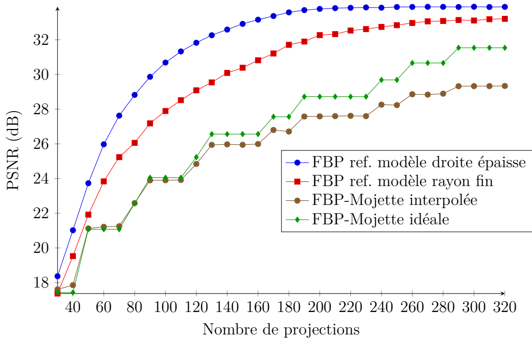
(a) FBP-Mojette
