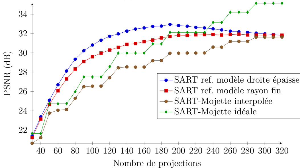
(b) SART-Mojette
