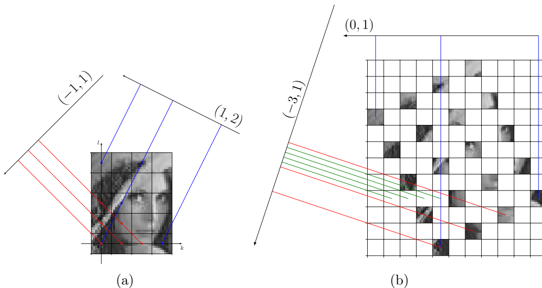
FIGURE 4.4 – (a) Image de 4 \times 5 pixels avec deux projections Mojetta de directions (-1, 1) et (1, 2) . (b) Image résultante d'une rotation discrète d'angle (2, 1) de taille 11 \times 12 pixels. Les deux projections Mojetta de directions (-1, 1) et (1, 2) deviennent respectivement (-3, 1) et (0, 1) . Dans l'espace Mojetta, la rotation entraîne un sur-échantillonnage de certaines projections, représenté par les lignes vertes.
