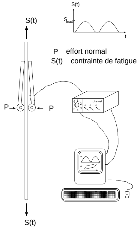
Figure 4.2: Schéma du montage expérimental du fretting-fatigue (Petiot)
