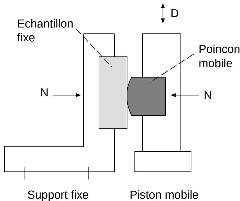
Figure 4.1: Schéma du montage expérimental du fretting
