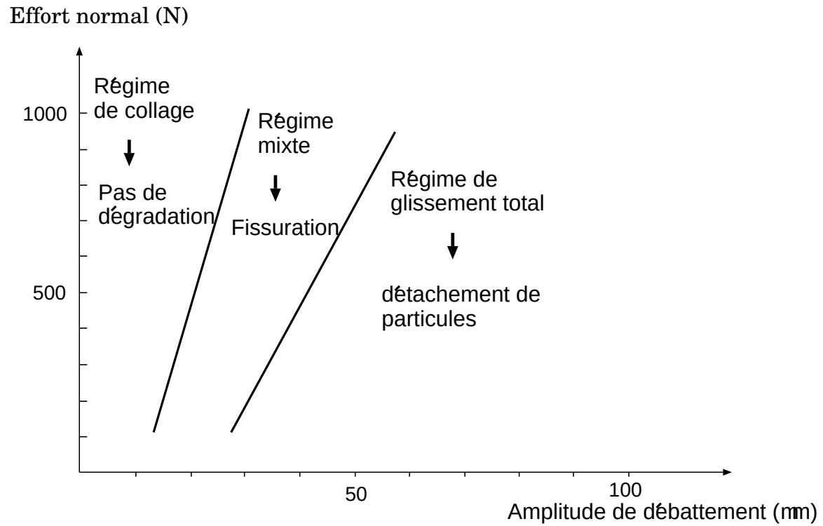
Figure 4.4: Carte de sollicitation et de réponse du matériau, d'après Zhou (1992)
