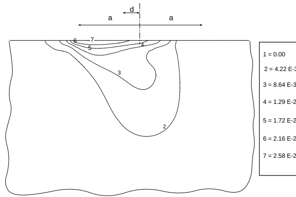
Figure 4.12: Isovaleurs des déformations plastiques équivalentes en régime de glissement total en fretting-fatigue P = 80\text{ N} , S_{max} = 500\text{ MPa}
