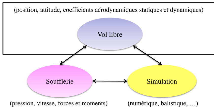
Figure 1: Différentes possibilités pour quantifier les coefficients aérodynamiques
