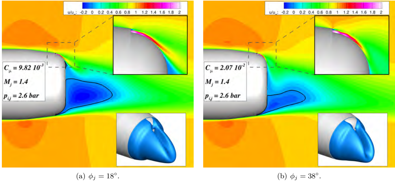
FIGURE 3.26 – Contours de la vitesse adimensionnée u/u_\infty pour les deux étendues azimutales considérées. Les conditions extérieures vérifient M_\infty = 0,7 et \alpha = 3^\circ et le soufflage est tel que M_j = 1,4 et p_{i,j} = 2,6 \text{ bar} . La surface représentée en bas à droite de chaque figure est une iso-surface de vitesse longitudinale nulle permettant de visualiser l’aire sur laquelle le jet attache.
