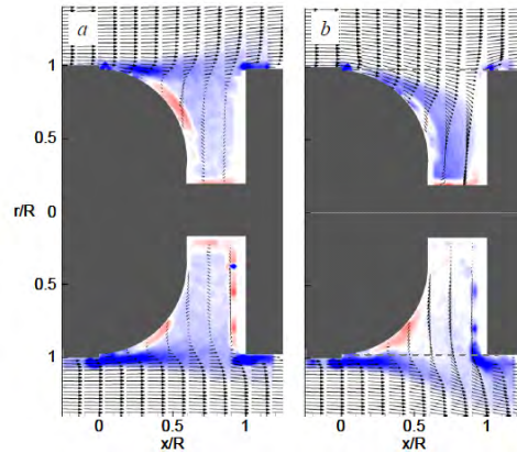
FIGURE 1.25 – Visualisation du champ de vitesses (vecteurs) et du champ de vorticit  (contours) par PIV.   gauche : sans contr le,   droite : avec contr le, d'apr s Abramson et al. [57].
