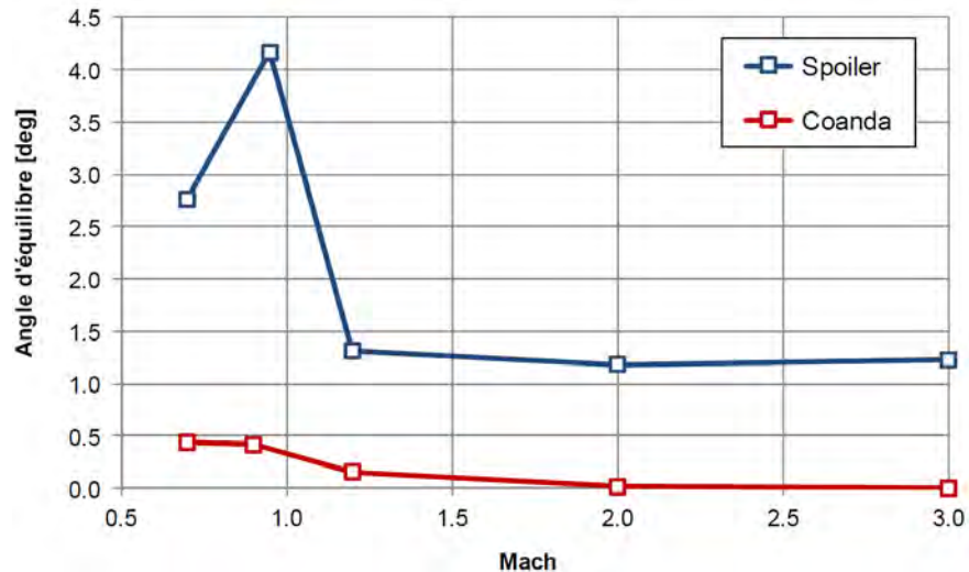
FIGURE 5.8 – Évolution de l'angle d'équilibre en fonction du nombre de Mach du projectile à incidence nulle et pour les deux dispositifs de contrôle considérés, d'après Wey et Martinez [224].
