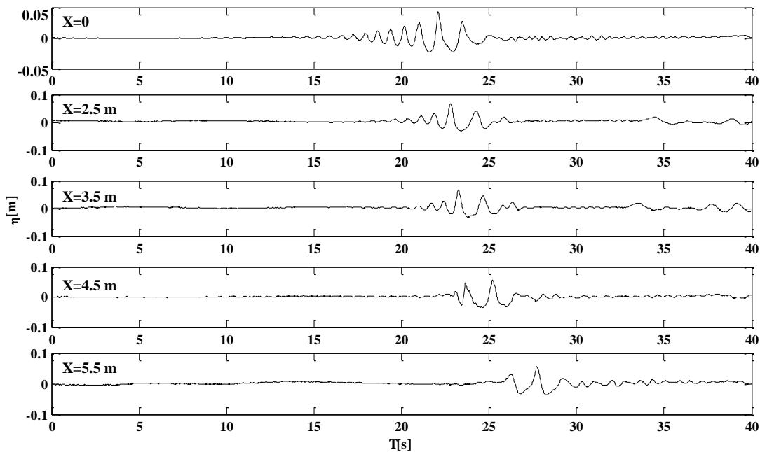
Figure III.3 : Evolution de la surface libre avec un courant dans le sens des ondes avec f=0,75 Hz à différentes positions le long du canal.
