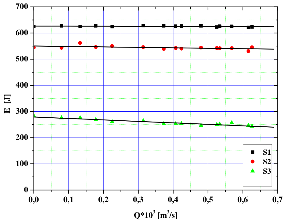
Figure IV.5 : Energie du paquet d'ondes en présence d'un rideau de bulles d'air artificiel à différentes positions le long du canal, Merkoune et al [2011].
