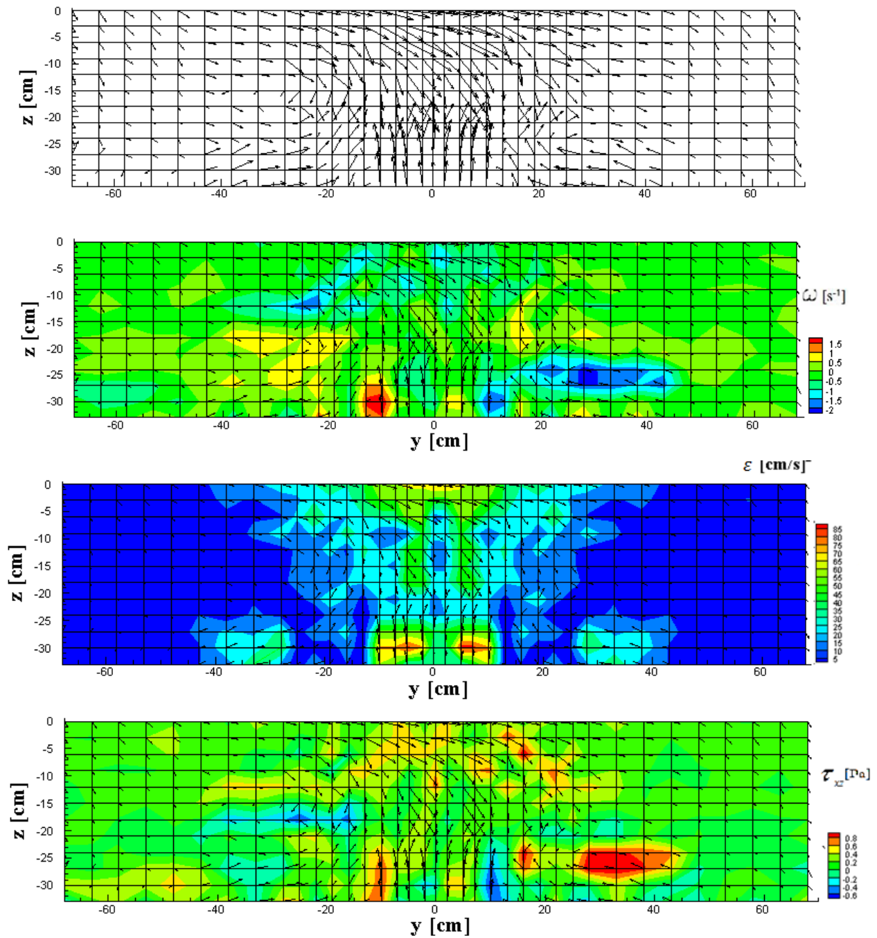
Figure IV.23: Caractéristiques d'écoulement (a) : champs de vitesse, (b) : vorticité, (c) : densité énergétique, (d) : taux de cisaillement pour un débit d'air Q=0,8 \cdot 10^{-3} \text{ m}^3/\text{s} à t_4 .
