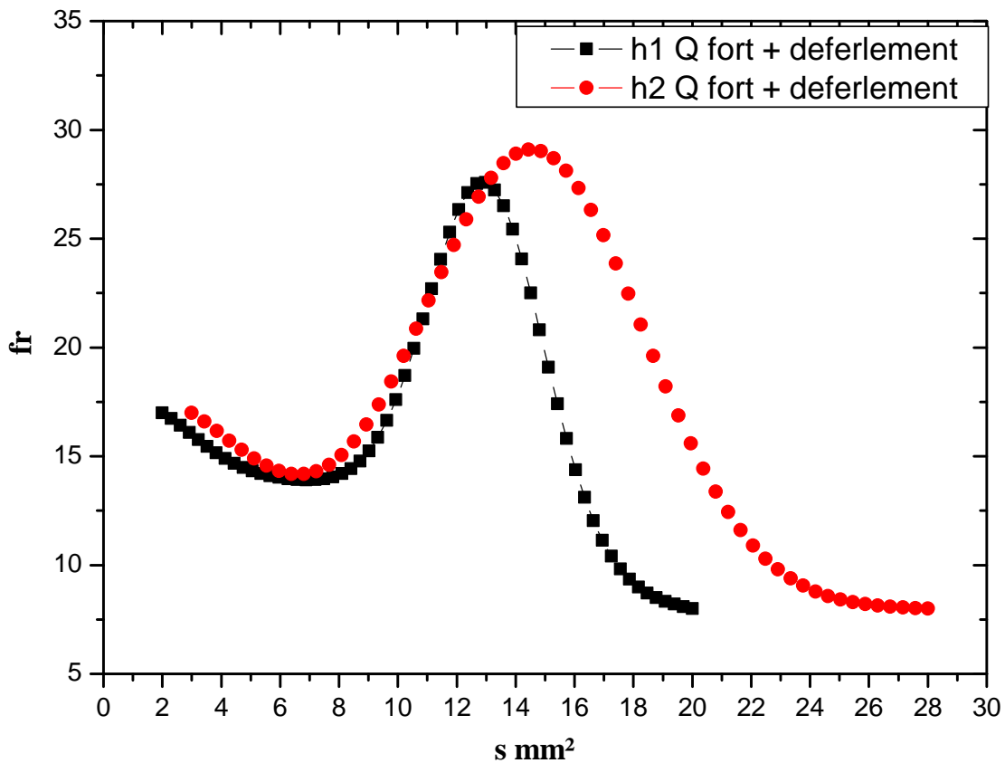
Figure II.15 : Distribution de la surface des bulles dans une gamme de hauteur définie, h1 \in z[5cm, 25cm] et h2 \in z[25cm, 45cm] .
