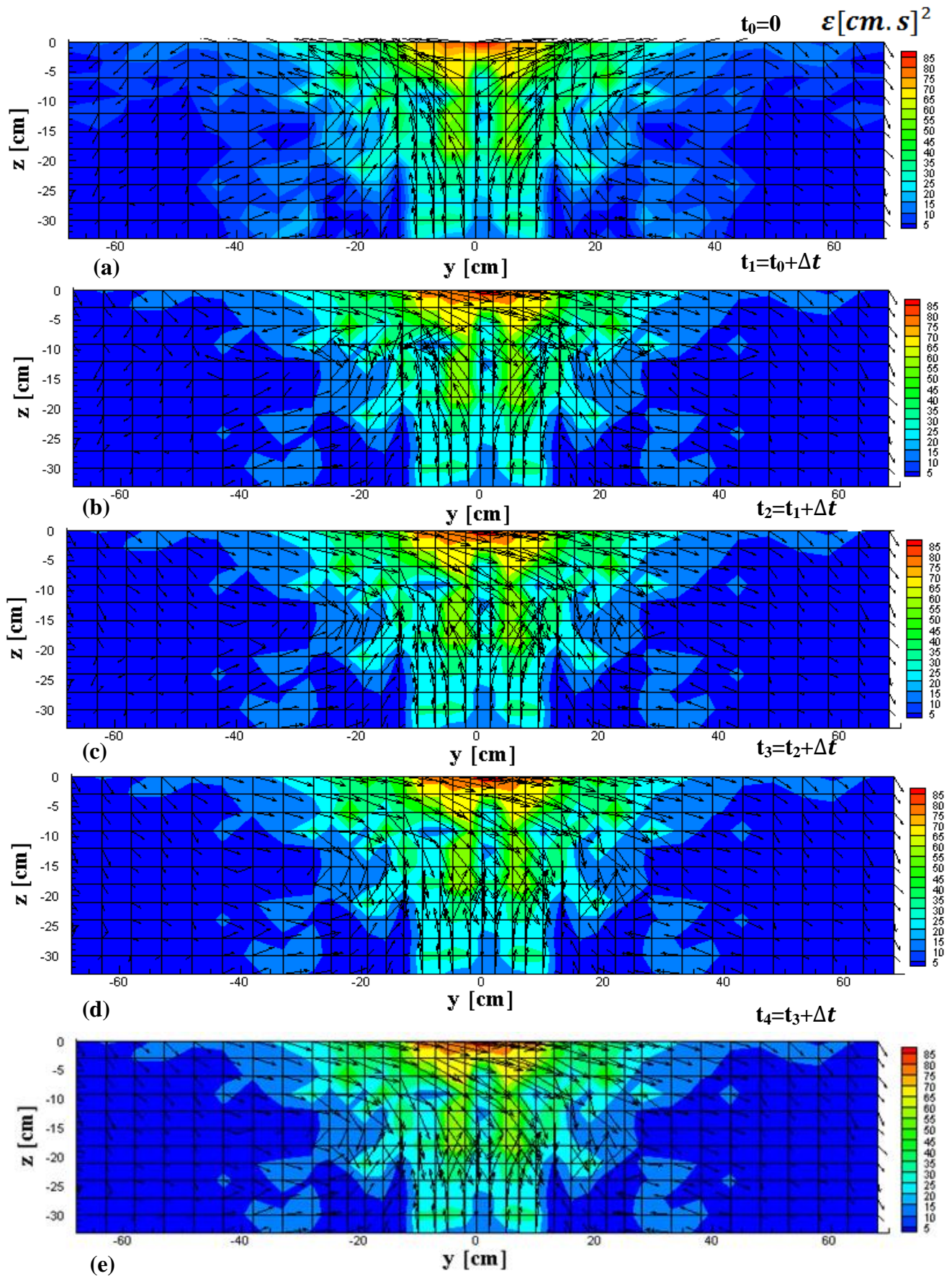
Figure IV.18: Evolution spatio-temporelle de la densité énergétique pour un débit d'air Q=1,2 \cdot 10^{-3} \text{ m}^3/\text{s} pendant 1s.
