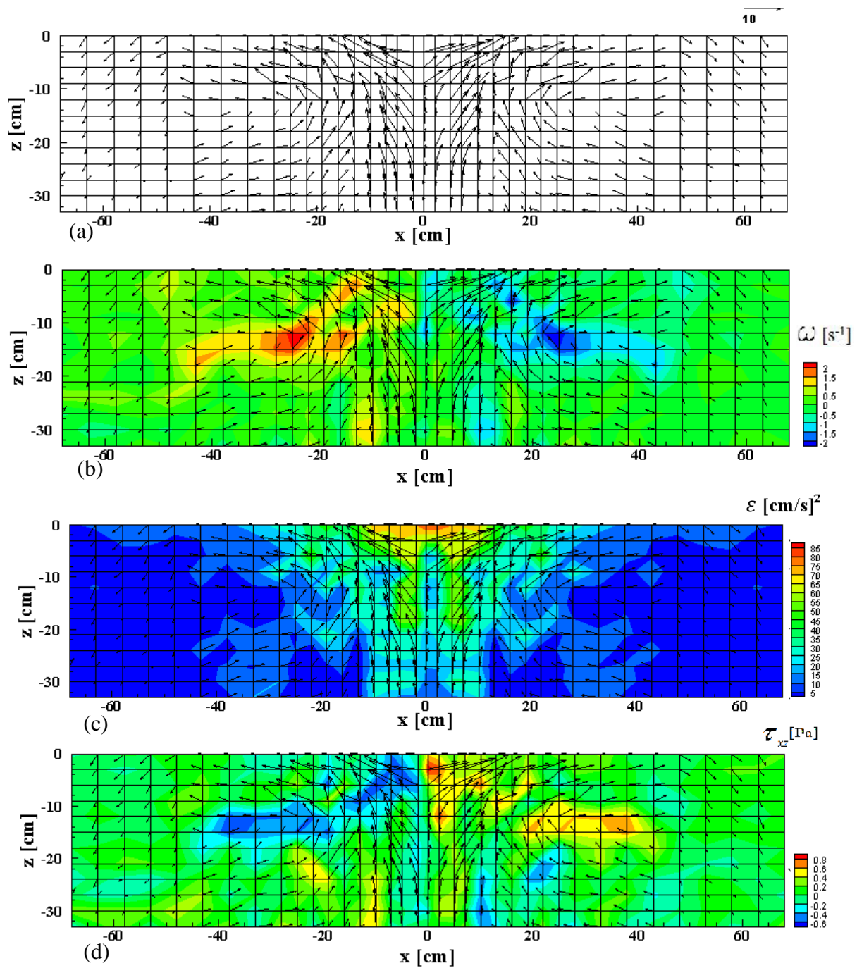
Figure IV.22 : Caractéristiques d'écoulement (a) : champs de vitesse, (b) : vorticité, (c) : densité énergétique, (d) : taux de cisaillement pour un débit d'air Q=0,8 \cdot 10^{-3} m^3/s à t_0 .
