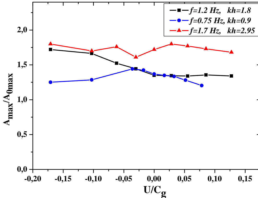
Figure III.8 : Evolution de la hauteur de focalisation pour f=1,7 Hz, f=1,2 Hz et f=0,75 Hz, Merkoune et al [2013].
