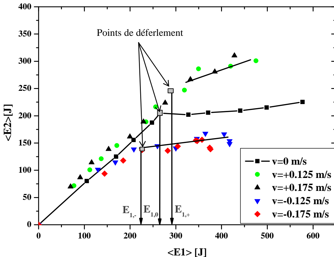
Figure III.4 : Evolution du flux énergétique en présence d'un courant pour les deux sens d'écoulement, Merkoune et al [2013].
