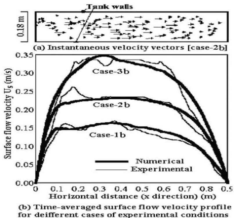
Figure I.20 : Comparaison entre les résultats numériques et expérimentaux pour des profils de vitesses d'écoulement moyen à la surface libre (Abdulmouti [2011]).
