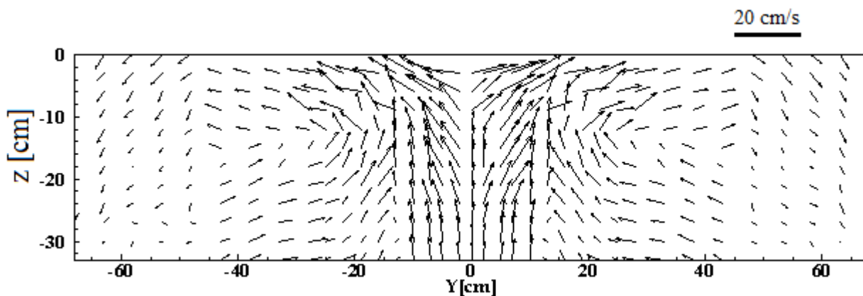
Figure II.24 : Cartographie du champ de vitesse pour un d bit d'air Q=1.2 \cdot 10^{-3} \text{ m}^3/\text{s} .
