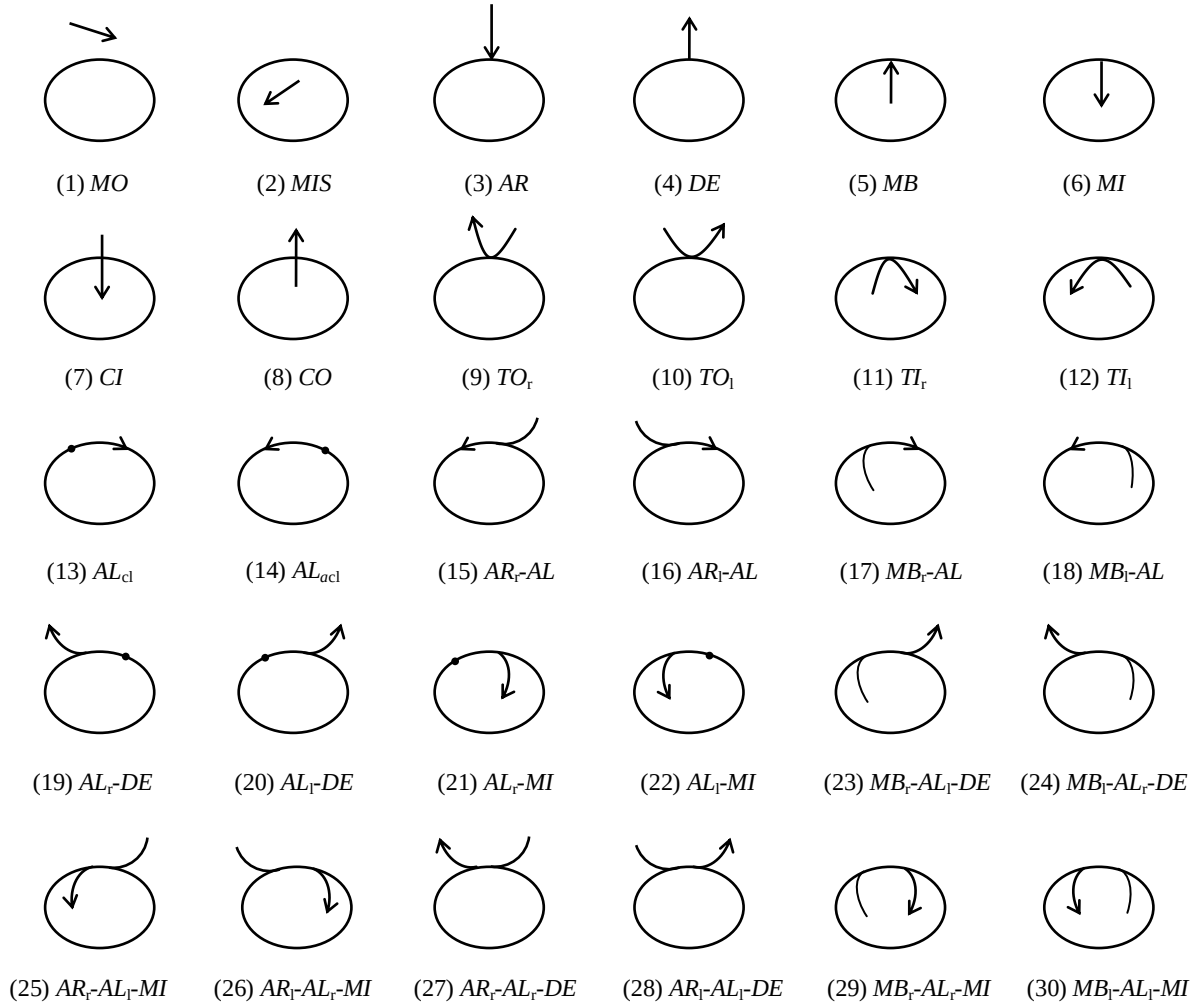
Figure A.1. Mouvements élémentaires entre une ligne orientée et une région
