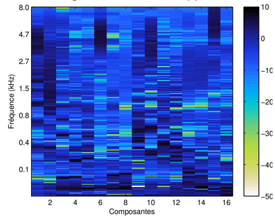
(c) Dictionnaire \tilde{\mathbf{W}}_2 appris par NMF sur le bruit seul.
