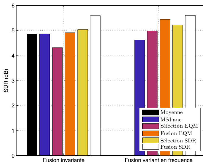
FIGURE 4.1 – Performance de fusion statique en moyenne, de fusion statique invariante et de fusion statique variant en fréquence, pour le rehaussement de la parole. Dans les barres relatives à la fusion variant en fréquence, la fusion par moyenne n'apparaît pas puisqu'elle est équivalente à la fusion invariante par moyenne.
