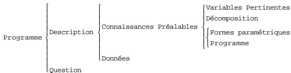
Figure 2.5 : Structure d'un programme bayésien
