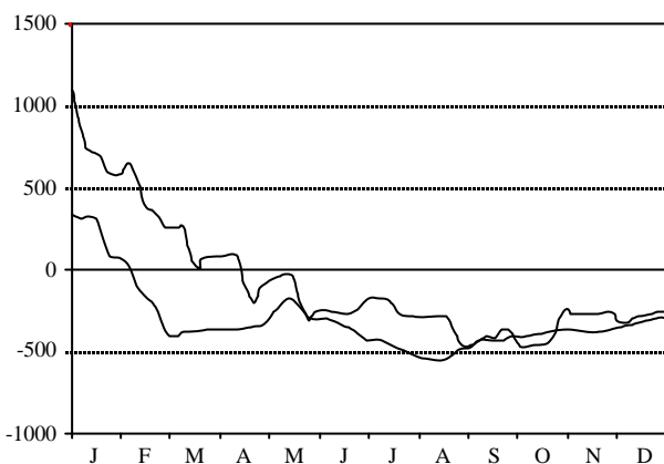
Figure 5.13 - Dynamique des matières en suspension (MES) (—, flux en g.m -3 ; —, budget en kg)
