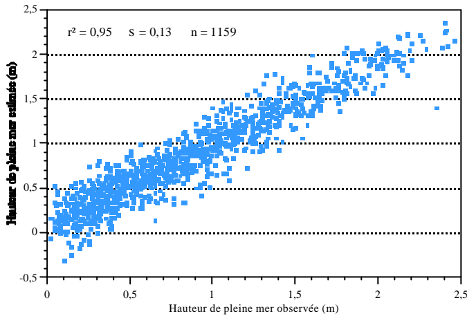
Figure 7.2 - Hauteurs de pleine mer observées et estimées
