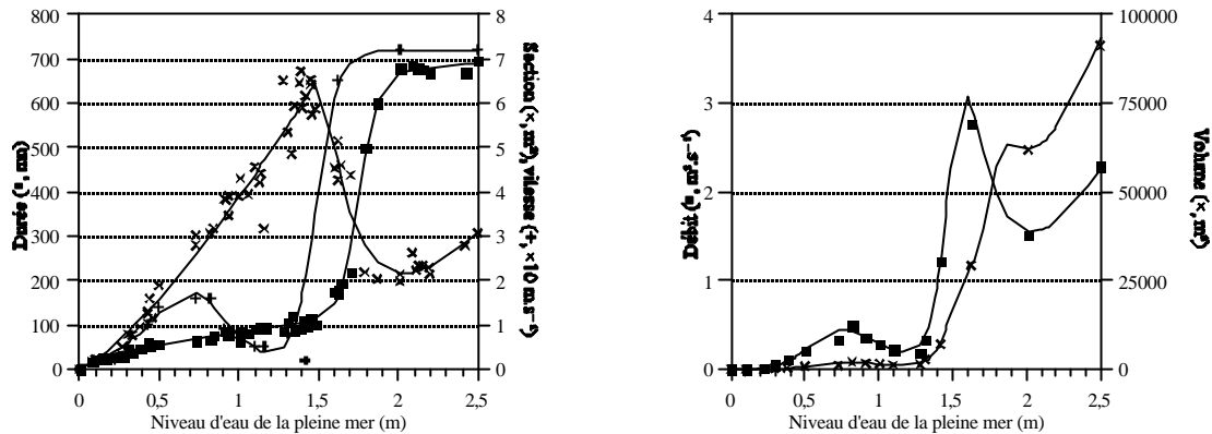
Figure 4.2 - Courbes de calibration du jusant (les courbes traduisent les équations mentionnées, les points, les valeurs réellement observées)
