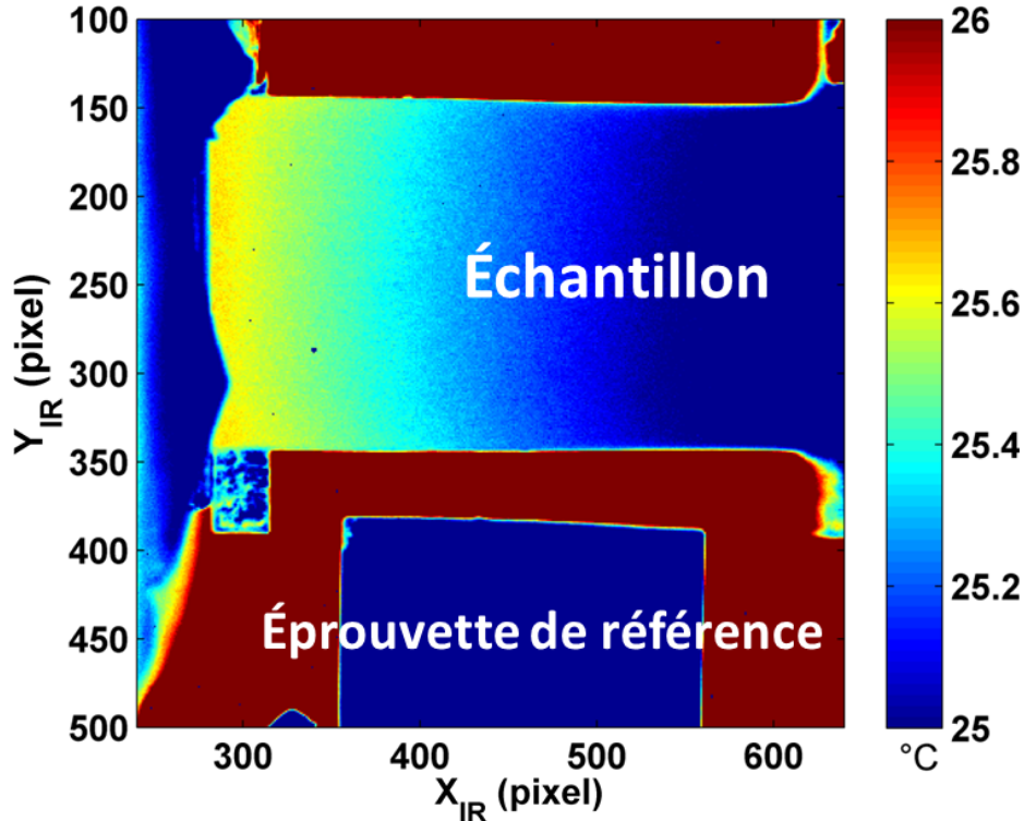
FIGURE 3.6 – Éprouvette sollicitée et éprouvette de référence
