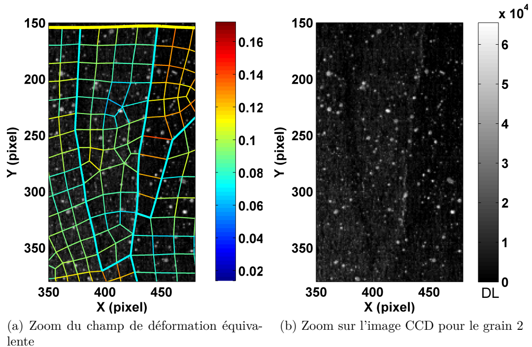
FIGURE 6.17 – Zoom sur le champ de déformation équivalent pour le grain 2 à l’instant C ainsi que l’image visible correspondante
