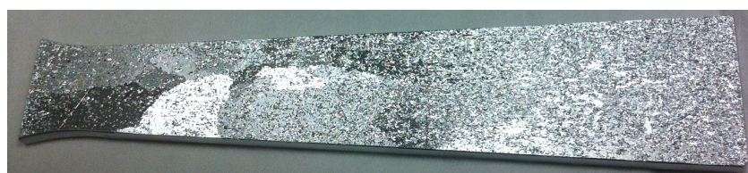
(a) Pré-écrouissage d’environ 2% au milieu de l’éprouvette Trap 2
