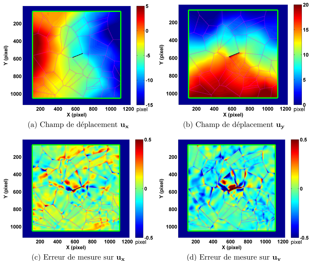
FIGURE 4.20 – Traitement Cinématique III-F : Champs de déplacements \mathbf{u}_x et \mathbf{u}_y obtenus par CIN-E ainsi que l'erreur de mesure par rapport au champ de déplacements simulé \mathbf{u}_x^{\text{Aster}} et \mathbf{u}_y^{\text{Aster}}
