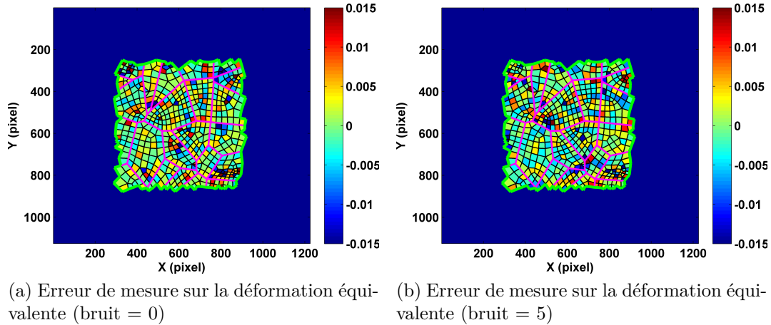
FIGURE 4.35 – Erreur de mesure sur la déformation équivalente pour le traitement Micro-élément-exact aux niveaux de bruit 0 et 5
