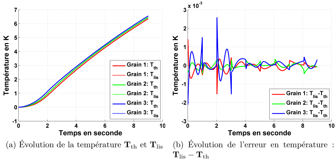
FIGURE 5.23 – Traitement Thermique III : Évolution temporelle de la température moyennée par grain, \mathbf{T}_{th} et \mathbf{T}_{lis} , ainsi que leurs différences pour les grains 1, 2 et 3
