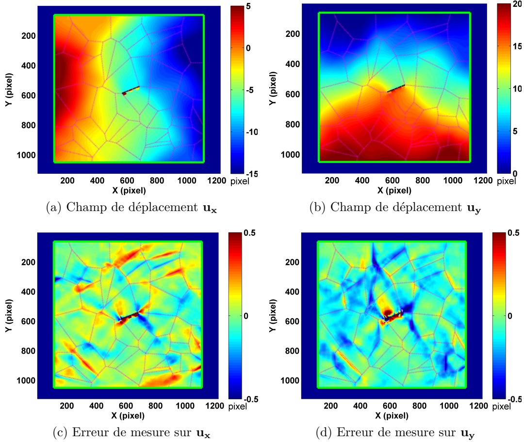
FIGURE 4.24 – Traitement Cinématique IV-F (Cas 2) : Champs de déplacements \mathbf{u}_x et \mathbf{u}_y obtenus par CIN-E ainsi que l’erreur de mesure par rapport au champ de déplacements simulé \mathbf{u}_x^{\text{Aster}} et \mathbf{u}_y^{\text{Aster}}
