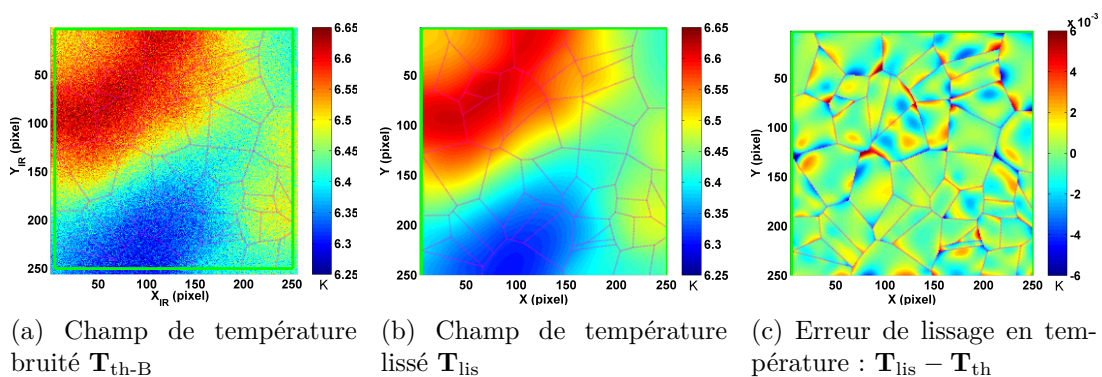
FIGURE 5.13 – Traitement Thermique II : Champ de température obtenu par le traitement d'image thermique ( \mathbf{T}_{\text{lis}} ) à partir de l'image bruitée ( \mathbf{T}_{\text{th-B}} ) ainsi que la différence par rapport au champ de température théorique ( \mathbf{T}_{\text{th}} )
