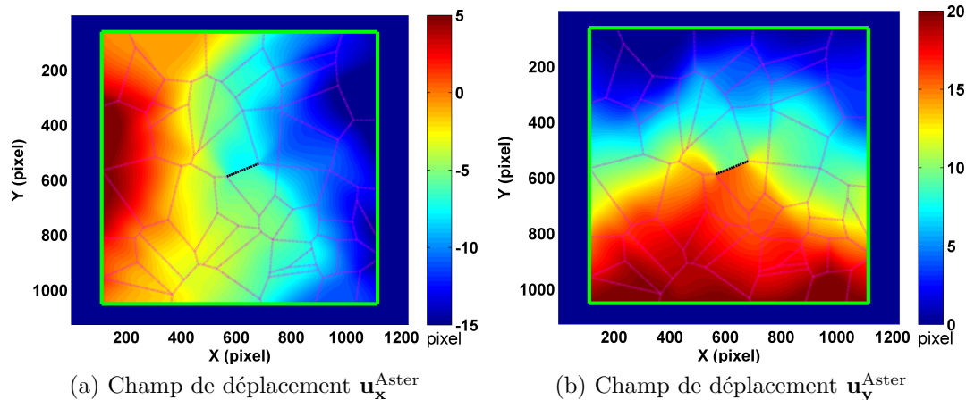
FIGURE 4.5 – Champs de déplacements obtenus par la simulation numérique pour la microstructure fissurée dans les directions \vec{X} et \vec{Y}
