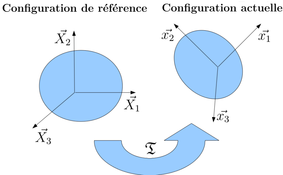
FIGURE 1.1 – Configuration Lagrangienne et Eulérienne
