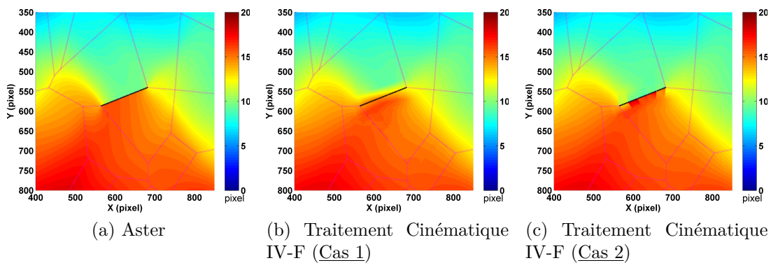
FIGURE 4.25 – Zoom du champ \mathbf{u}_y sur la zone de fissure pour le Cas 1 et Cas 2 du Traitement Cinématique IV-F ainsi que le résultat donné par Aster
