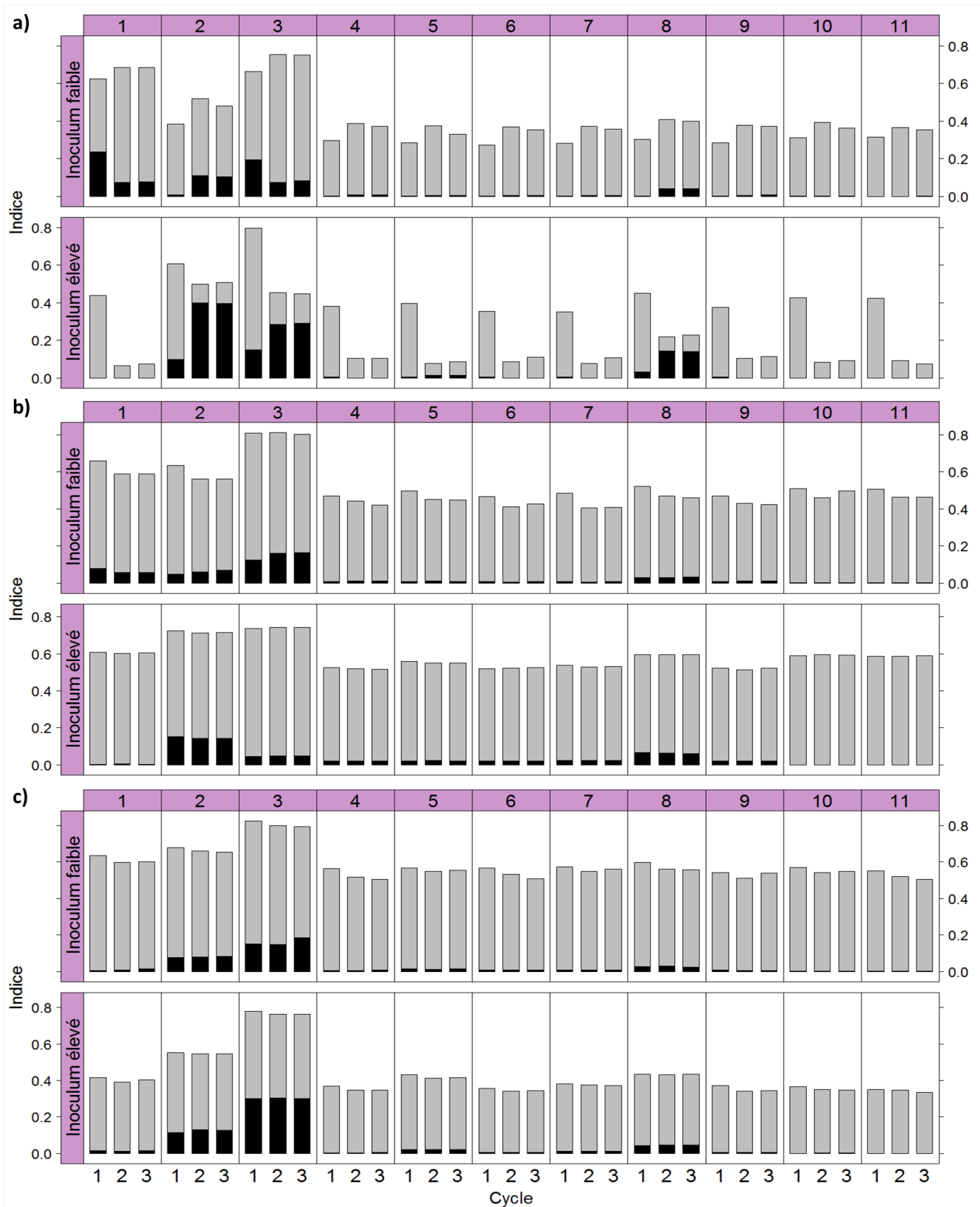
FIGURE A.21 – Indices de sensibilité principaux (en noir) et totaux (en gris + noir) des paramètres 11 paramètres du module épidémiologique calculés sur le rang de la PJFN de la plante à trois dates, a) initiation florale, b) floraison et c) 30 jours avant la récolte. Numérotation des paramètres : 1 : ei , 2 : ip , 3 : lgr , 4 : ei^{age} , 5 : a^{min} , 6 : sc_a , 7 : sc_s , 8 : \Delta_a , 9 : \Delta_s , 10 : \beta_a , 11 : \beta_s .
