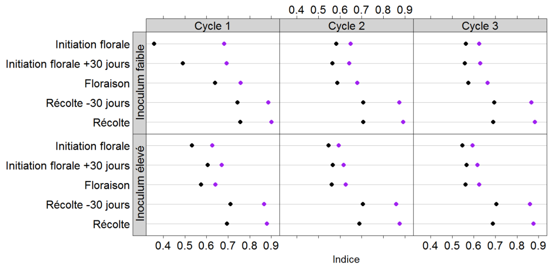
FIGURE 3.6 – Indices de sensibilité principaux (en noir) et totaux (en violet) du paramètres 3 : lgr du module épidémiologique calculés sur le pourcentage de maladie sur la plante à cinq temps selon deux doses d'inoculum.
