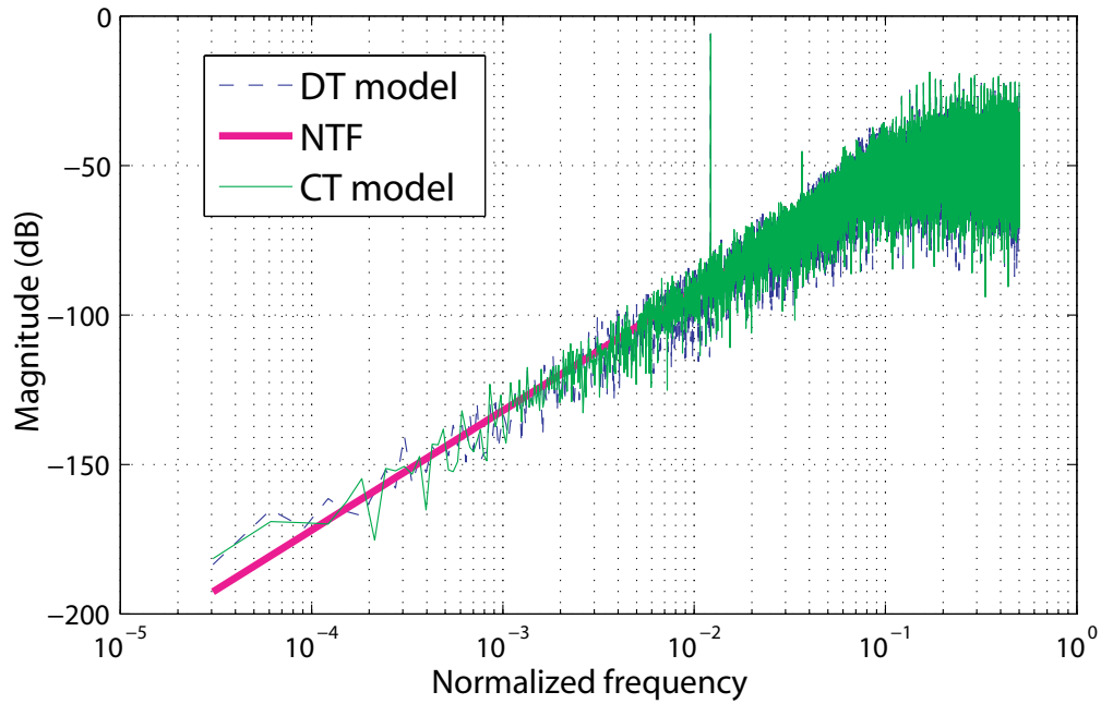
Figure 15: Entrée et sortie d'un modulateur \Sigma\Delta dans le domaine des fréquences
