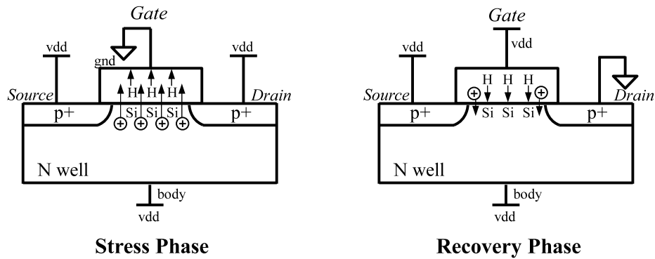
Figure 3: La phase de stress et de rétablissement du mécanisme NBTI.
