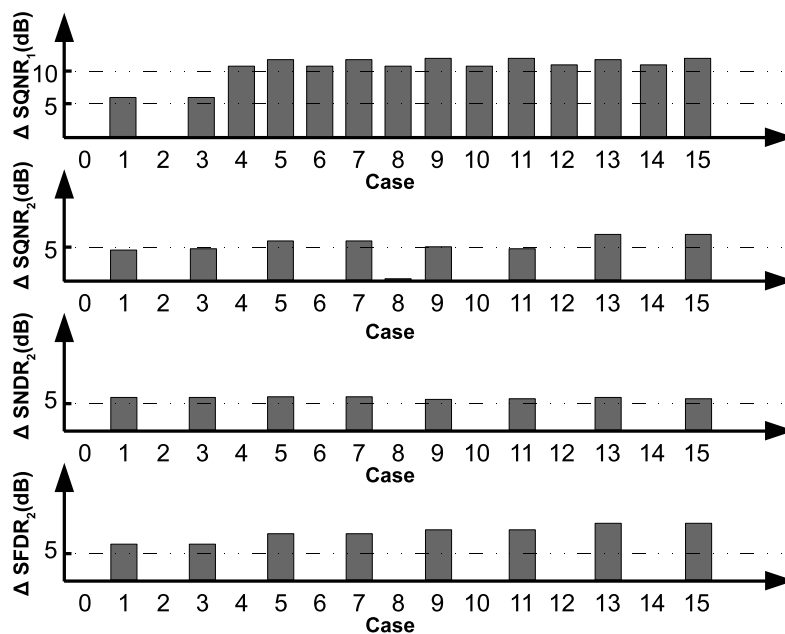
Figure 19: La dégradation de la performance versus le cas faillant du blocage par la barre graphique, SQNR 1 (cas minimum du design) et SQNR 2 , SNDR 2 , SFDR 2 (cas de sur-design). \Delta = X_0 - X_i est la paramètre de la performance, 'i' est l'index des cas.
