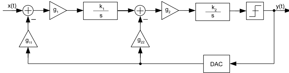
Figure 16: Le modèle du modulateur CT \Sigma\Delta de 2 ème ordre.
