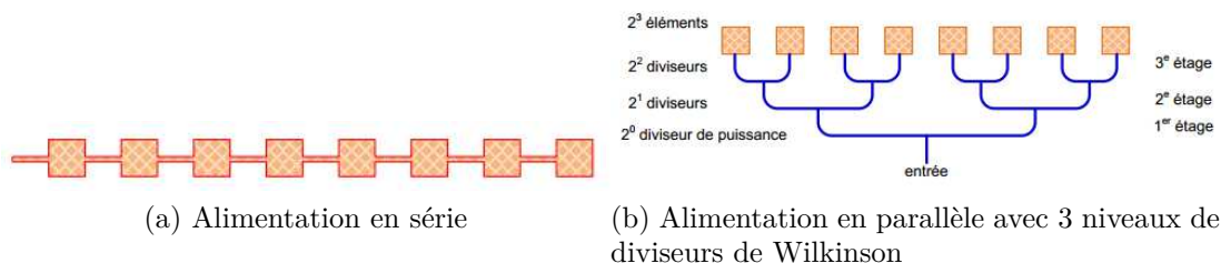
Figure 4.4 – Techniques d'alimentation [24].
