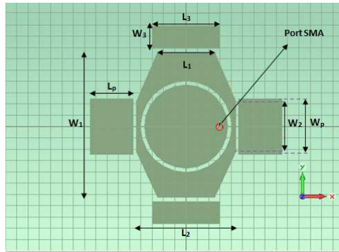
Figure 6.1 – Antenne avec quatre parasites.
