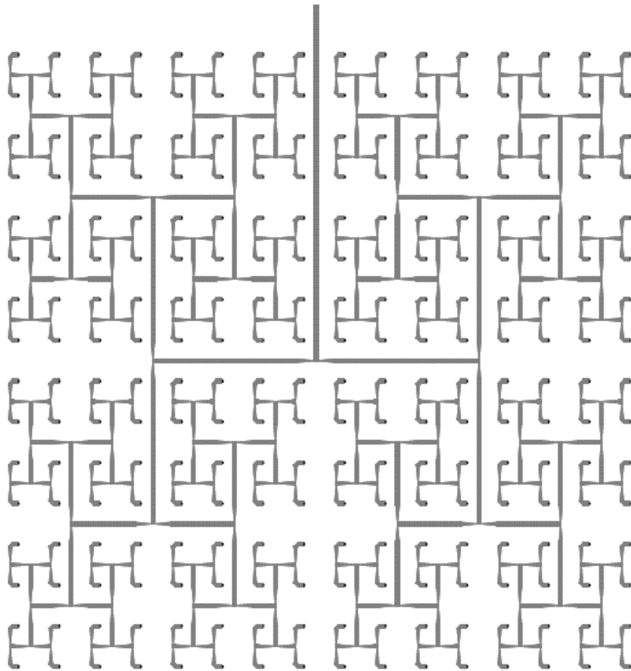
Figure 4.33 – Couche d'alimentation du réseau 16 \times 16 .
