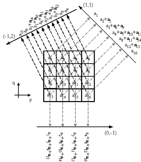
FIG. 3. – 4 \times 4 square Mojette transform with three projections. Transformation Mojette sur un carrée 4 \times 4 pour trois projections.
