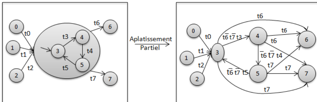
Figure IV.3 – Raccordement des états internes
