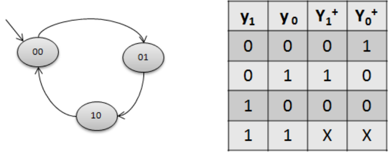
Figure IV.6 – Fonction d'état futur
