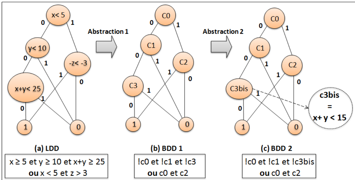
Figure III.7 – Présentation en LDD de F4
