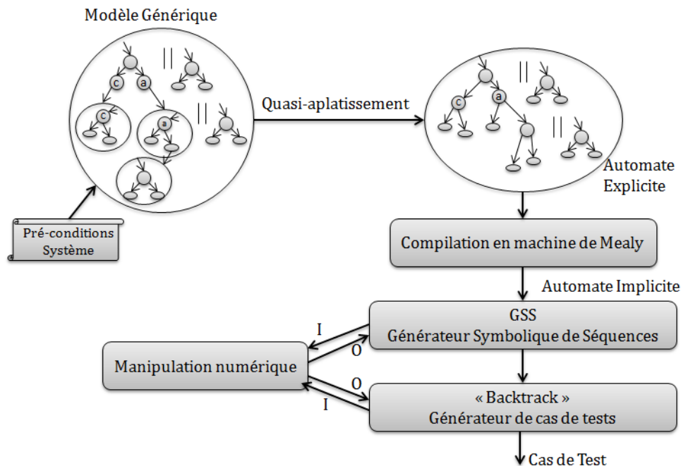
Figure IV.1 – Architecture globale du générateur de tests
