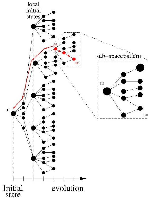
Figure IV.8 – Représentation GSS du modèle
