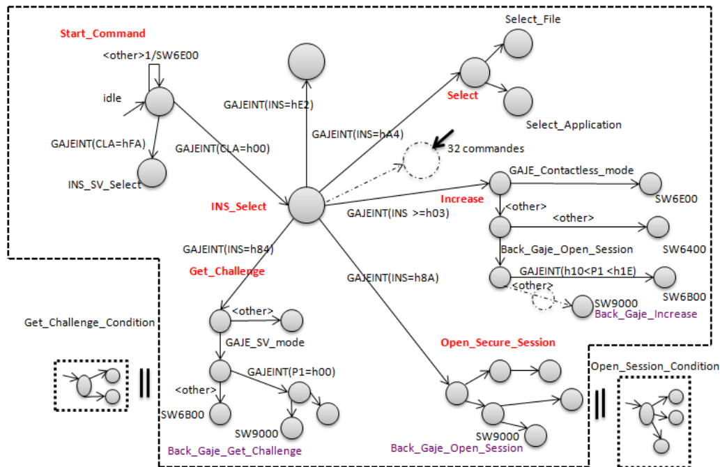
Figure V.7 – Modèle aplati de la carte à puce
