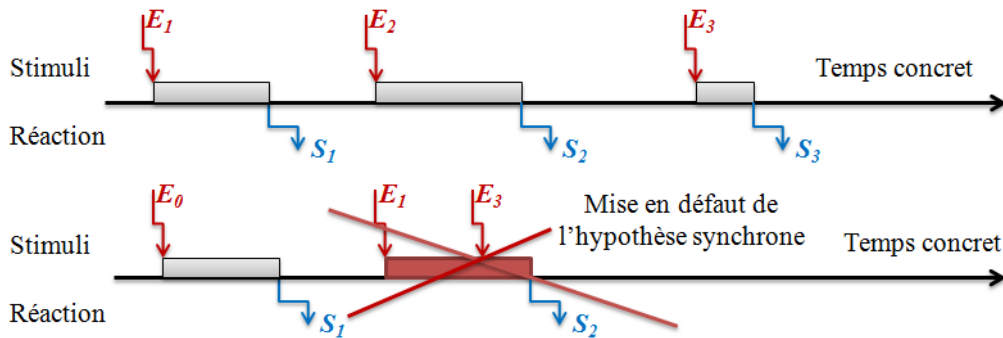
Figure II.4 – Vérification de l'hypothèse synchrone.
