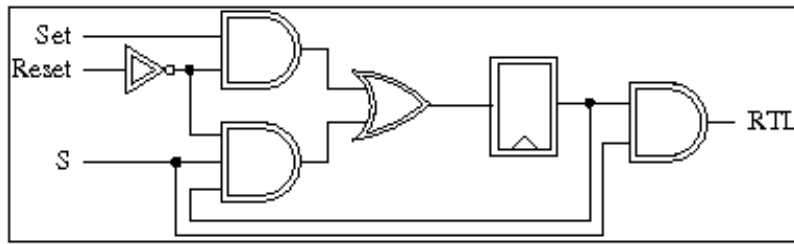
Figure II.9 – Réécriture de l'instruction "await" en Light Esterel.
