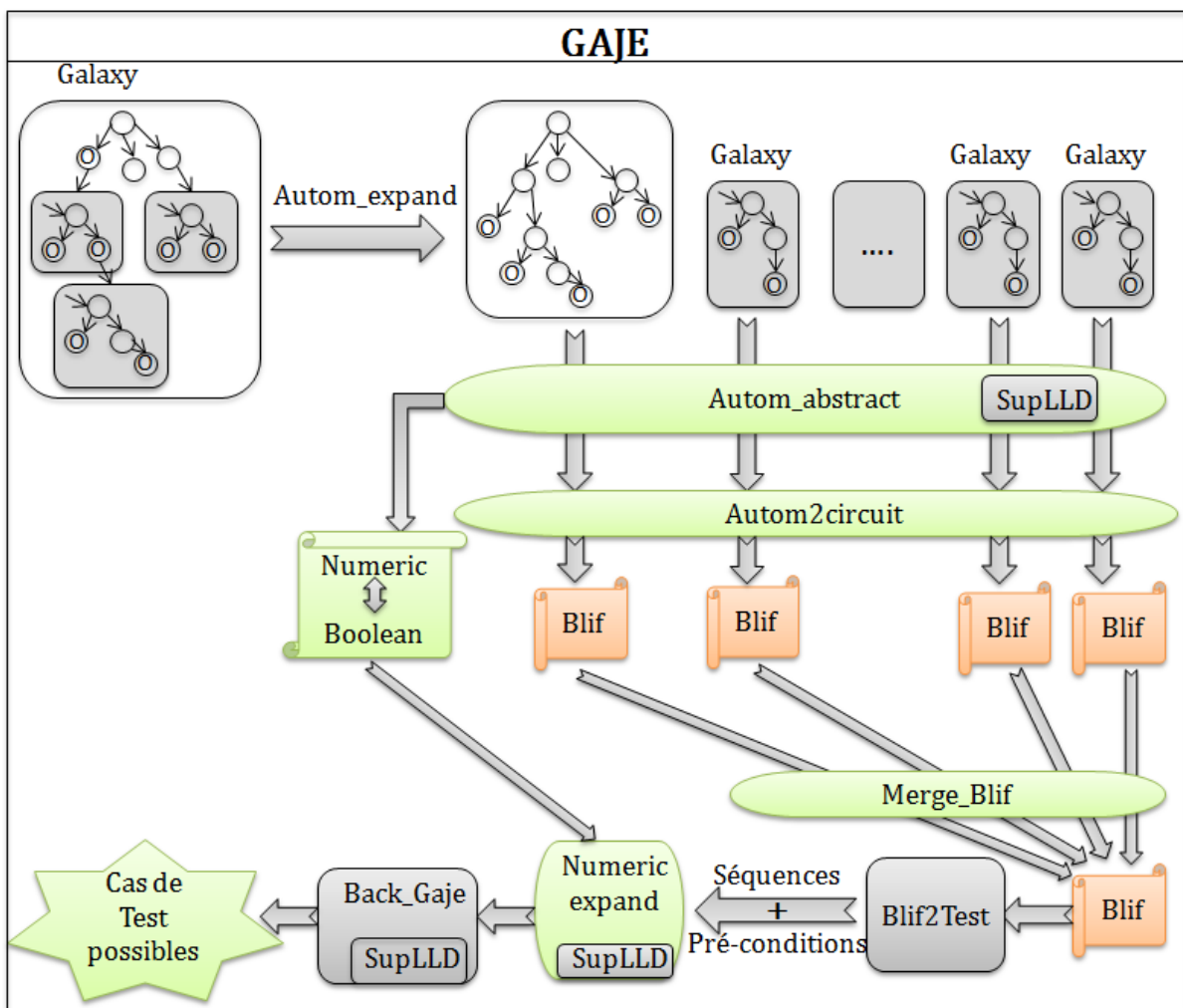
Figure V.1 – Chaîne des outils de la première version de GAJE
