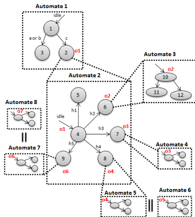
Figure IV.2 – Conception du modèle global
