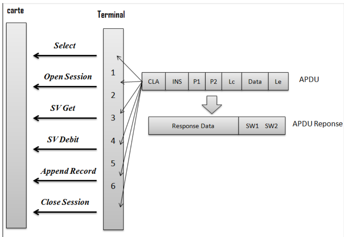
Figure V.3 – Exemple d'un scénario de la carte
