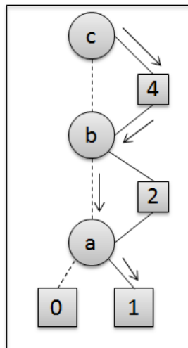
Figure III.4 – Présentation en EVBDD de F2
