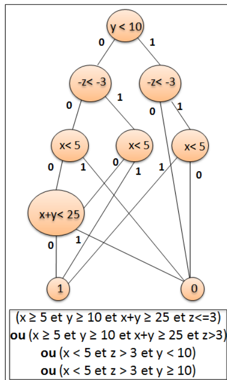
Figure III.8 – OLLD ordonné par \{y < 10\}; \{-z < -3\}; \{x < 5\}; \{x + y < 25\}
