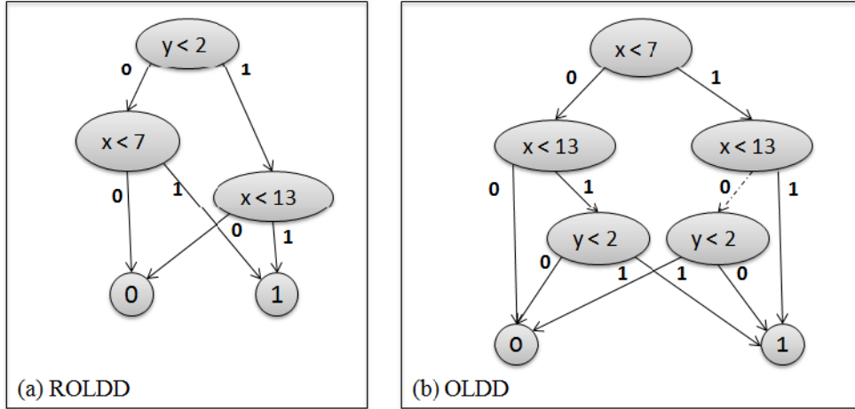
Figure III.12 – Ordonnement à niveaux des LDDs
