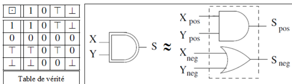
Figure II.5 – L'opérateur AND quadri-valué en Light Esterel.
