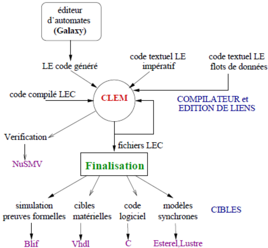
Figure II.12 – Chaîne de compilation Light Esterel .
