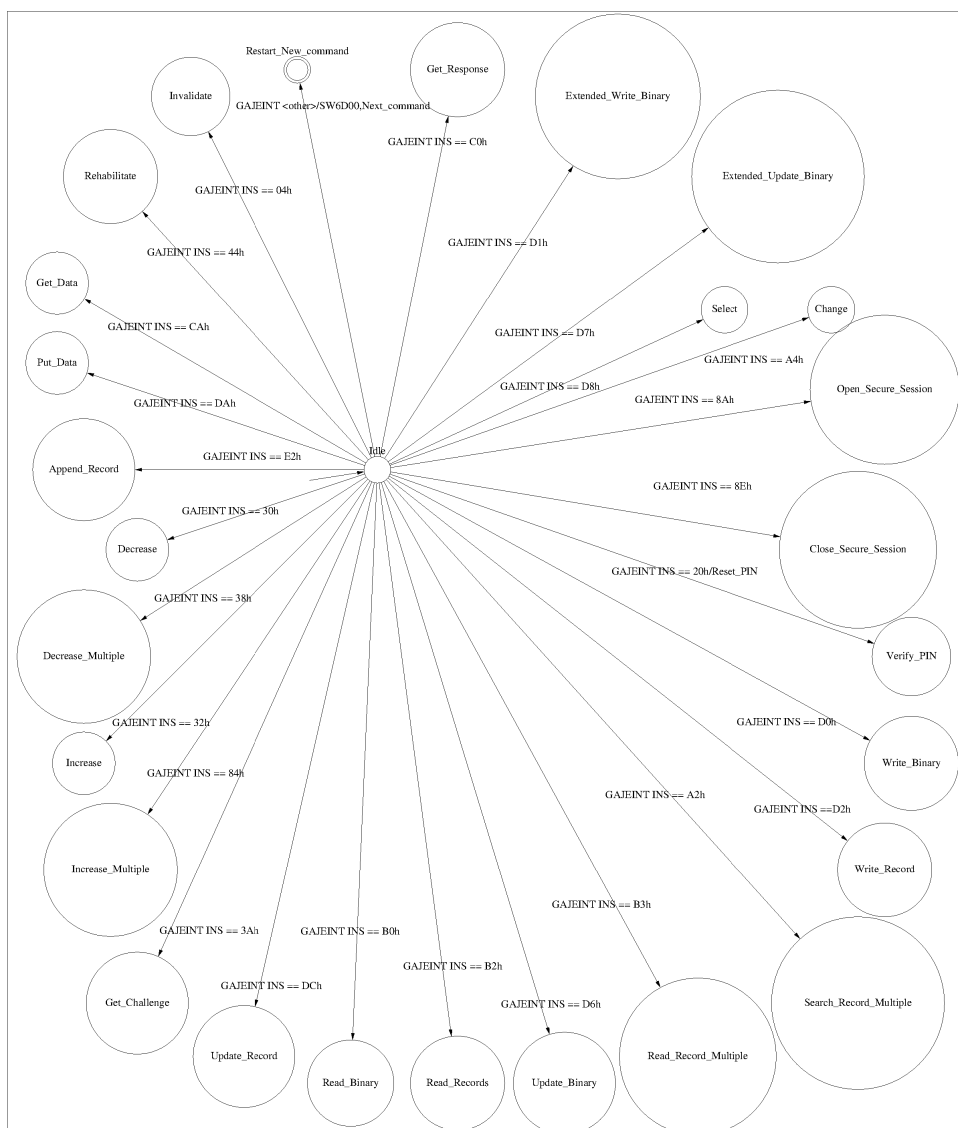
Figure V.6 – INS Command en galaxy
