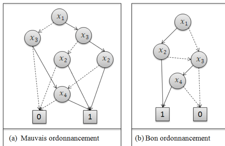
Figure III.2 – Présentation en BDD de f(x_1, \dots, x_4) = x_1x_2 + x_3x_4
