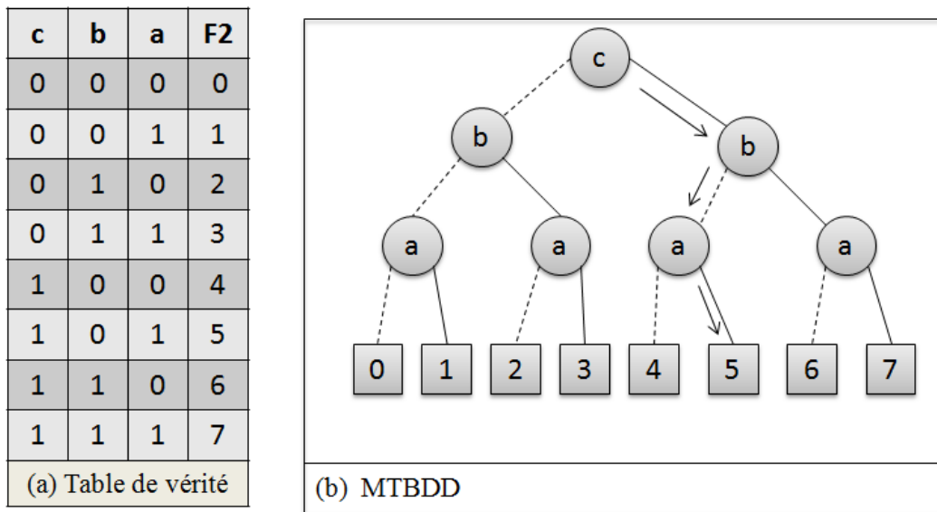
Figure III.3 – Présentation en MTBDD de F2
