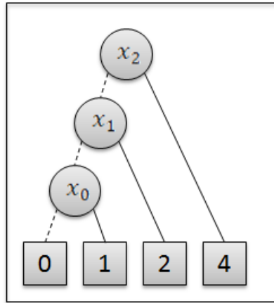
Figure III.5 – Présentation en BMD de F_2
