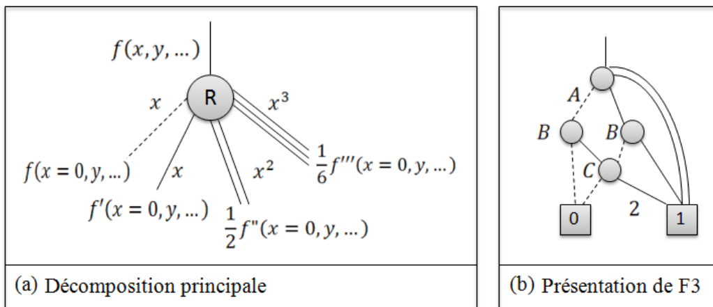
Figure III.6 – Présentation principale et en TED de F3
