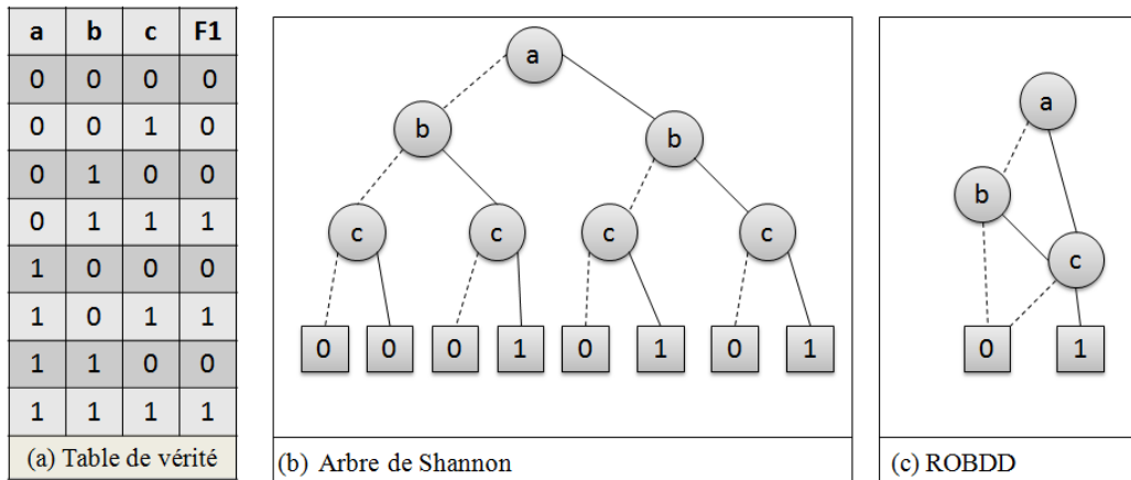
Figure III.1 – Présentation de F1 en BDD
