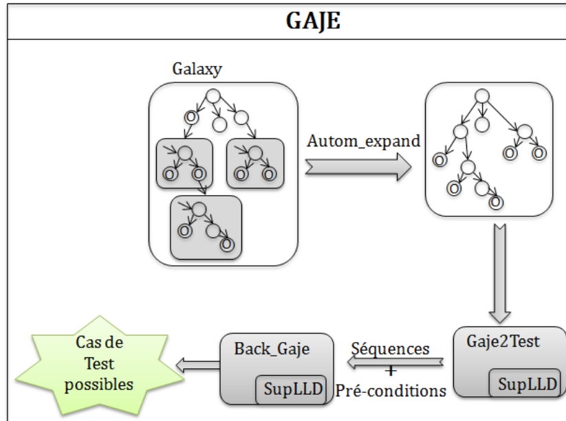
Figure V.2 – Chaîne des outils de la deuxième version de GAJE
