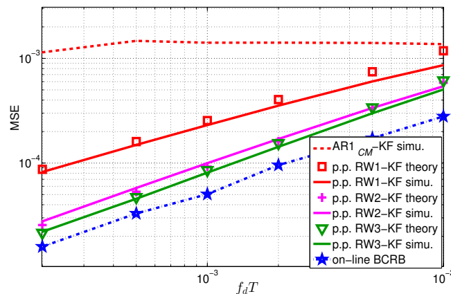
FIGURE 5.4 – MSE versus f_d T avec SNR = 20 dB, N_p = 16 , canal GSM
