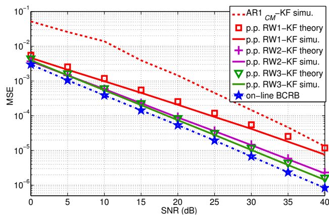
FIGURE 5.3 – MSE du per-path KF versus SNR avec f_d T = 10^{-3} , N_p = 16 , canal GSM
