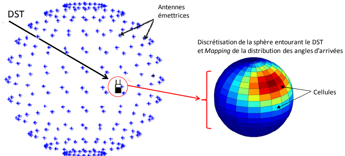
Figure II.2-11 : Principe de génération des angles d'arrivées
