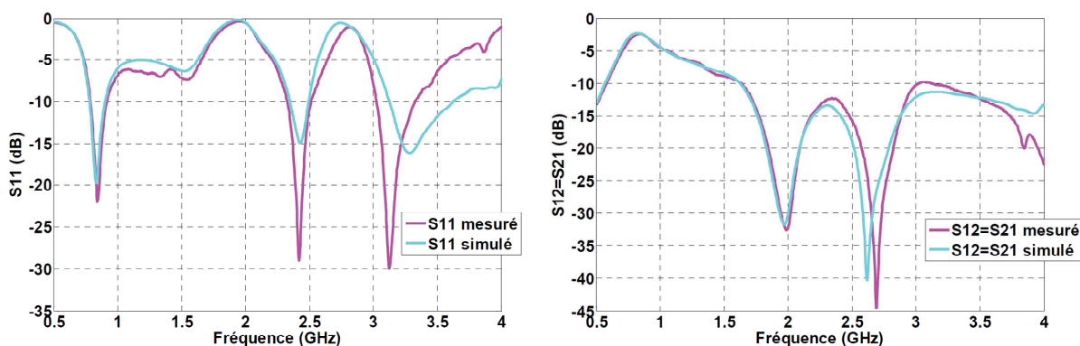
Figure II.1-11 : Coefficients de réflexion des prototypes réalisés
