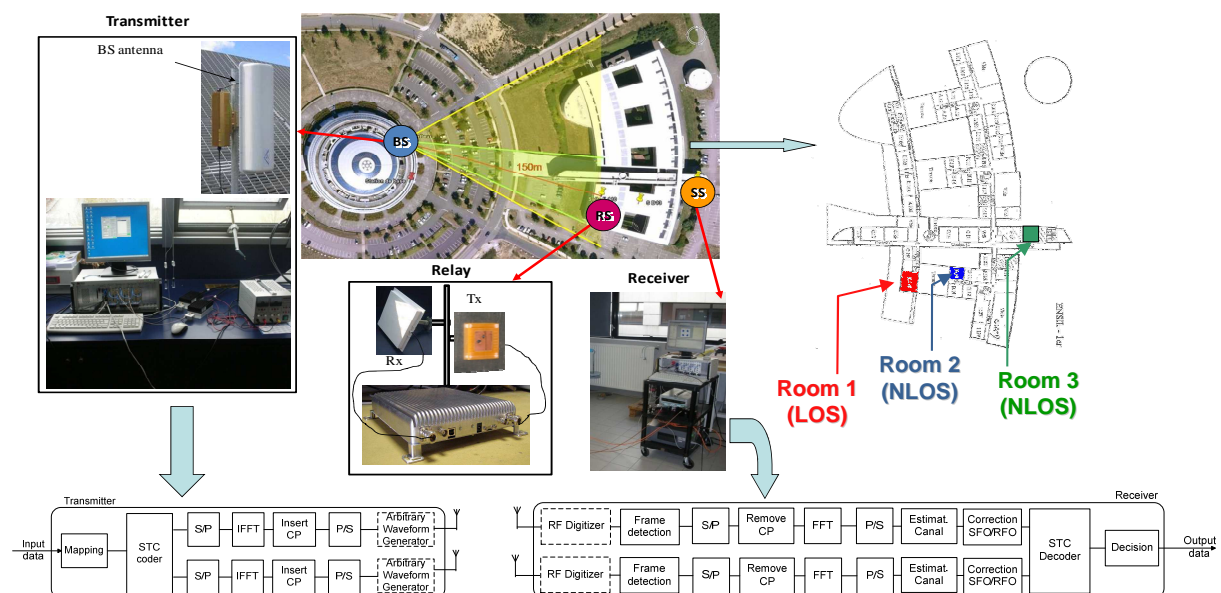
Figure II.4-2 : Démonstrateur expérimental de transmissions WiMax Outdoor to Indoor, utilisant un relais TDD.
