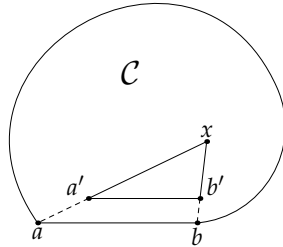
FIG. I.3 – Illustration de la contraposée de la propriété I.5.
