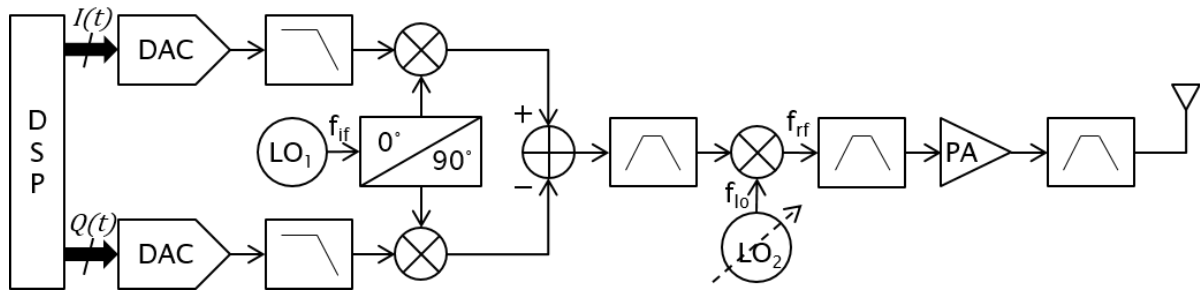
Figure II-1 : Émetteur hétérodyne
