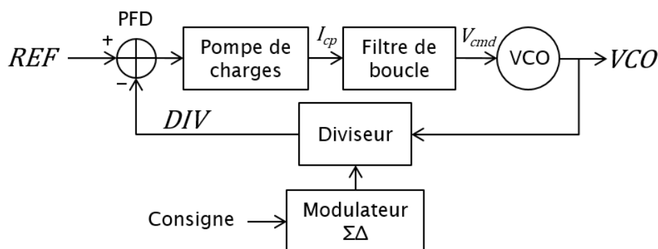
Figure III-1 : PLL analogique
