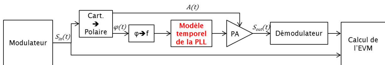
Figure IV-20 : Schéma de simulation
