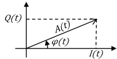
Figure II-4 : Équivalence cartésien/polaire
