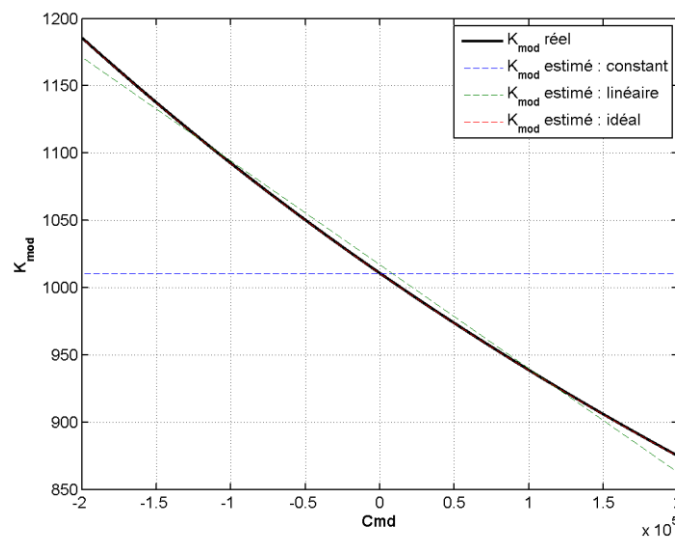
Figure V-5 : Méthodes d'estimation de la non-linéarité du gain de l'oscillateur
