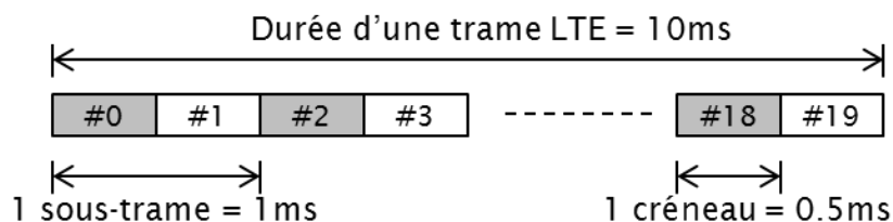
Figure I-12 : Trame de type 1
