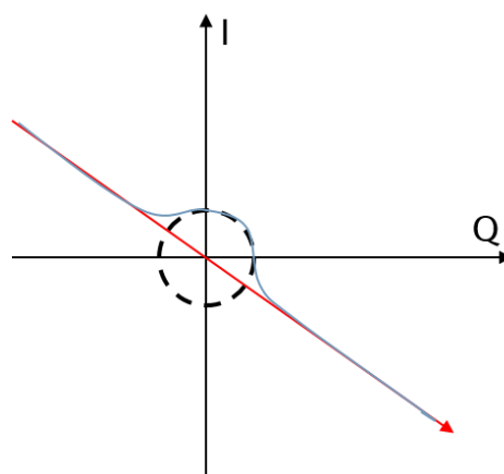
Figure III-36 : Principe du pré-processing
