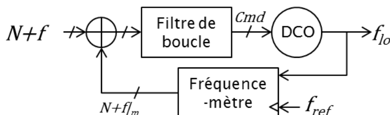
Figure IV-1 : PLL numérique
