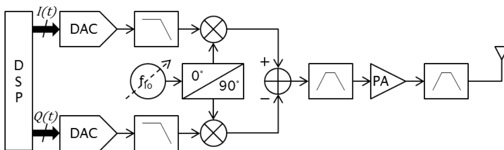
Figure II-2 : Émetteur homodyne
