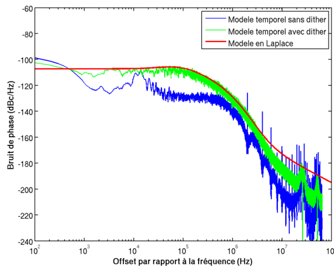
Figure IV-8 : Bruit de phase du TDC ramené en sortie de la PLL
