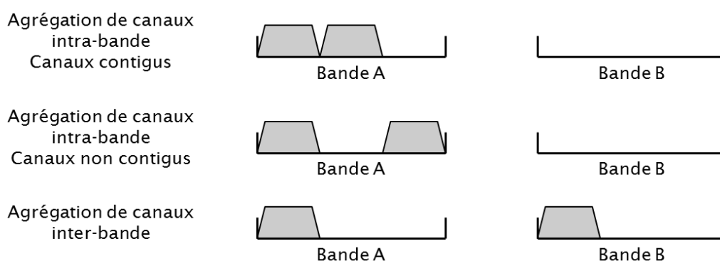
Figure I-14 : Types d'agrégation de canaux
