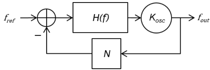
Figure II-11 : Schéma simplifié d'une PLL
