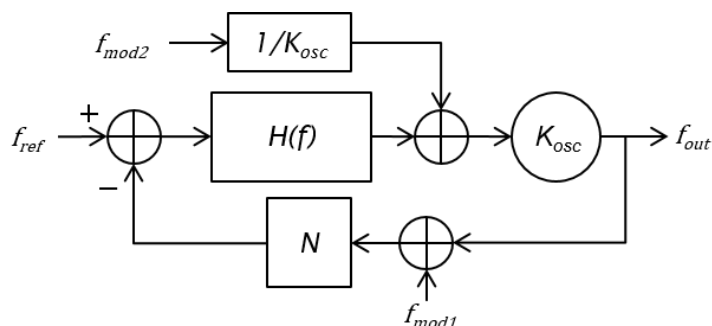
Figure II-14 : Insertion de la modulation en deux points
