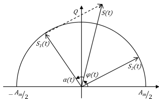
Figure II-10 : Construction du signal dans une architecture LINC
