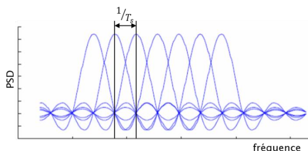
Figure I-6 : Sous-porteuses OFDM
