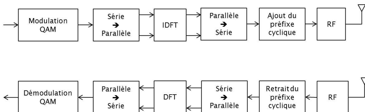
Figure I-7 : Modulateur/Démodulateur OFDM
