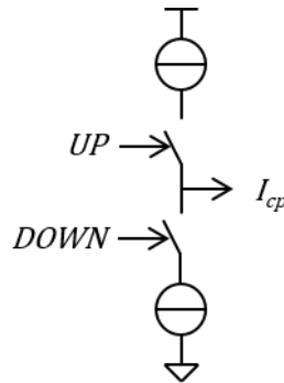
Figure III-6 : Schéma de principe d'une pompe de charges
