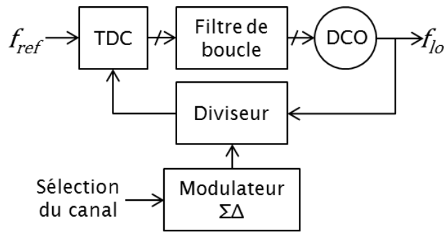
Figure II-24 : PLL numérique fractionnaire
