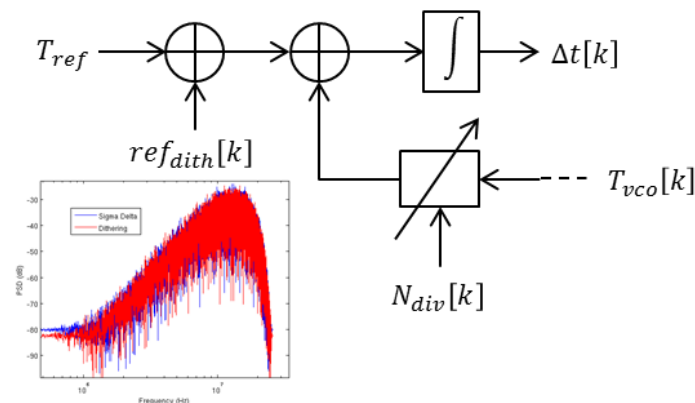
Figure III-27 : Ajout du « dither » sur la référence
