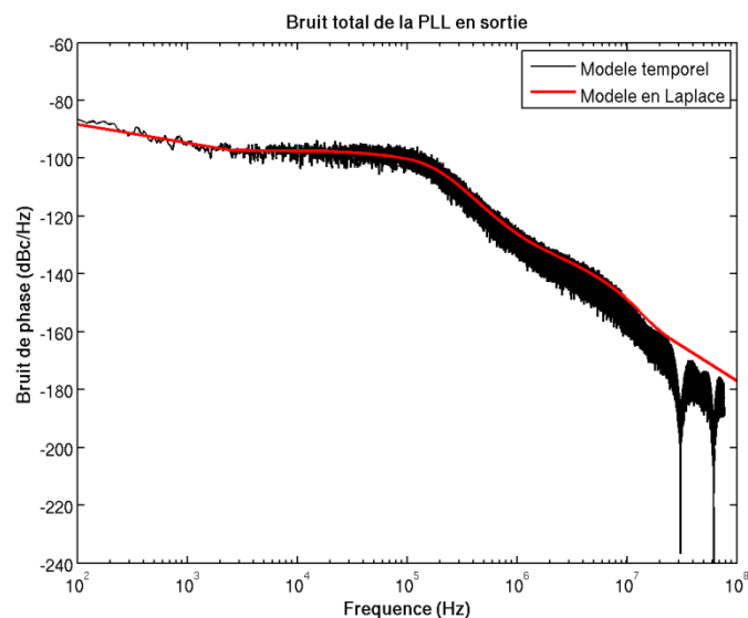
Figure III-18 : Bruit de phase total de la PLL
