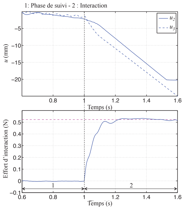
FIGURE 4.17 – Déplacements u_2 et u_3 (haut) et effort d'interaction (bas). L'effort mesuré est en bleu tandis que la ligne magenta représente l'effort d'interaction théorique pour la configuration du prototype imposée par la position de l'environnement.
