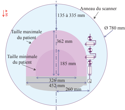
FIGURE 4.8 – Mise en évidence des dimensions (Scanner vu de face).
