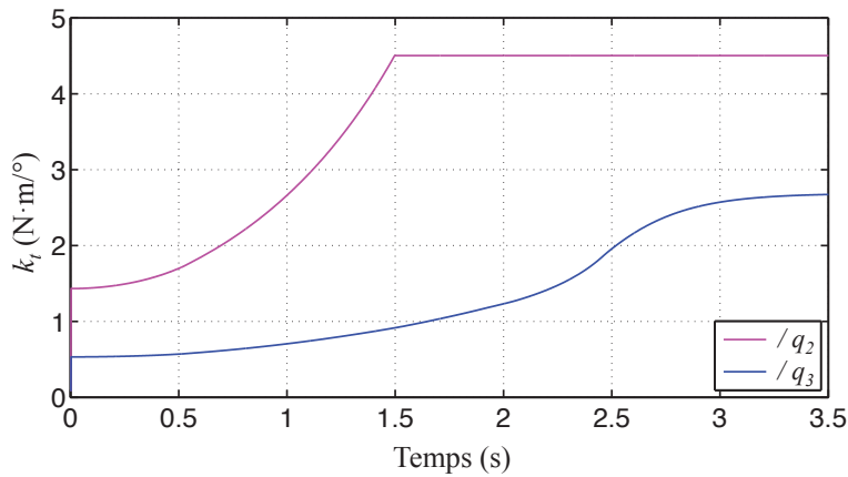
FIGURE 4.24 – Raideurs aux articulations q_2 et q_3 lors du suivi de trajectoire.
